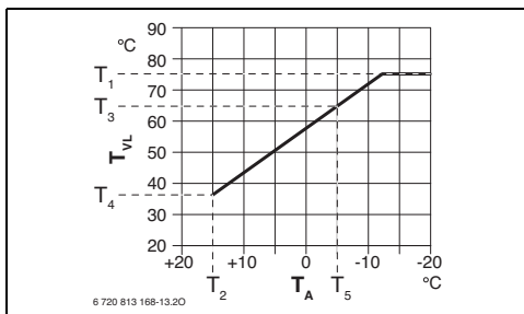
Fig. 14 Diagrama de calefacción para radiadores convencionales
