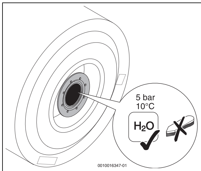
Fig. 65 Rocíe el acumulador
