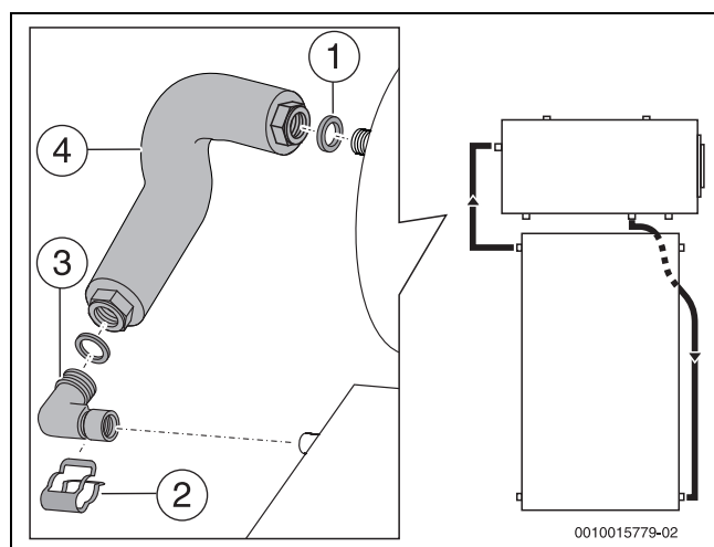
Fig. 48 Montaje de la tubería de alimentación
