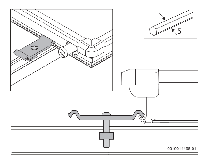
Fig. 41 Sólo colocar el tensor bilateral del colector
