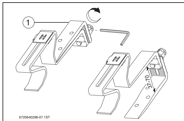
Fig. 18 Girar la parte inferior de los ganchos de tejado, dimensiones en mm
