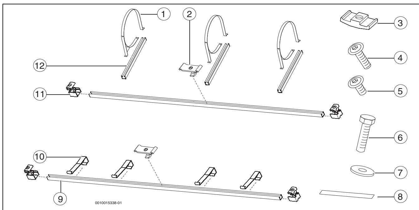
Fig. 2 Juego de montaje (TSS300)
