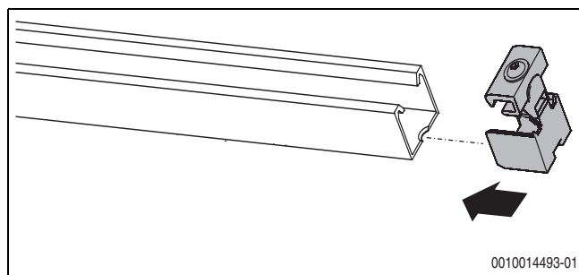
Fig. 38 Montaje del tensor del colector a la derecha
