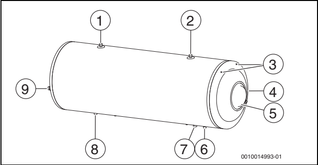
Fig. 5 Acumulador para sistema termosifón
