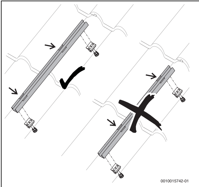
Fig. 28 Posicionar correctamente los perfiles guía para el acumulador
