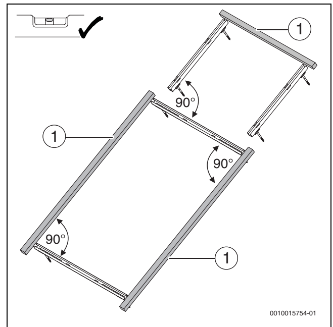
Fig. 30 Alinear los perfiles guía de una manera exacta
