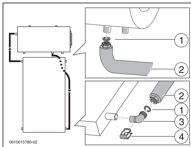
Fig. 49 Montaje de la tubería de retorno
