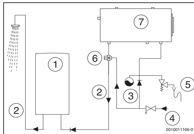
Fig. 52 Ejemplo de instalaciones sin módulo solar
