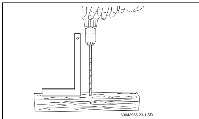
Fig. 15 Elaborar una plantilla para taladrar
