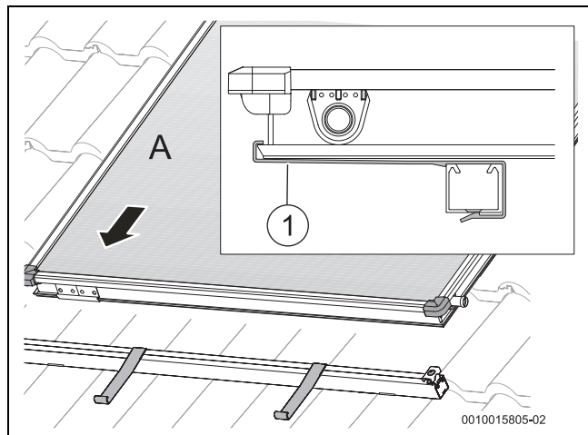
Fig. 39 Deje deslizar el colector hasta los seguros contra deslizamiento
