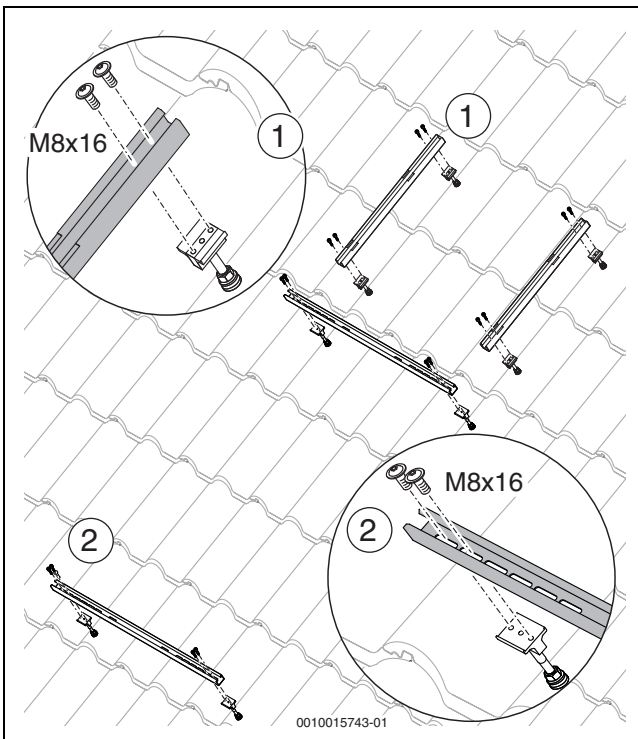
Fig. 29 Montar los perfiles guía abajo y arriba
