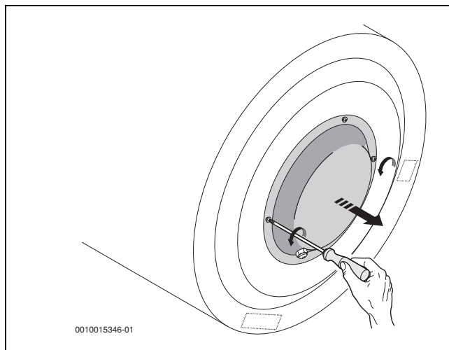
Fig. 63 Retirar la tapa del acumulador
