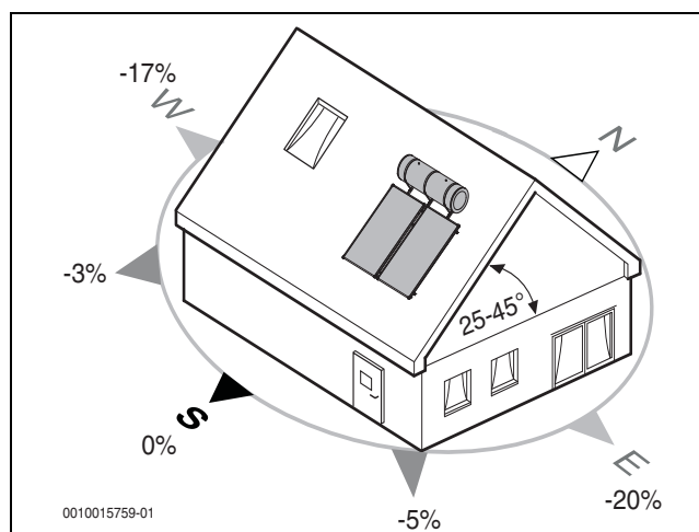
Fig. 8 Pérdidas de rendimientos solares en diferencias por % (Atenas)
