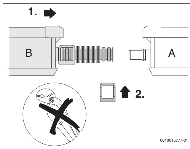
Fig. 42 Colocar el colector izquierdo junto al colector derecho
