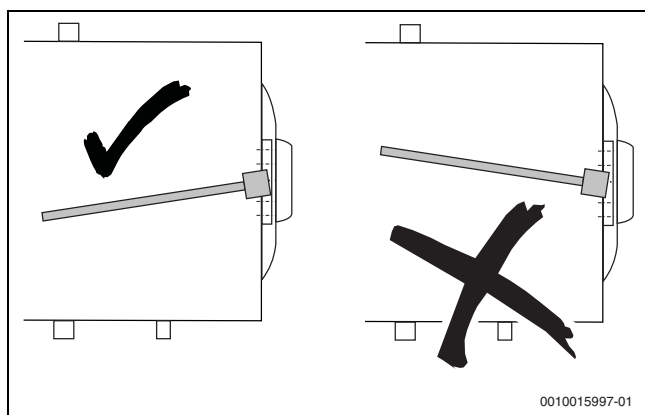
Fig. 66 Resistencia eléctrica indicando hacia abajo
