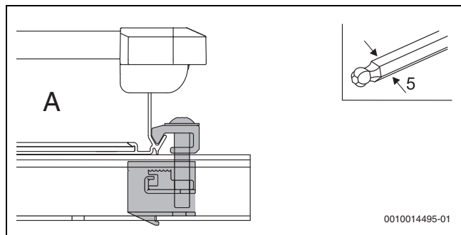
Fig. 40 Apretar el tornillo del tensor del colector
