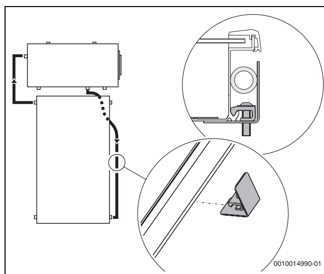
Fig. 50 Montar el soporte en el borde del colector
