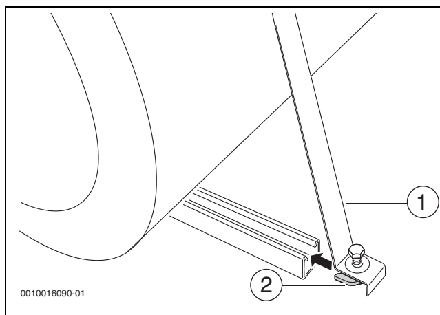
Fig. 35 Atornillar la abrazadera del acumulador
