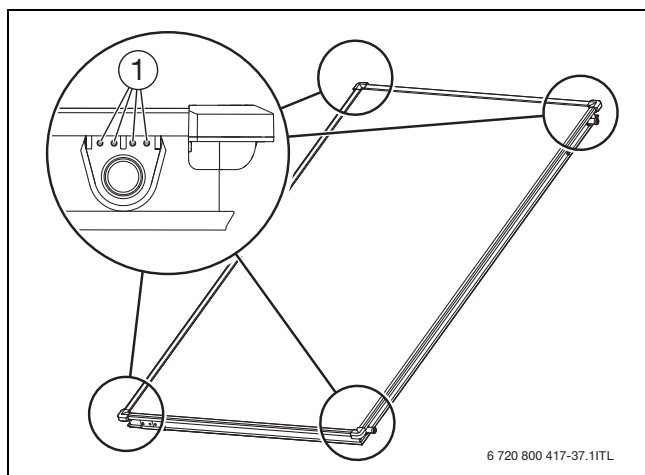
Fig. 59 Aberturas de ventilación
