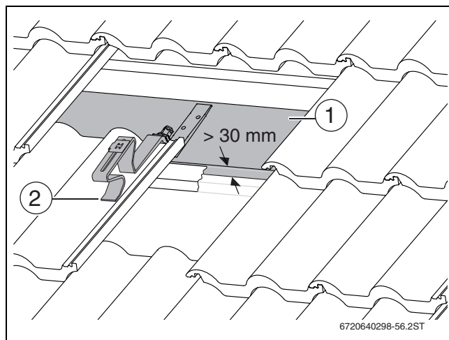
Fig. 23 Montar el anclaje en la tabla/el madero
