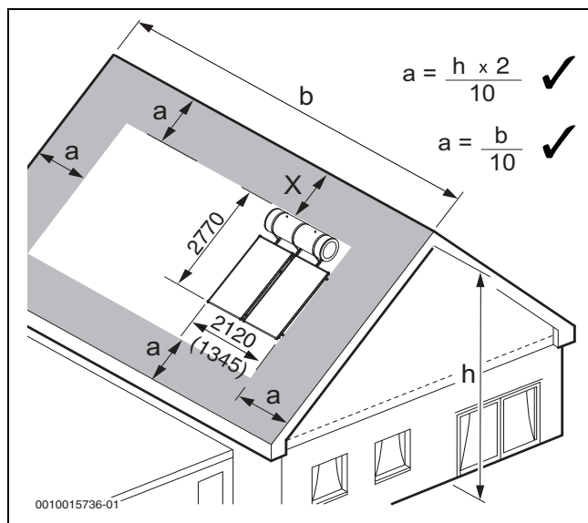
Fig. 9 Dimensiones (valor en paréntesis: sistema con 1 colector)
