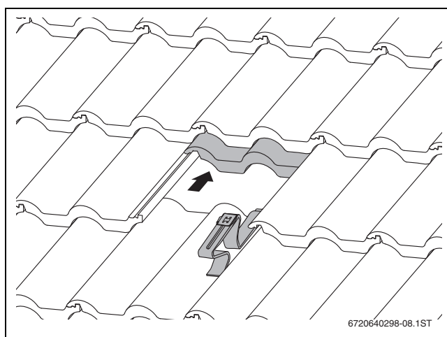
Fig. 19 Gancho de tejado colgado
