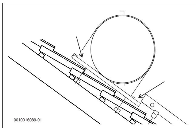
Fig. 55 Posible conexión del dispositivo pararrayos a los perfiles guía del acumulador
