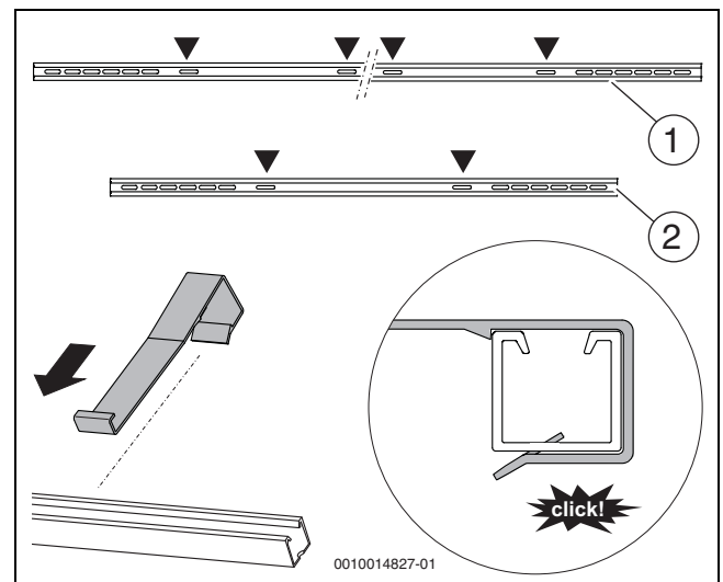
Fig. 31 Montar los seguros antideslizamiento al perfil guía inferior
