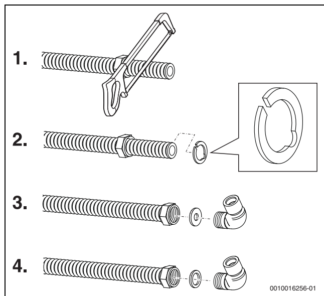
Fig. 47 Acortar el tubo de conexión; representación sin aislamiento
