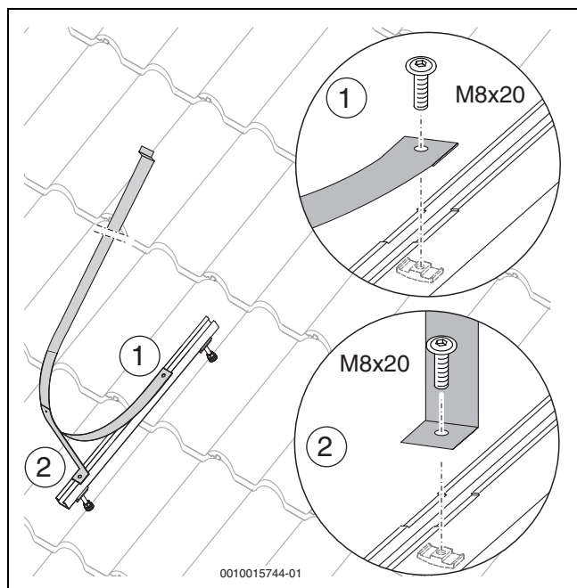
Fig. 32 Montar la abrazadera del acumulador
