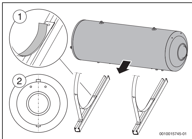
Fig. 33 Colocar el acumulador en la abrazadera del acumulador y alinearlo
