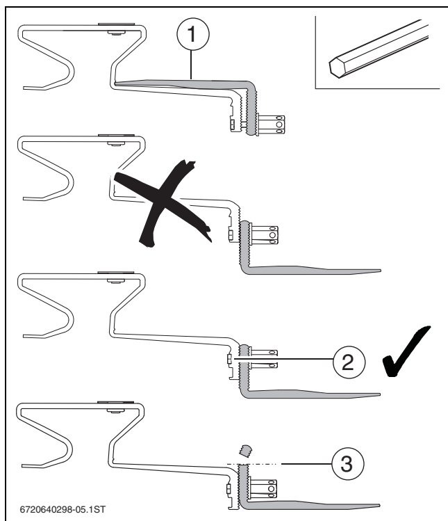
Fig. 22 Preparar el anclaje
