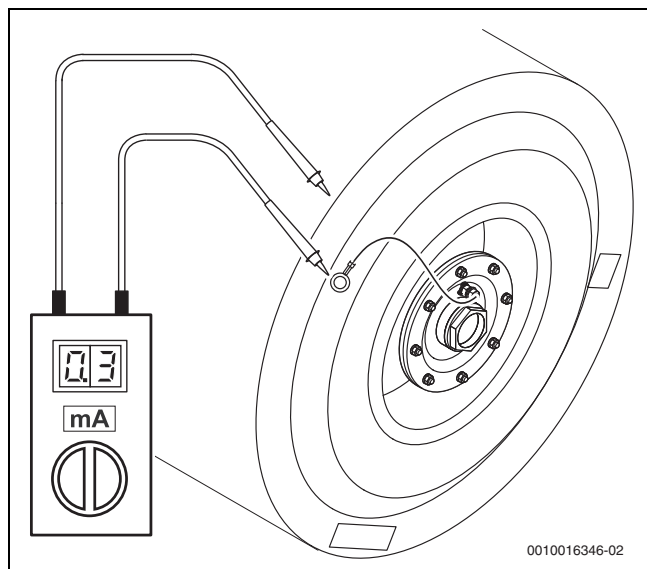
Fig. 62 Comprobar el funcionamiento eléctrico del ánodo
