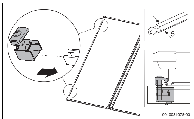
Fig. 45 Montar la sujeción del colector en el lado izquierdo
