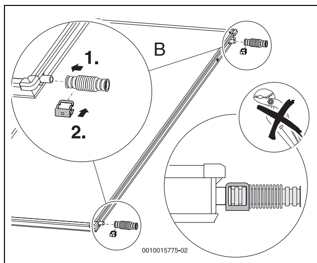
Fig. 37 Montar el set de conexión hidráulica en el colector izquierdo
