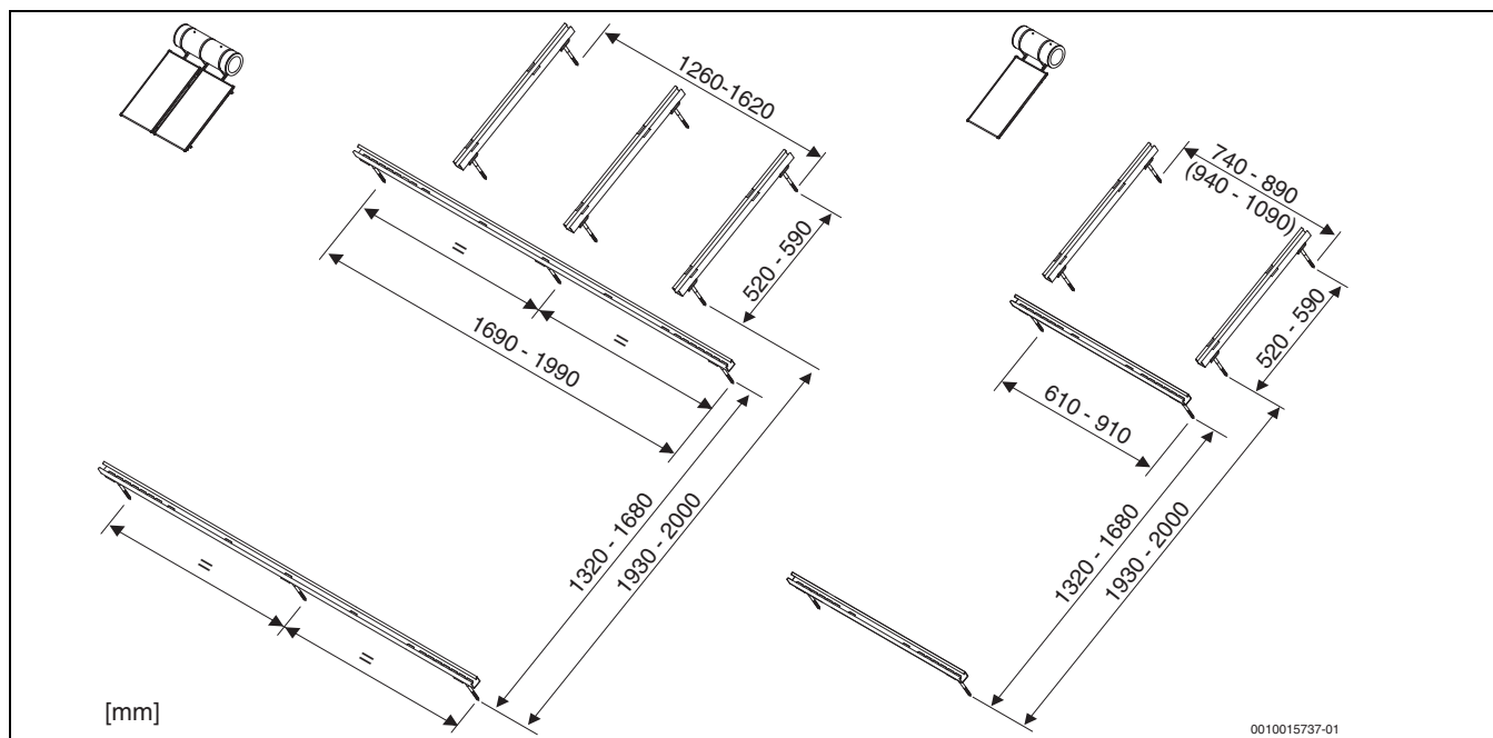
Fig. 14 Distancias tornillos de doble rosca en: TSS300 (izquierda) y TSS150/200 (derecha), el valor en paréntesis vale para TSS200
