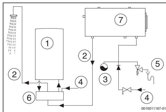
Fig. 53 Ejemplo de instalaciones con módulo solar
