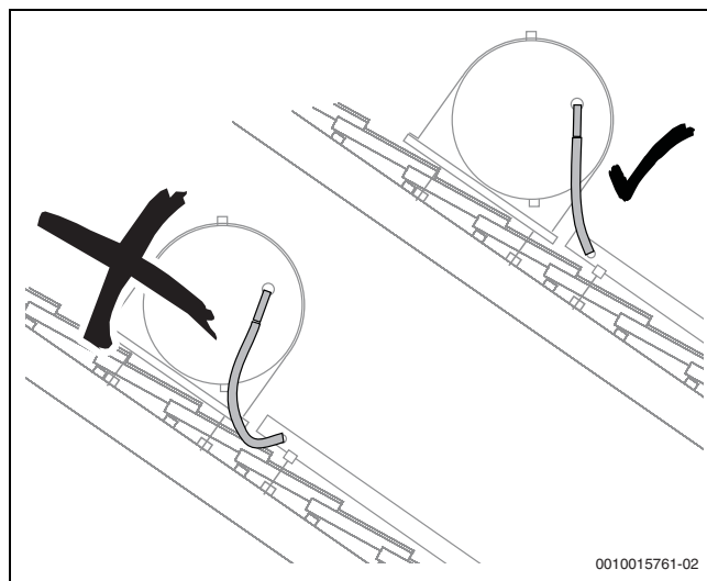
Fig. 46 No colocar una comba de la tubería (aquí: tubería de alimentación)
