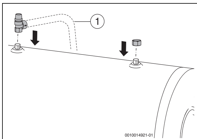
Fig. 57 Montar la válvula de seguridad y la tapa
