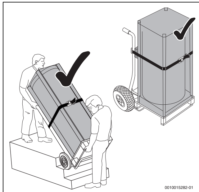
Fig. 13 Transportar el acumulador con la carretilla
