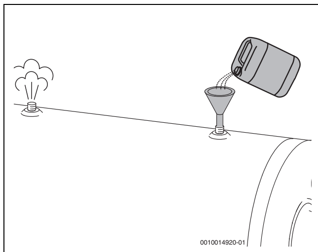
Fig. 56 Llenar líquido solar
