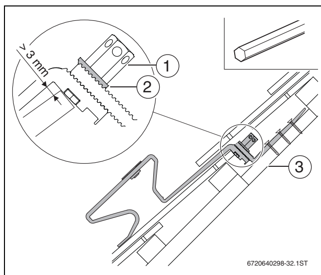
Fig. 25 Montar el anclaje
