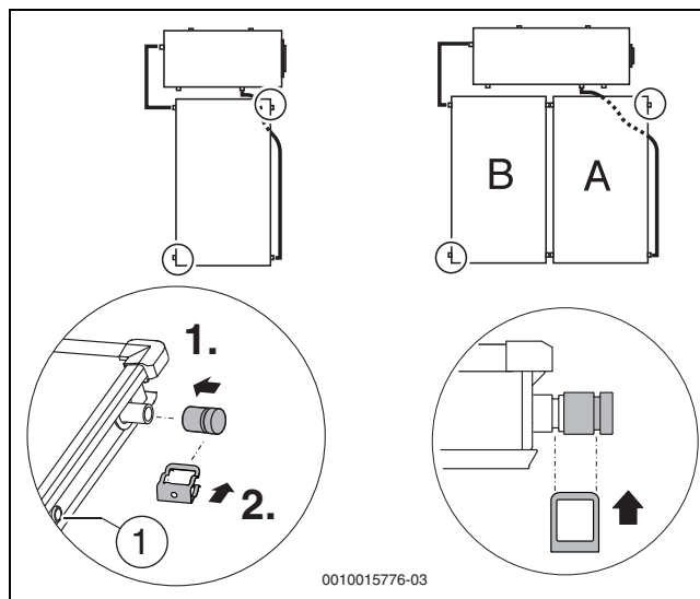
Fig. 36 Montar los tapones de cierre
