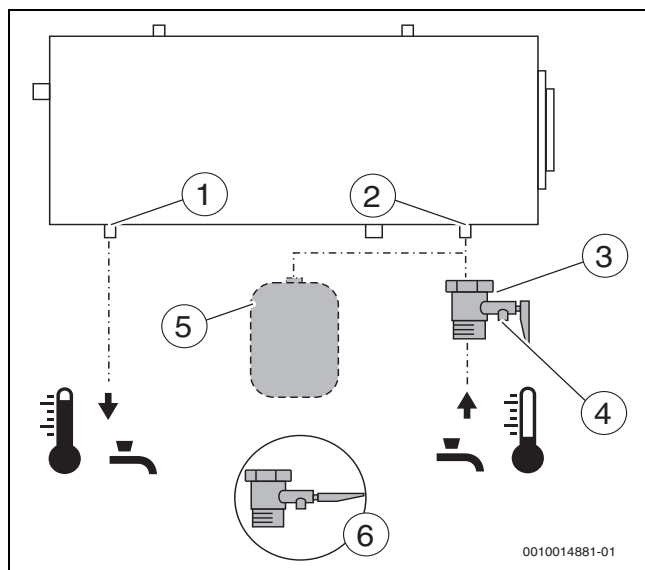
Fig. 51 Conexión de las tuberías de agua sanitaria
