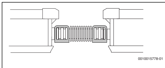
Fig. 51 Unión de tubo ondulado montado
