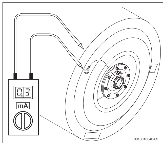
Fig. 81 Comprobar el funcionamiento eléctrico del ánodo
