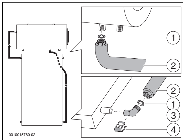
Fig. 68 Montaje de la tubería de retorno
