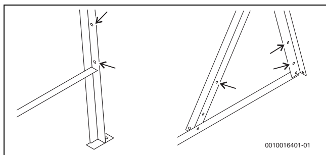
Fig. 74 Ejemplos de montaje del cable de puesta en tierra en el soporte de montaje (izquierda MTSS, derecha: WSF)
