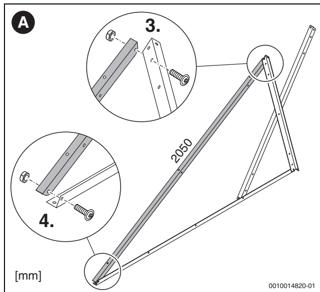
Fig. 22 Montar perfil 2050 mm
