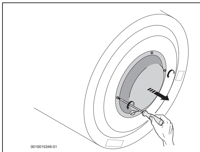
Fig. 80 Retirar la tapa del acumulador
