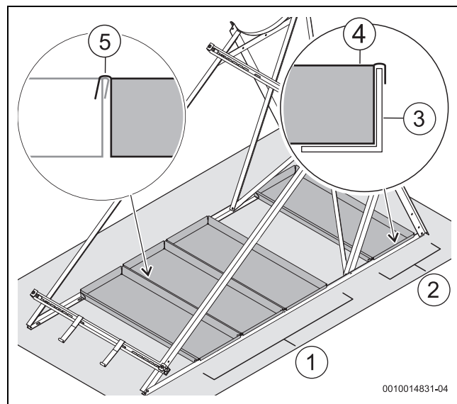
Fig. 33 Colocar las bandejas de carga
