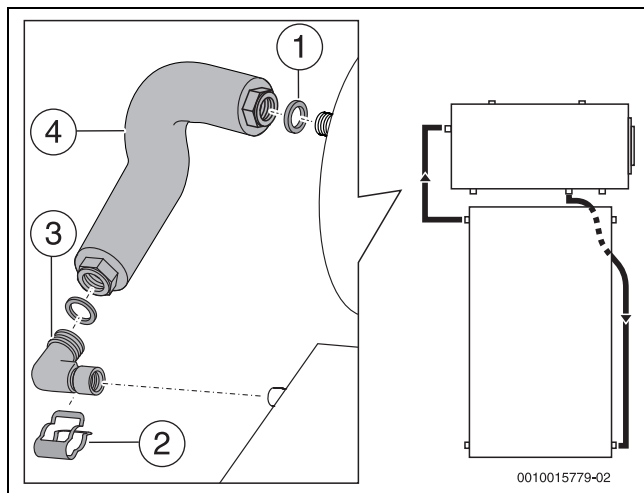
Fig. 67 Montaje de la tubería de alimentación (sistema TSS200)
