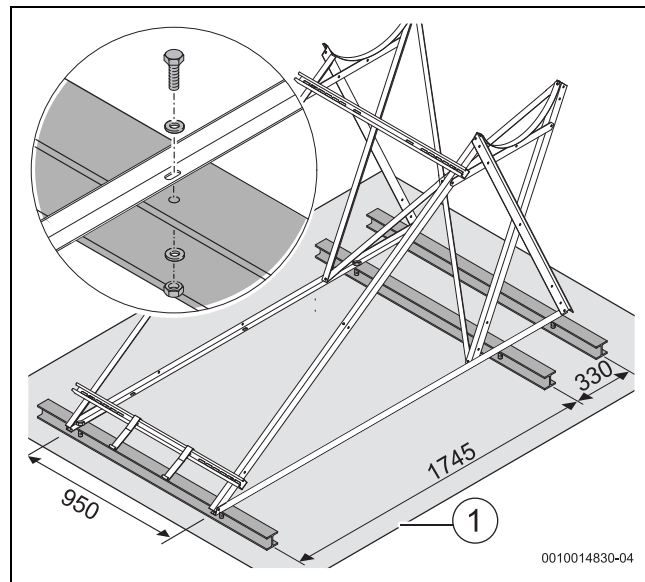
Fig. 32 Ejemplo TSS150/200: montar perfiles angulares en vigas en doble T (ejemplo TSS300 → fig. 34)
