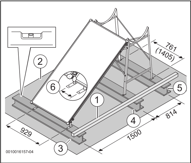
Fig. 58 Ejemplo TSS150/200: montaje sobre soportes de doble T (valor en paréntesis: 2 colectores TSS300)
