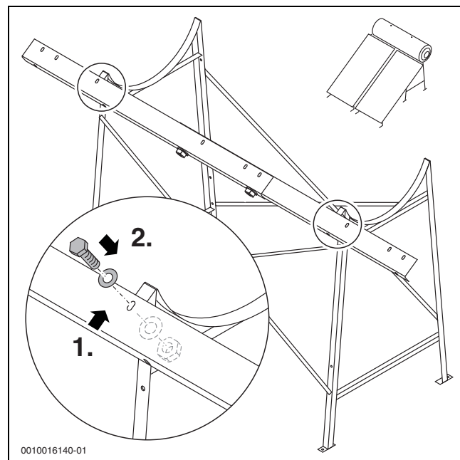
Fig. 39 Fijar los perfiles angulares unidos en el soporte de montaje
