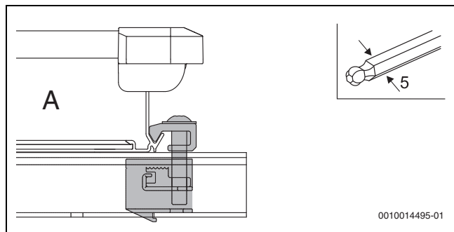
Fig. 47 Apretar el tornillo del tensor del colector
