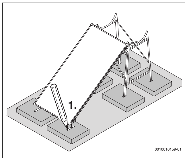
Fig. 60 Ejemplo: montaje en placas de concreto, marcar los orificios de taladrado
