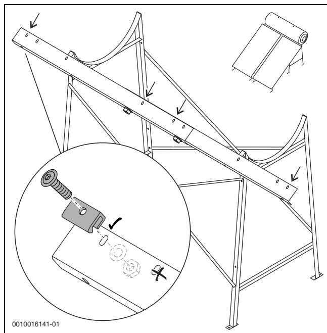
Fig. 41 MTSS2: Atornillar el pisador en los perfiles angulares
