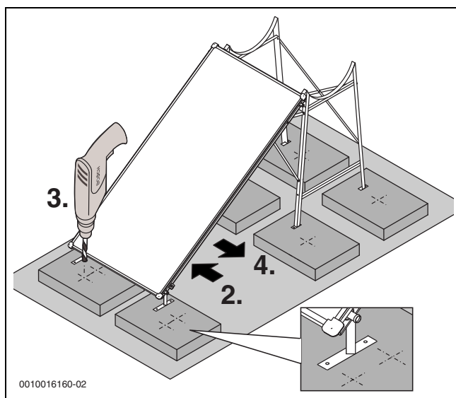
Fig. 61 Ejemplo: montaje en placas de concreto
