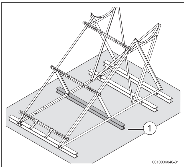
Fig. 31 Ejemplo: Unión del techo con soporte de doble T
