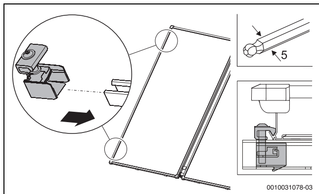
Fig. 52 Montar la sujeción del colector en el lado izquierdo
