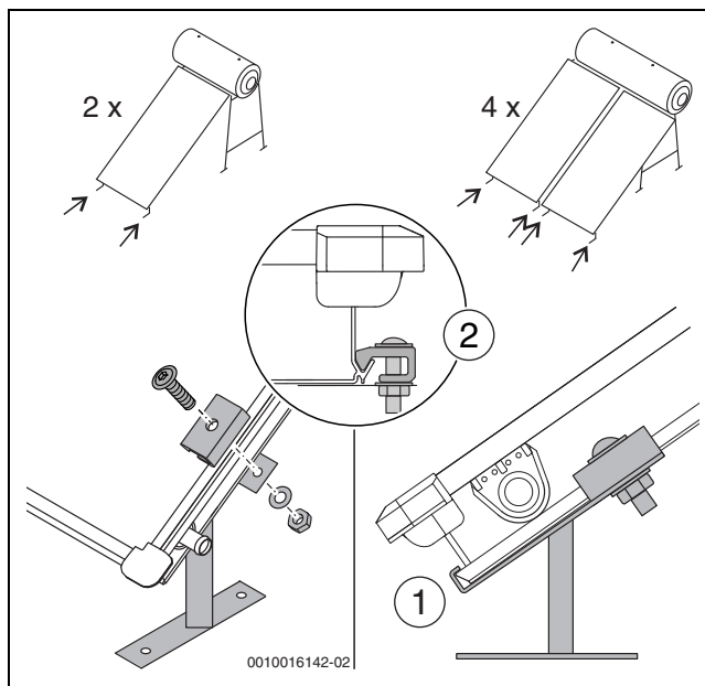
Fig. 42 Montar el soporte de pie
