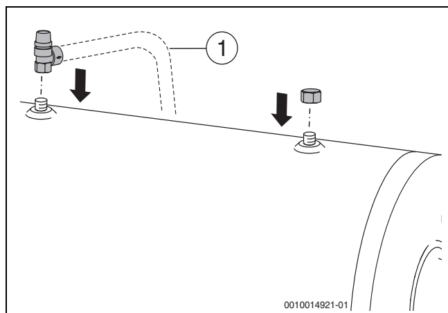
Fig. 76 Montar la válvula de seguridad y la tapa
