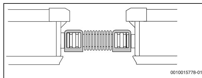
Fig. 56 Unión de tubo ondulado montado
