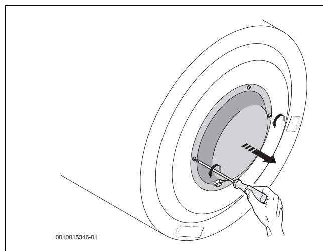
Fig. 82 Retirar la tapa del acumulador
