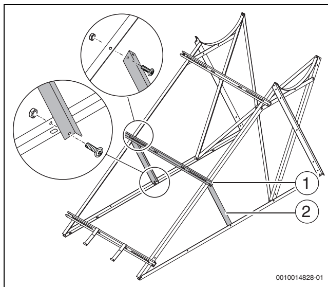
Fig. 30 Montar los accesorios para cargas elevadas
