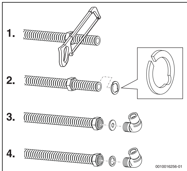
Fig. 66 Acortar el tubo ondulado; representación sin aislamiento
