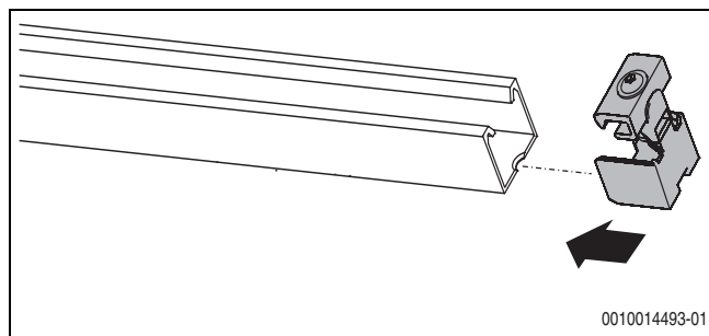
Fig. 45 Montaje del tensor del colector a la derecha
