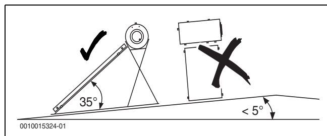
Fig. 9 Tener en cuenta el posicionamiento y la inclinación de tejado permitida
