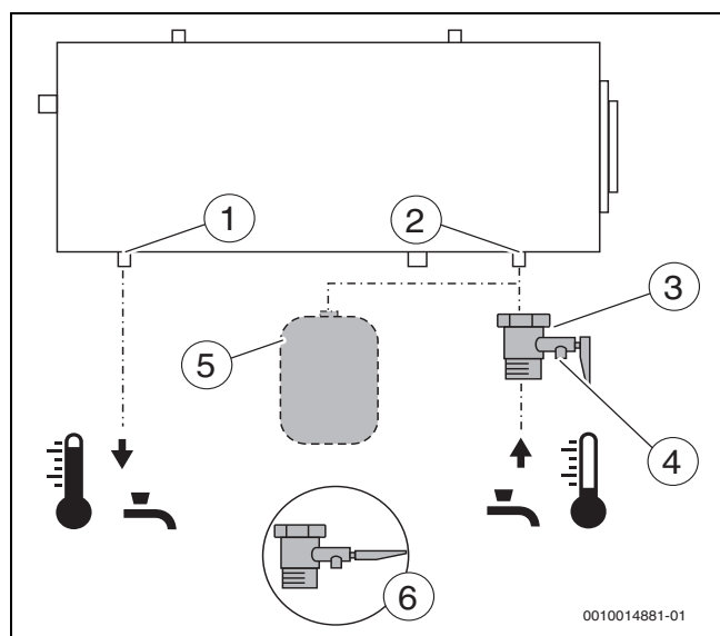
Fig. 70 Conexión de las tuberías de agua sanitaria
