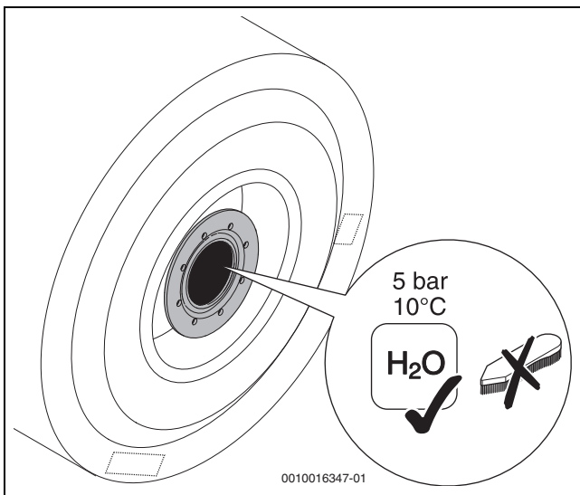
Fig. 84 Rocíe el acumulador
