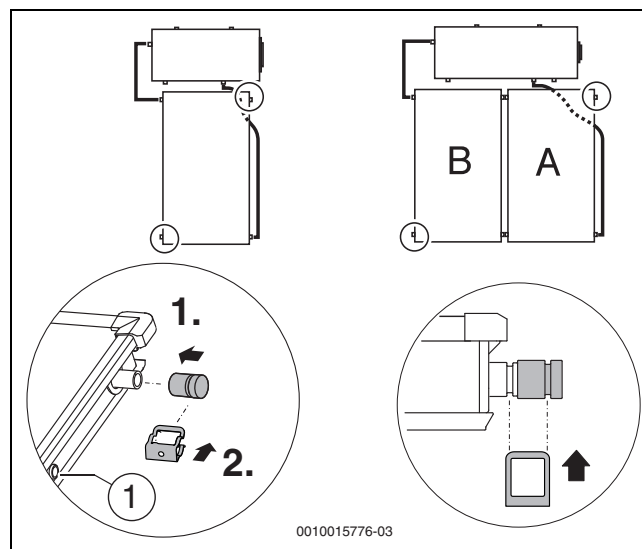
Fig. 43 Montar los tapones de cierre
