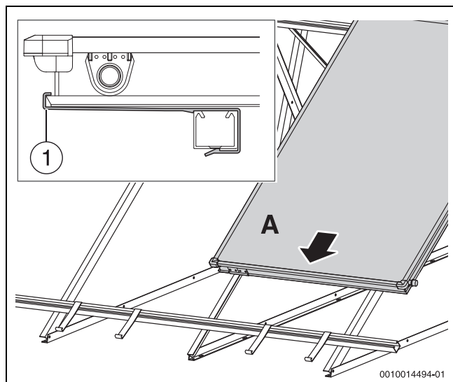
Fig. 46 Deje deslizar el colector derecho hasta los seguros contra deslizamiento
