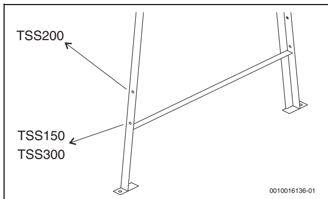
Fig. 36 Posiciones inferiores de fijación de la cruz para viento
