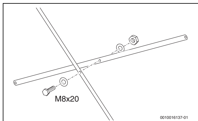
Fig. 35 Atornillar los perfiles planos
