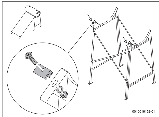
Fig. 40 MTSS1: Atornillar el pisador directamente en el soporte de montaje
