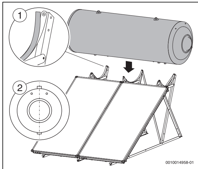
Fig. 63 Colocar el acumulador en el soporte para tejado plano y alinearlo
