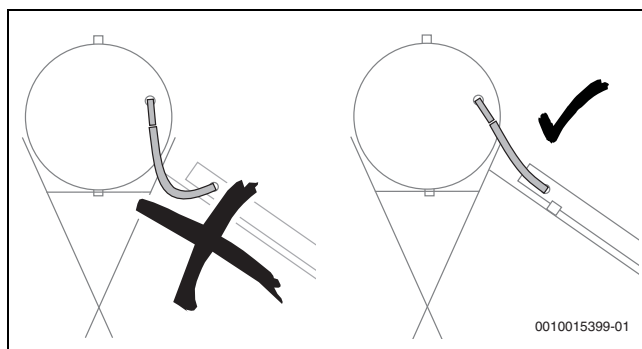
Fig. 65 No colocar una comba de la tubería (aquí: tubería de alimentación)
