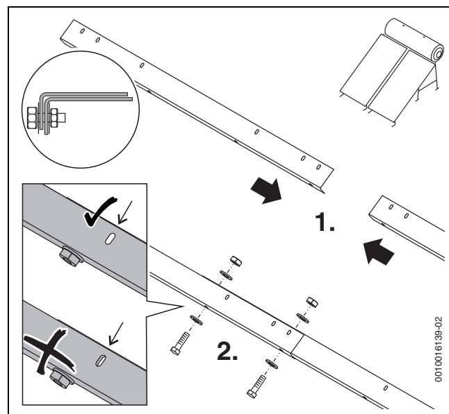
Fig. 38 Preinstalar perfiles angulares
