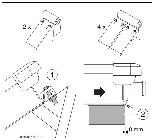
Fig. 53 Fijar el colector arriba
