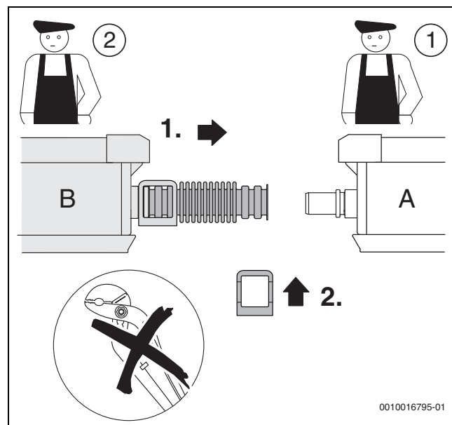
Fig. 54 Realizar el montaje del colector entre dos personas
