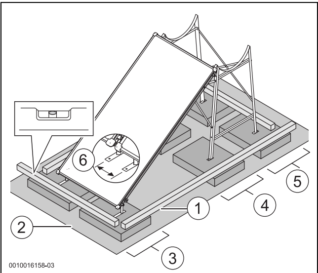
Fig. 59 Ejemplo TSS150/200: montaje en planchas de concreto
