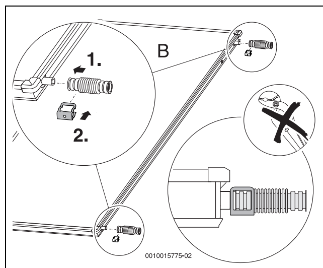
Fig. 44 Montar el set de conexión hidráulica en el colector izquierdo
