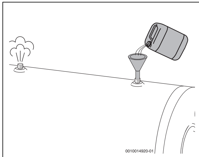
Fig. 75 Llenar líquido solar
