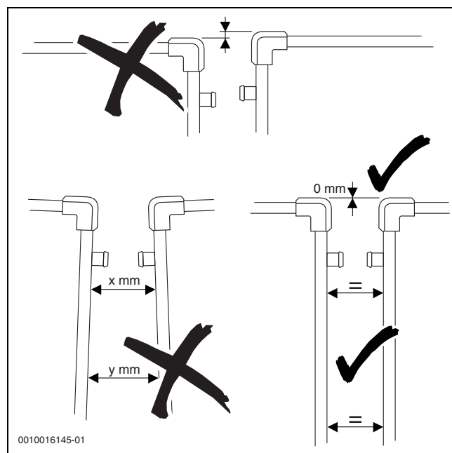
Fig. 62 Alinear correctamente los colectores
