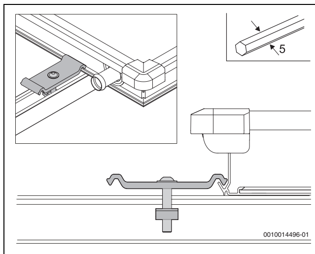
Fig. 48 Sólo colocar el tensor bilateral del colector
