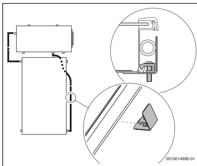
Fig. 69 Montar el soporte en el borde del colector
