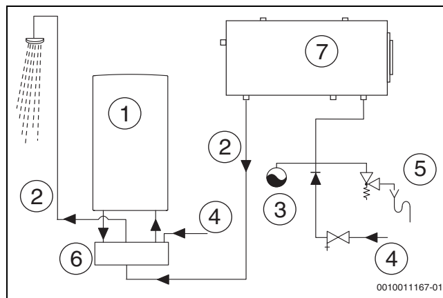
Fig. 72 Ejemplo de instalaciones con módulo solar
