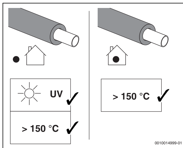
Fig. 77 Aislamiento de las tuberías
