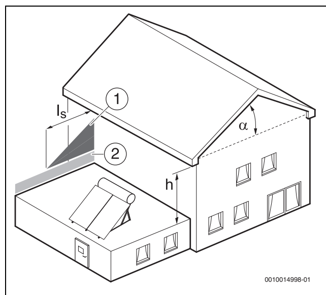
Fig. 11 Disposición de colectores por saltos de altura
