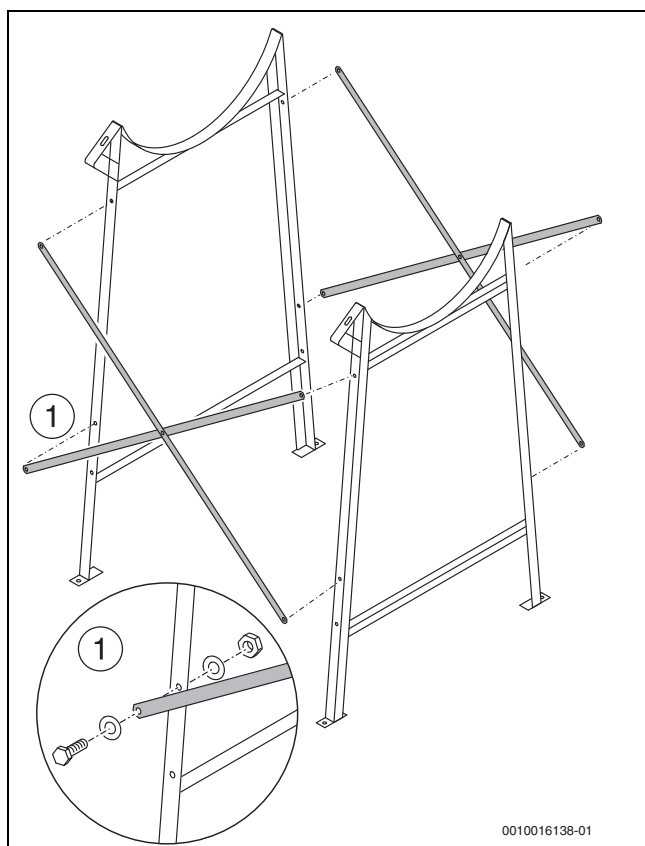
Fig. 37 Montar la cruz para viento (aquí: TSS200)
