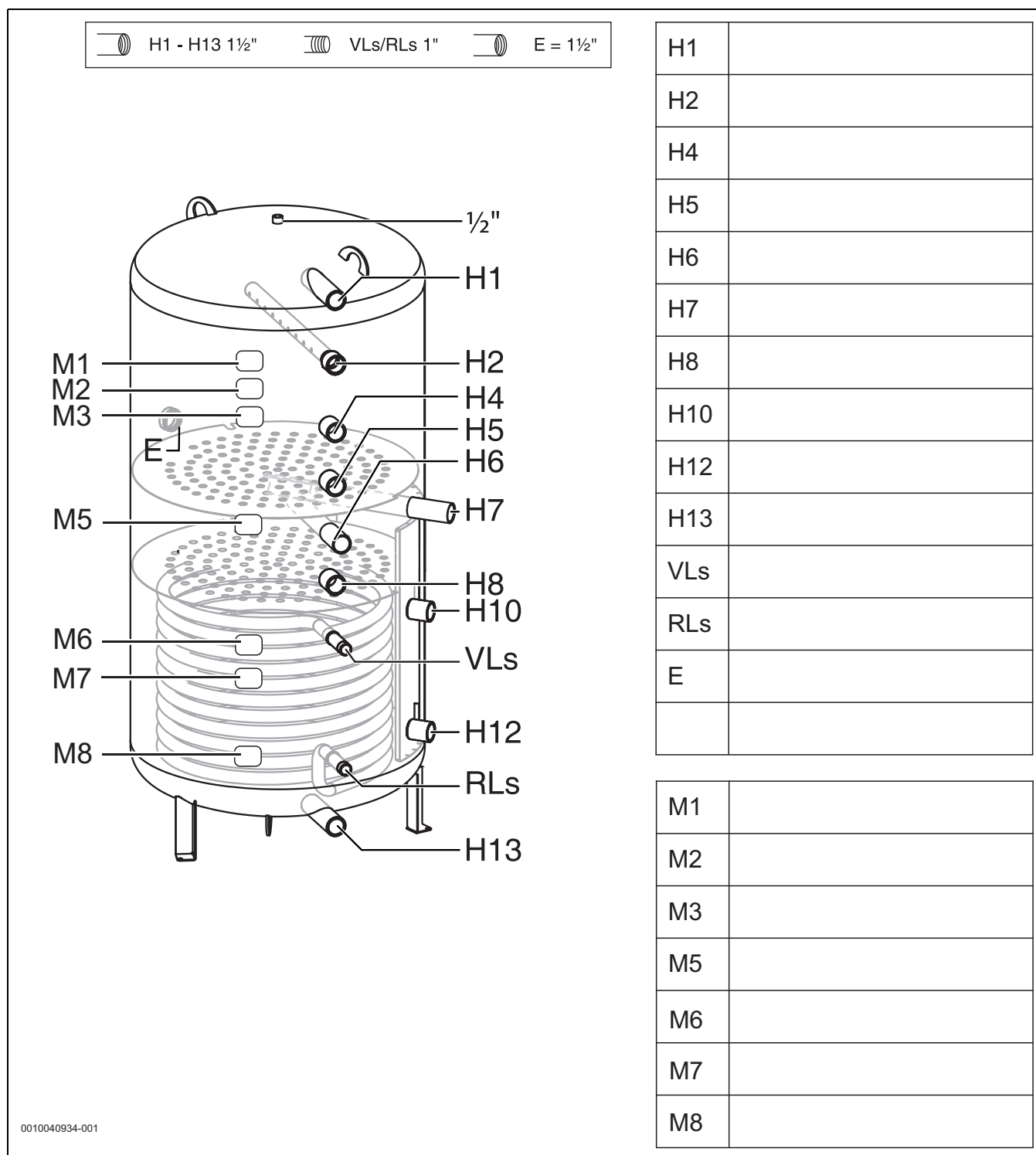
Fig. 30 BHS 750, 1000-6 ERZ
