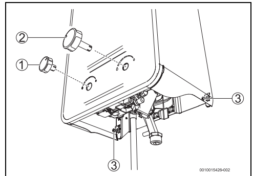
Fig. 13 Retirar la carcasa
