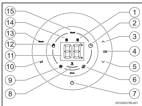
Bild 5 Bedienfeld
