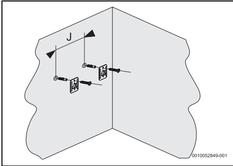
8. ábra Rögzítőpanelek
