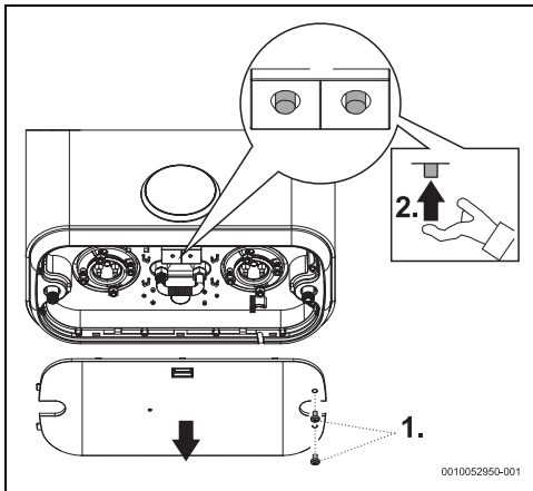
Rys. 16 Termostat zabezpieczający
