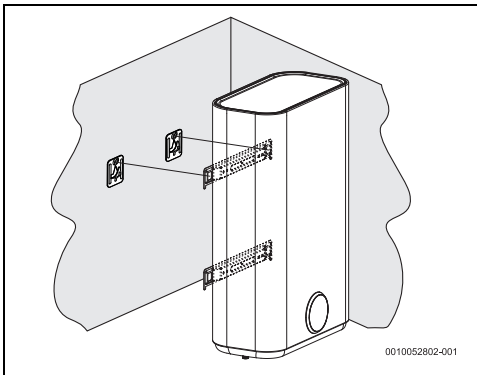
9. ábra Fügőleges telepítés (falra szerelés)
