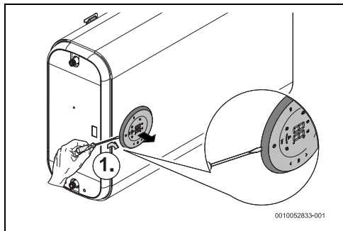
Fig. 12 Dégager l'écran
