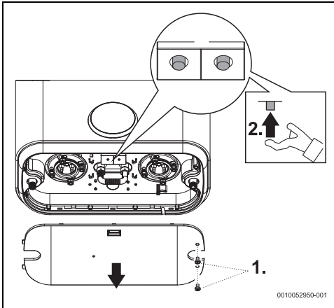
Bild 16 Sicherheits thermostat
