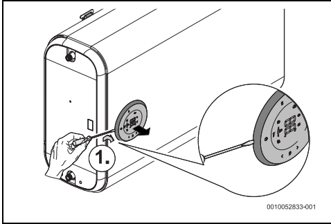
Fig. 12 Scoaterea afișajului
