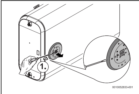
Rys. 12 Odłączanie wyświetlacza
