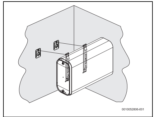
11. ábra Vízszintes telepítés (falra szerelés)
