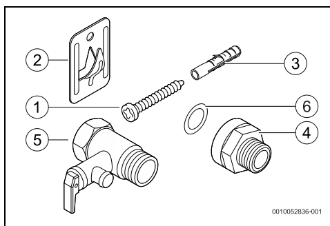
Fig. 1 Piezas suplidas
