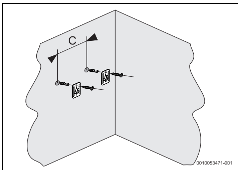
Bild 10 Montageplatten
