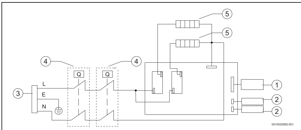
Bild 17 Anschlusschema
