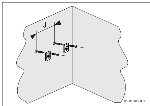
Bild 8 Montageplatten
