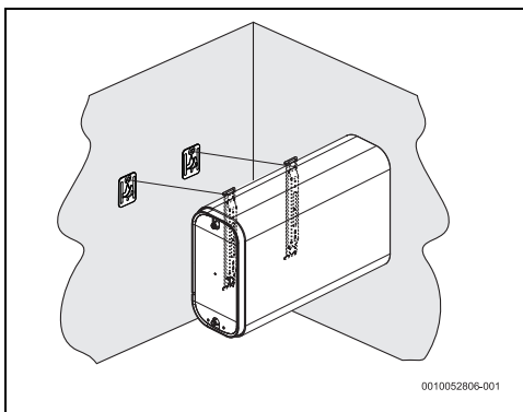
Fig. 11 Instalare orizontală (montare pe perete)
