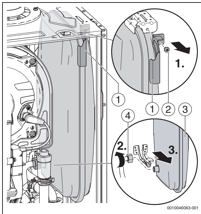
Fig. 132 Desmontar el vaso de expansión
