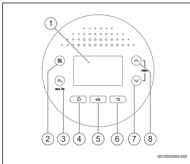
Fig. 28 Vista general del campo de mando
