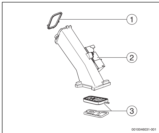
Fig. 113 Componentes del tubo de aire-gas
