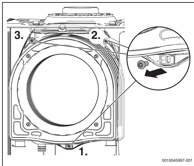
Fig. 99 Desmontar el intercambiador de calor
