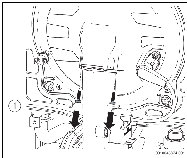
Fig. 121 Desmontaje de los tornillos
