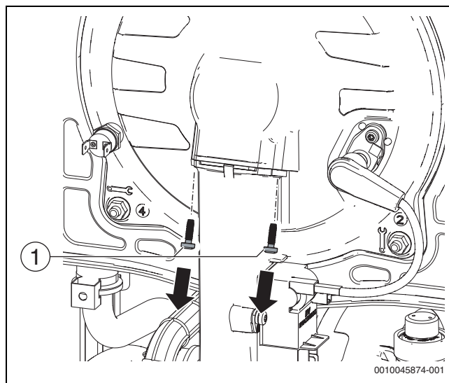
Fig. 112 Desmontaje de los tornillos
