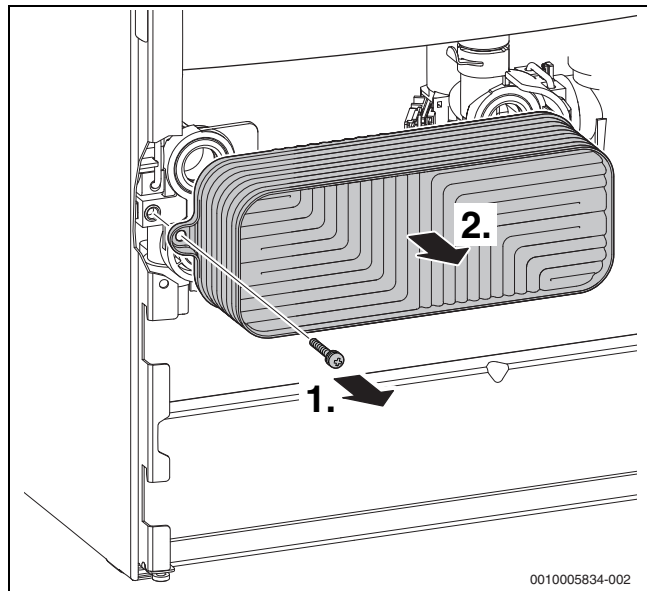
Fig. 138 Desmontar el intercambiador de placas
