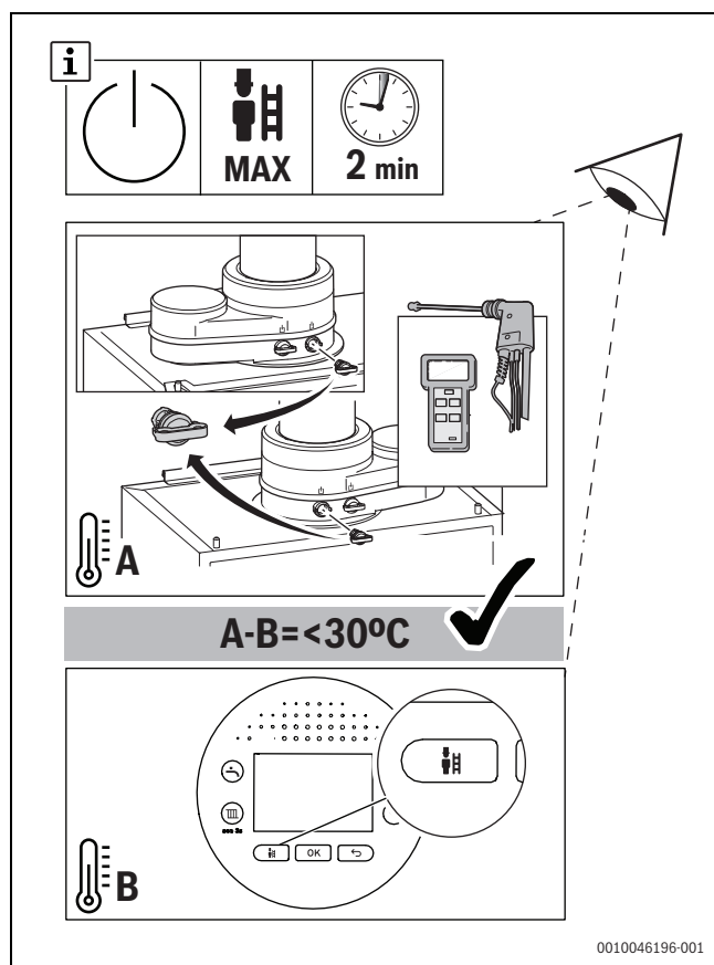
Fig. 72 Prueba de control dT
