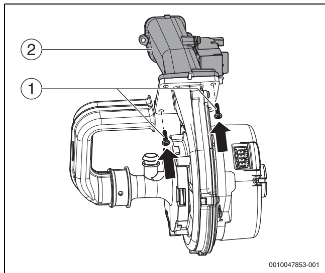
Fig. 114 Instalación del tubo de aire-gas
