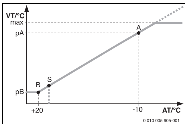
Fig. 152 Curva de calefacción
