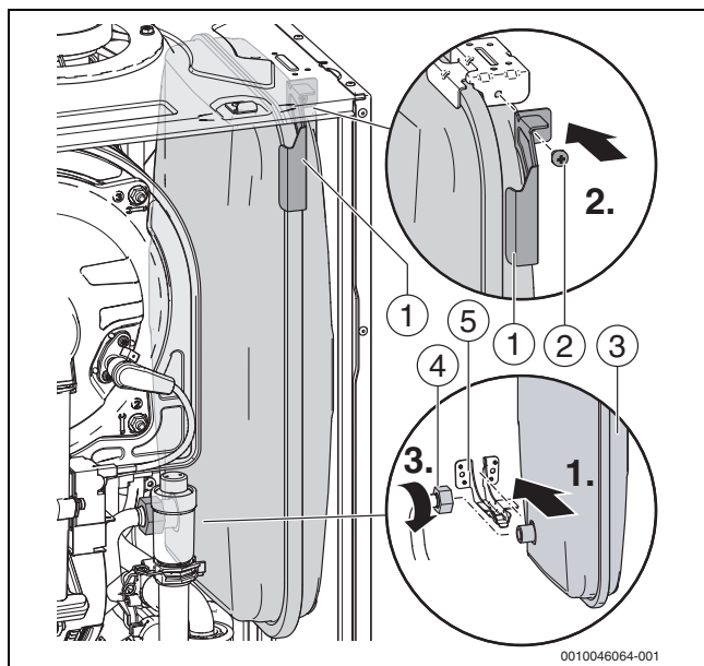
Fig. 133 Instalar un nuevo vaso de expansión
