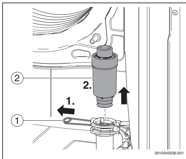
Fig. 95 Desmontar el purgador automático
