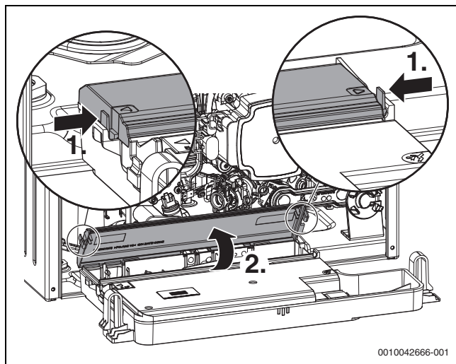
Fig. 25 Abrir la cubierta de mantenimiento
