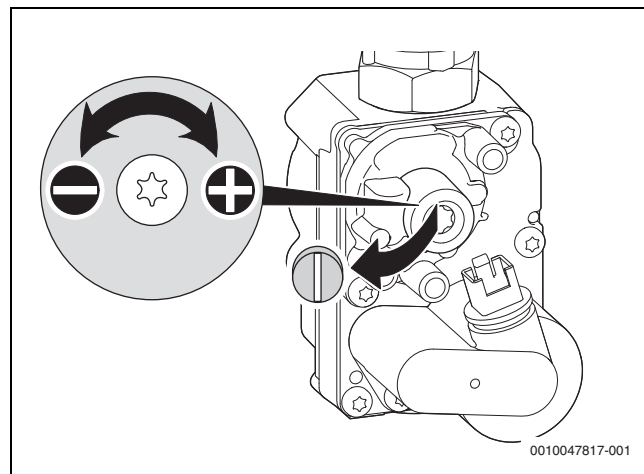
Fig. 33 Retirar el precinto en el tornillo de ajuste
