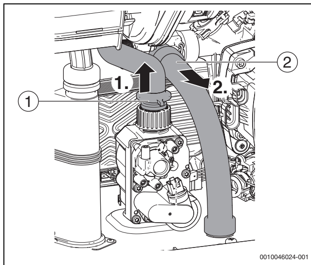
Fig. 139 Retirar la manguera de desagüe y de gas
