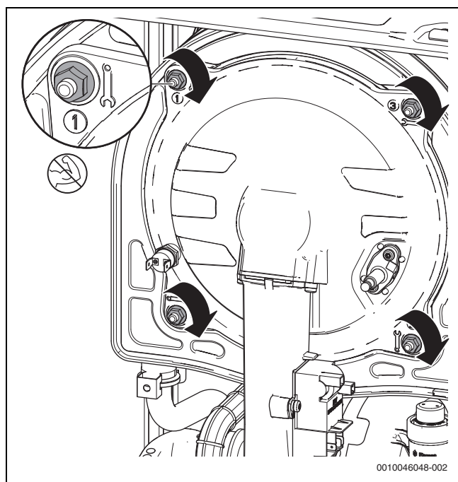
Fig. 123 Instalar el módulo de puerta de cámara de combustión en el intercambiador de calor
