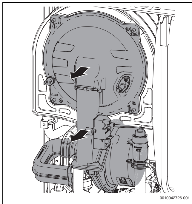
Fig. 94 Desmontar el módulo de puerta de cámara de combustión
