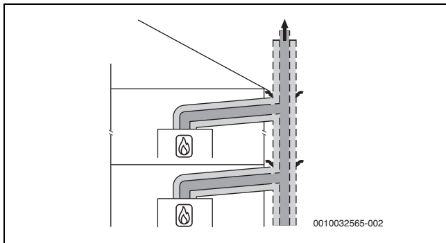
Fig. 15 Conexión múltiple según C_{(12)3x} con una instalación de evacuación de gases concéntrica en el lugar de instalación
