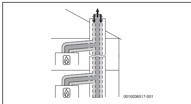
Fig. 13 Asignación múltiple según C_{43p} con guía concéntrica de aire/gases de escape en el lugar de montaje
