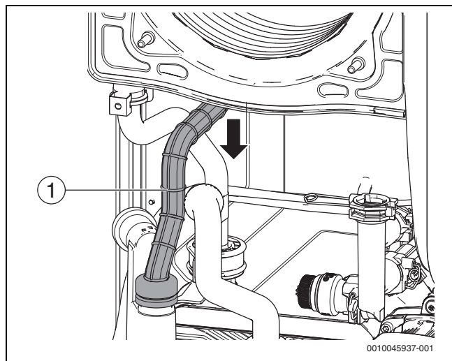
Fig. 96 Soltar el tubo de purga de condensados
