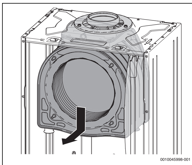
Fig. 100 Retirar el intercambiador de calor
