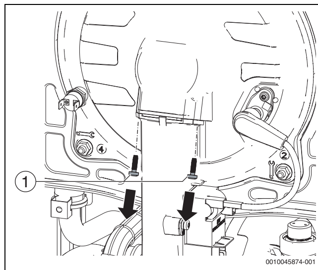
Fig. 74 Desmontaje de los tornillos
