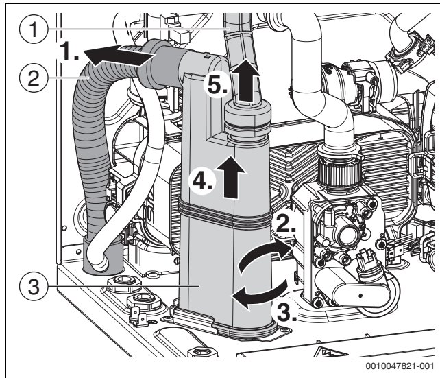
Fig. 48 Desmontar el sifón de condensado
