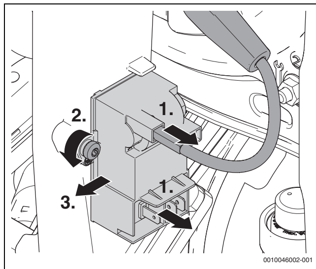
Fig. 103 Desmontar el transformador de encendido
