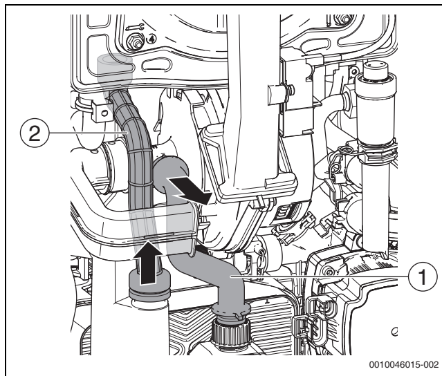
Fig. 107 Desmontar la manguera de evacuación de condensado y la de conexión de gas
