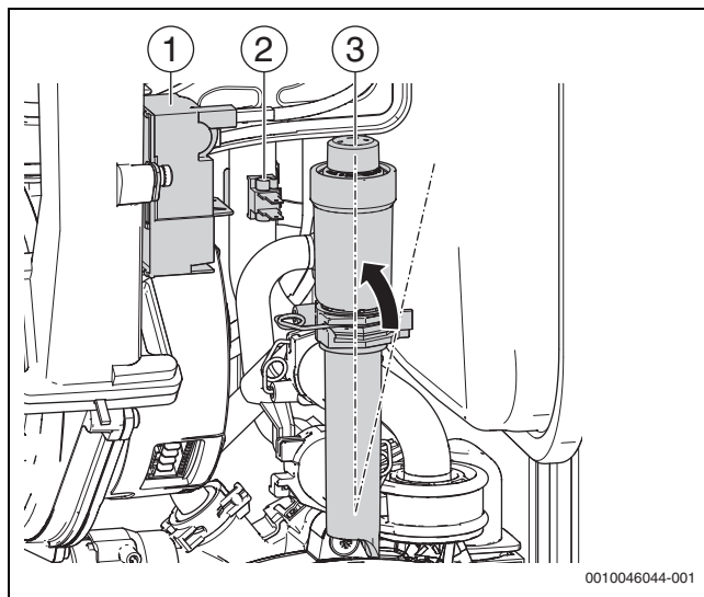
Fig. 127 Instalar el NTC nuevo en el tubo de retorno
