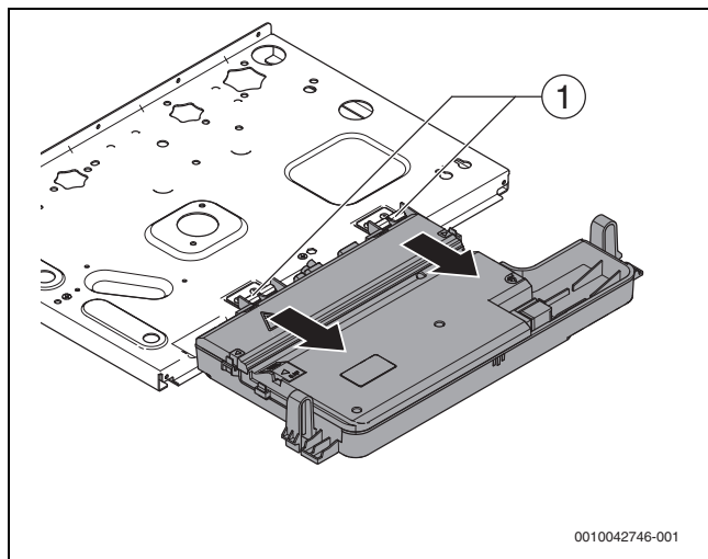
Fig. 134 Sustituir la unidad de mando
