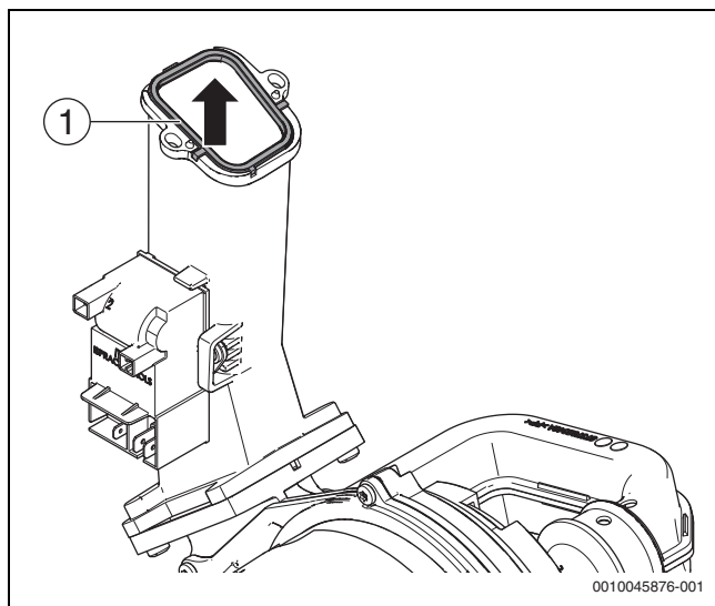
Fig. 76 Desmontaje de la junta
