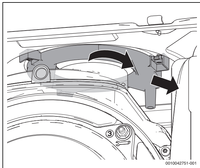
Fig. 146 Desmontar la protección contra la lluvia
