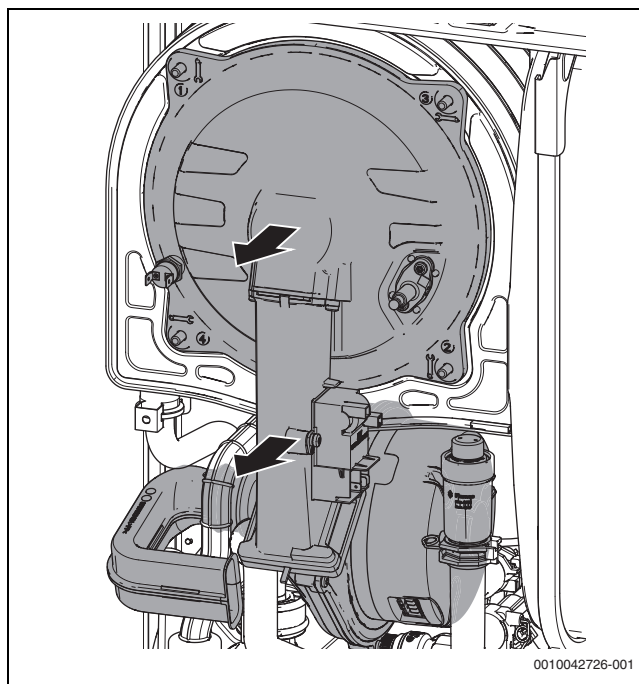
Fig. 40 Desmontar la puerta de la cámara de combustión
