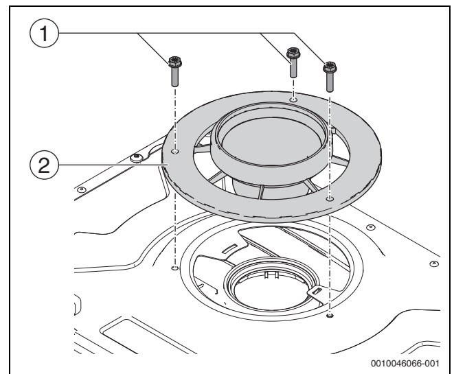
Fig. 57 Instalar el set y el adaptador del tubo de gases de escape
