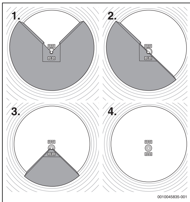
Fig. 68 Pasos para el desmontaje del aislamiento
