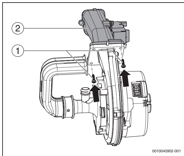
Fig. 81 Montaje del tubo de aire-gas, del ventilador y del seguro de reflujo
