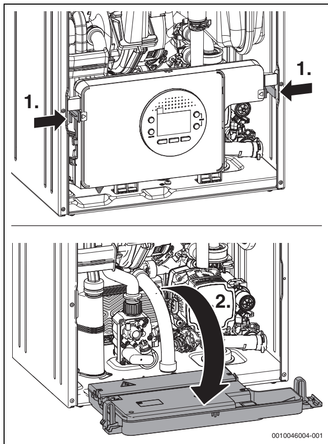
Fig. 24 Plegar la electrónica hacia abajo
