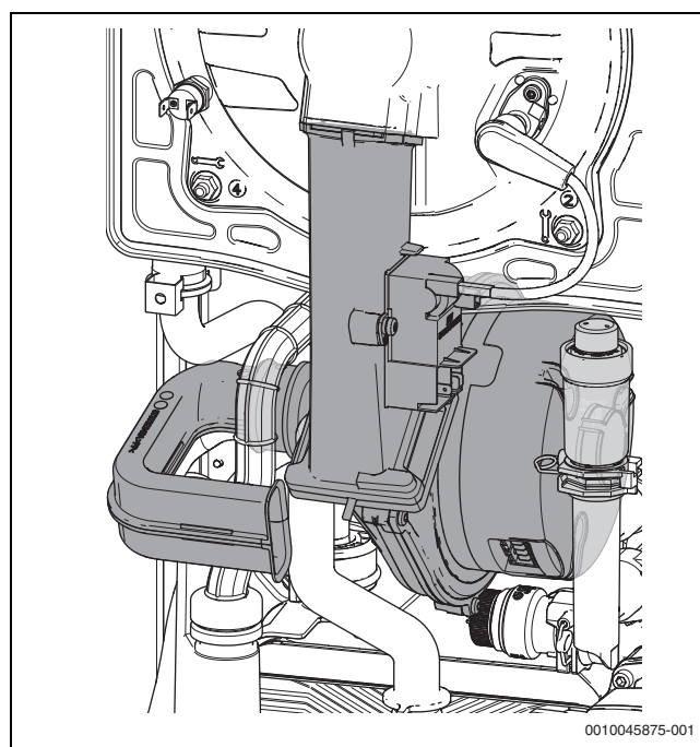
Fig. 75 Desmontaje de los componentes
