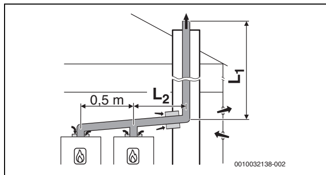
Fig. 16 Sistema en cascada con 2 aparatos: Conducción rígida de gases de evacuación por la chimenea después de B 53p con suministro de aire atmosférico en el aparato
