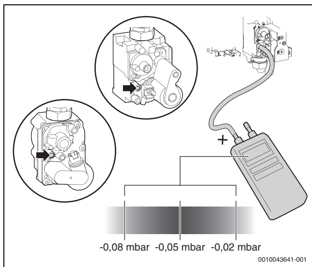
Fig. 32 Medir la presión diferencial
