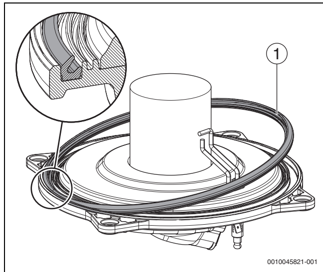
Fig. 65 Sustituir la junta bilabial
