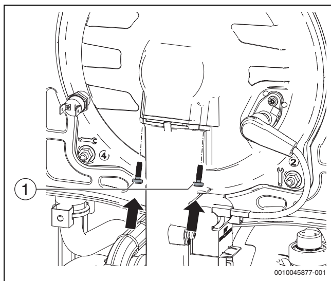
Fig. 77 Montaje de los tornillos en la puerta de la cámara de combustión
