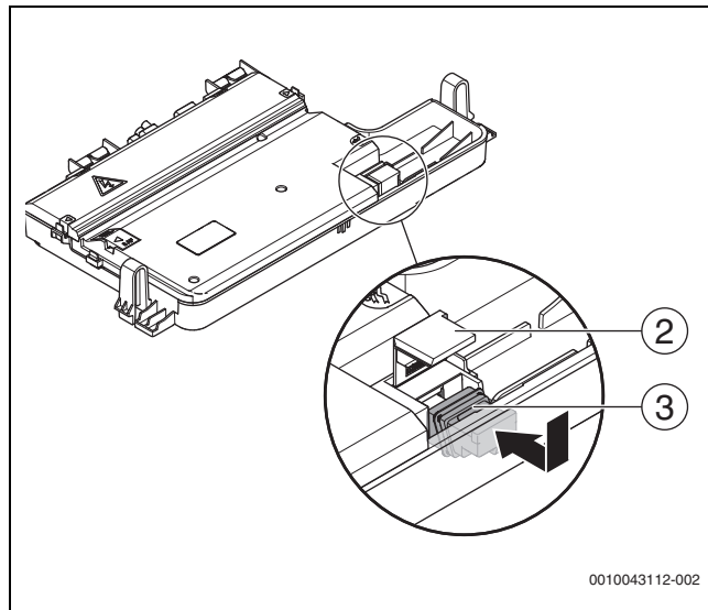
Fig. 135 Colocar el codificador
