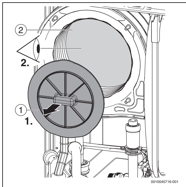
Fig. 46 Retirar la protección de aislamiento y comprobar el aislamiento
