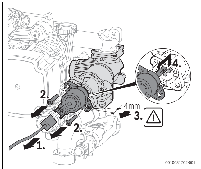
Fig. 147 Desmontar el motor en la válvula de 3 vías
