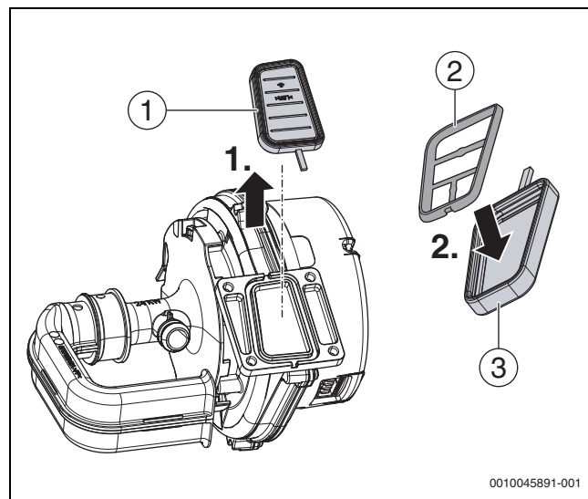
Fig. 79 Sustitución del seguro de reflujo
