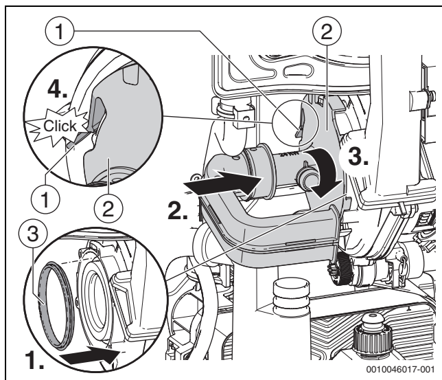
Fig. 109 Instalar una nueva tobera de Venturi
