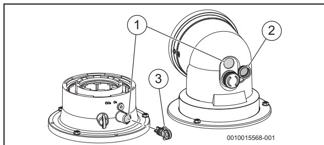
Fig. 30 Punto de medición para la comprobación de la estanqueidad de la tubería de gases de escape
