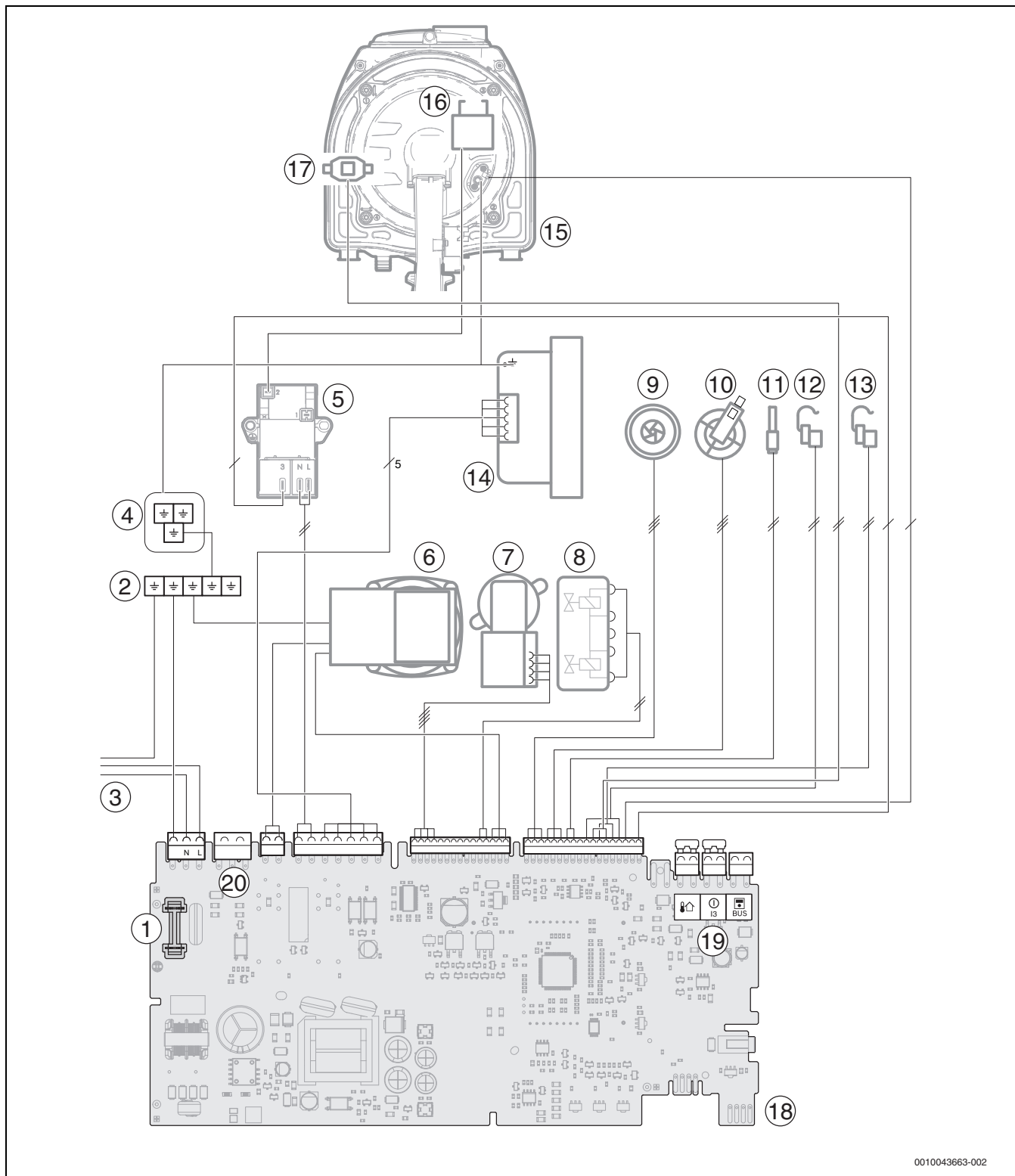
Fig. 151 Cableado eléctrico
