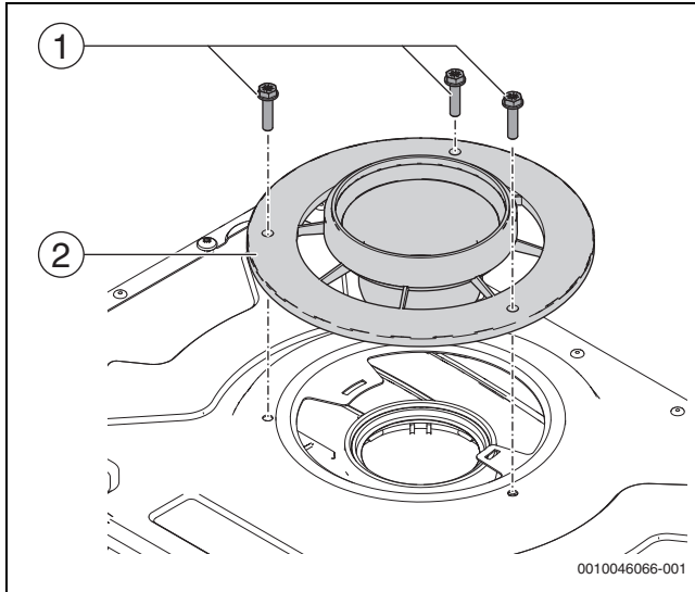
Fig. 54 Desmontar el set y el adaptador del tubo de gases de escape
