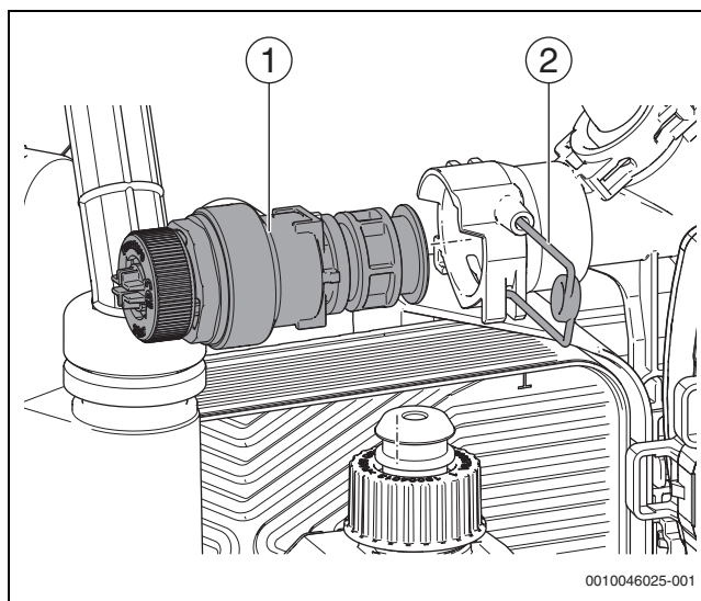
Fig. 140 Desmontar la válvula de seguridad
