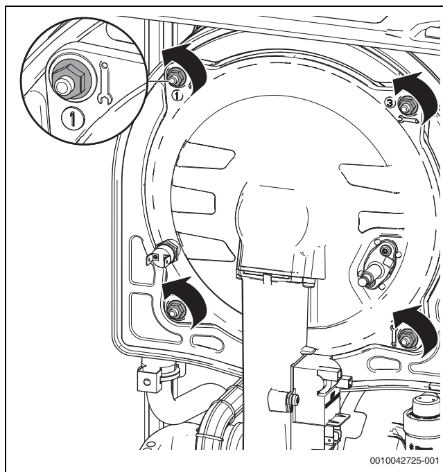
Fig. 39 Retirar las tuercas de fijación
