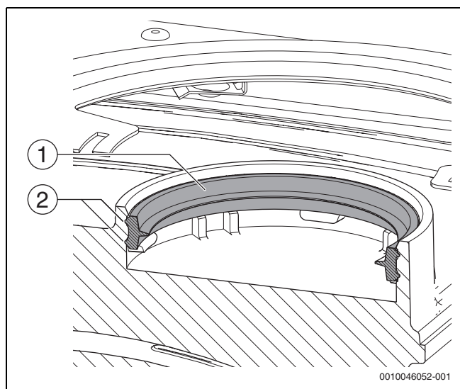
Fig. 131 Instalar una nueva junta bilabial
