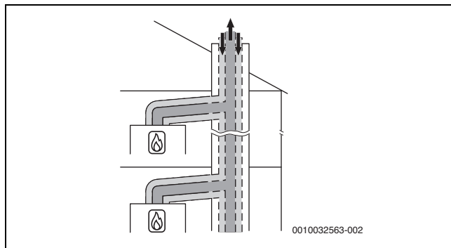
Fig. 14 Conexión múltiple según C_{(10)3x} con una instalación de evacuación de gases concéntrica en el lugar de instalación
