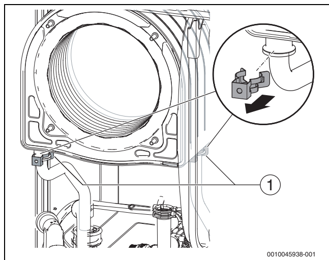
Fig. 97 Desmontar las abrazaderas
