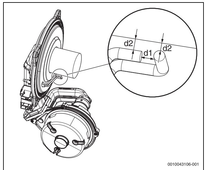
Fig. 50 Comprobar el electrodo de ionización y de encendido
