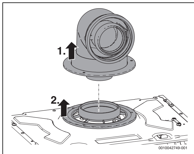
Fig. 144 Desmontar el set de tubo salida de gases de escape
