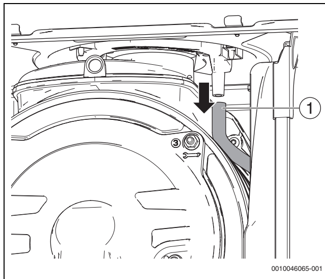
Fig. 53 Desmontar la manguera de salida de agua
