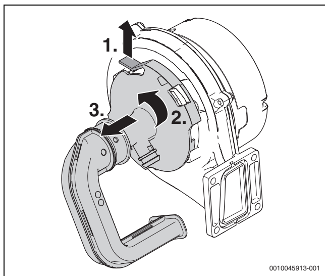
Fig. 85 Desmontaje del ventilador
