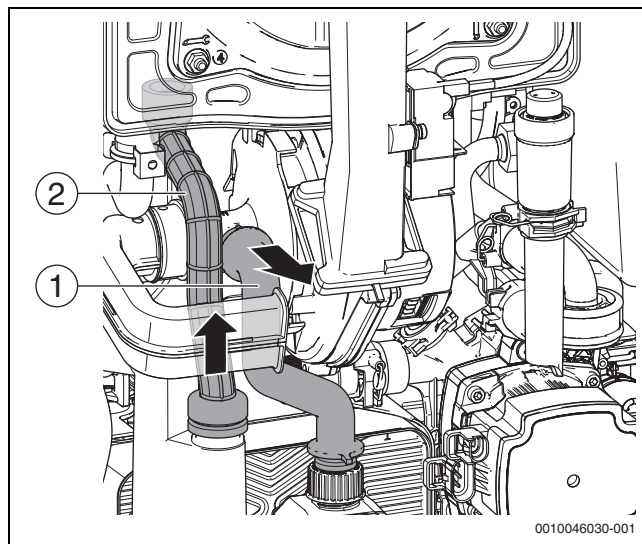
Fig. 111 Retirar la manguera de condensados y de gas
