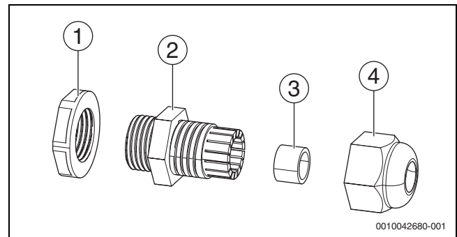
Fig. 23 Piezas del atornillamiento de cables
