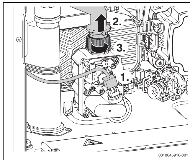
Fig. 87 Desmontaje de la manguera de conexión de gas, de la conexión de enchufes y de la tuerca
