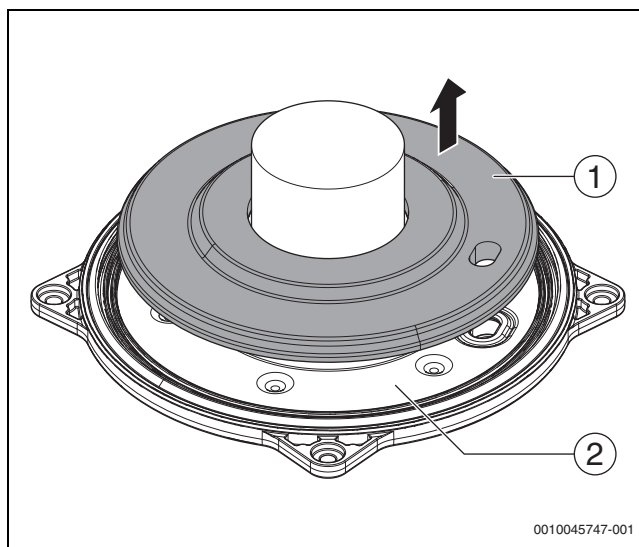
Fig. 61 Desmontar el aislamiento
