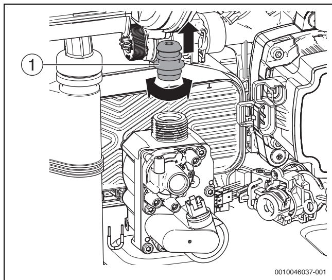
Fig. 117 Desmontar la válvula de mariposa primaria
