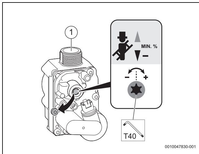
Fig. 52 Ajustar la concentración de CO 2 (arriba válvula SIT, abajo válvulas Honeywell)
