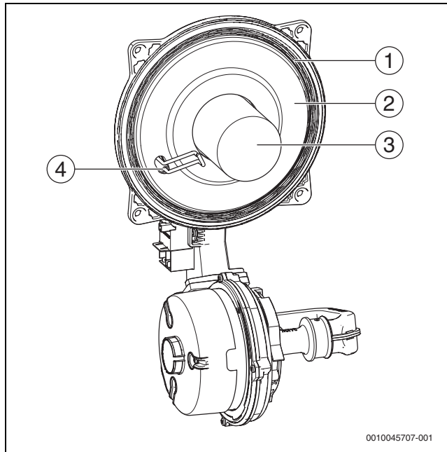
Fig. 47 Puerta de la cámara de combustión
