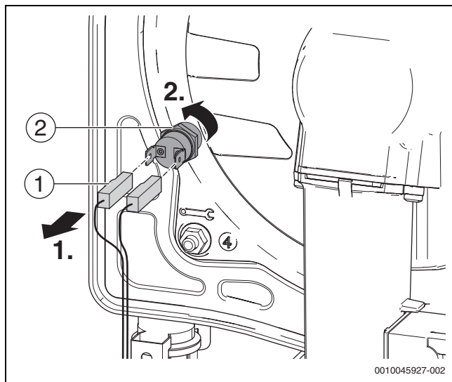
Fig. 92 Desmontaje del limitador de temperatura
