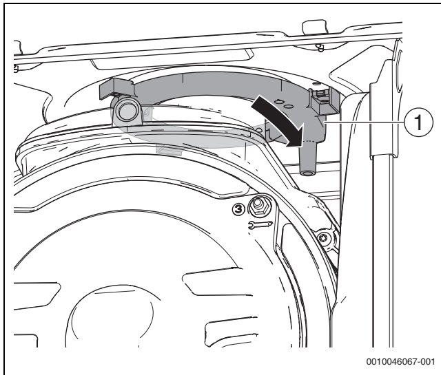
Fig. 55 Desmontar la protección contra las lluvias
