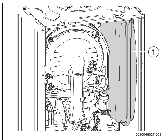
Fig. 59 Comprobar el vaso de expansión
