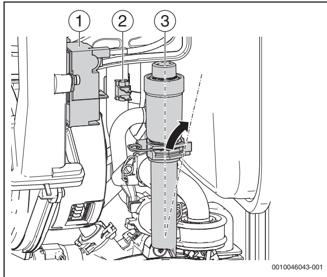
Fig. 126 Desmontar el NTC en el tubo de retorno
