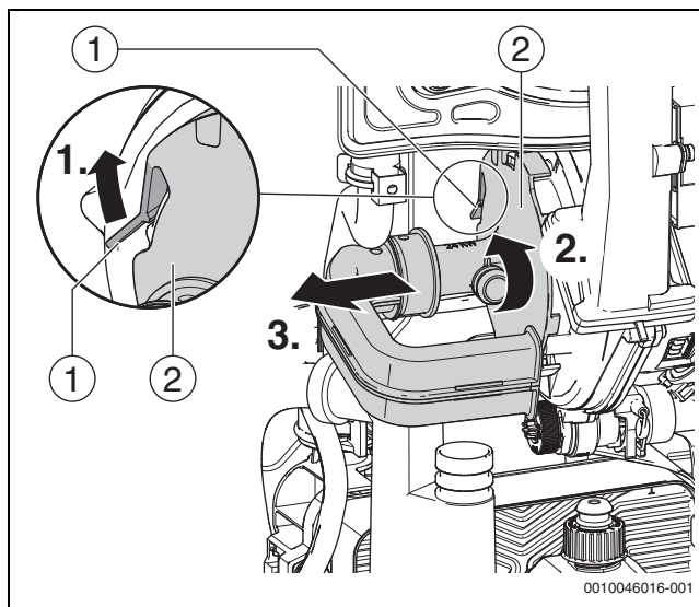
Fig. 108 Desmontar la tobera de Venturi
