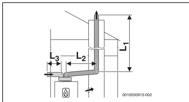
Fig. 9 Conducción rígida de evacuación según C 53 y conducción de la evacuación de gases, con tubos separados para el acceso de aire de admisión y evacuación de gases
