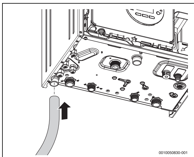
Fig. 19 Montar la manguera en el sifón de condensado
