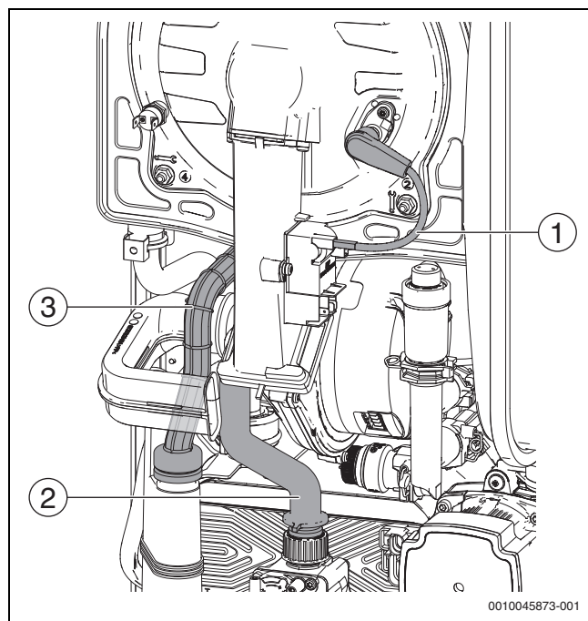
Fig. 73 Puerta de la cámara de combustión
