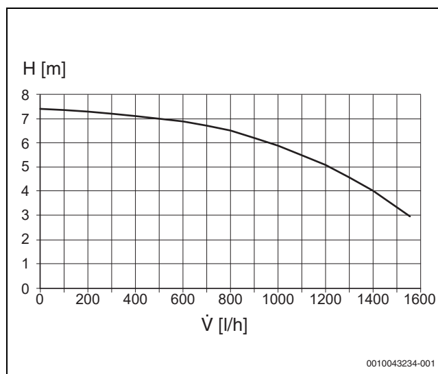
Fig. 27 Curva característica de la bomba de circulación (número constante de revoluciones)
