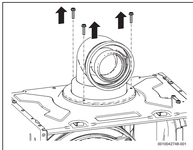
Fig. 143 Retirar los tornillos de sujeción
