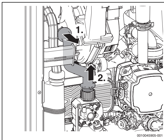
Fig. 83 Desmontaje de la manguera de conexión de gas
