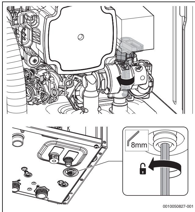
Fig. 60 Punto de vaciado
