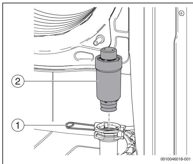
Fig. 136 Sustituir el purgador automático
