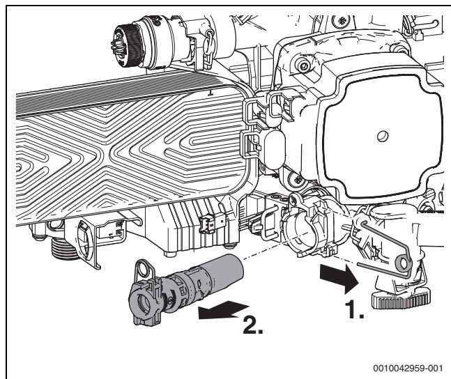
Fig. 137 Sustituir el silenciador
