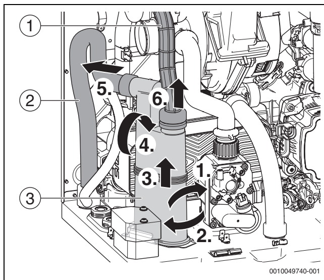
Fig. 49 Desmontar el sifón de condensado
