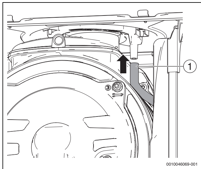
Fig. 58 Instalar la manguera de salida de agua
