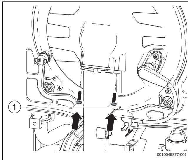
Fig. 115 Montaje de los tornillos en la puerta de la cámara de combustión
