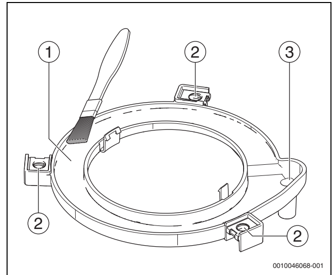
Fig. 56 Limpiar la protección contra las lluvias
