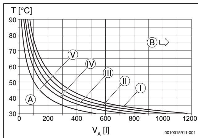
Fig. 17 Líneas características del vaso de expansión
