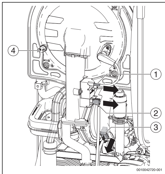
Fig. 37 Desconectar la conexión eléctrica
