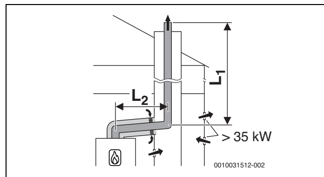
Fig. 11 Conducción canalizada rígida de la evacuación de gases según B 33 con suministro de aire de admisión mediante la instalación concéntrica de la evacuación de gases en el lugar de instalación
