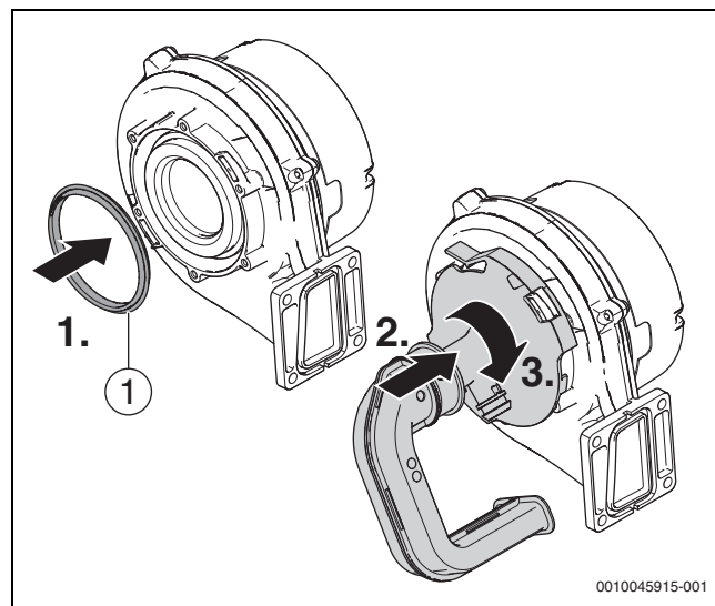
Fig. 86 Montaje del ventilador
