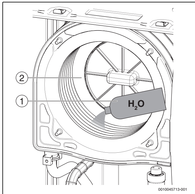
Fig. 45 Enjuagar con agua
