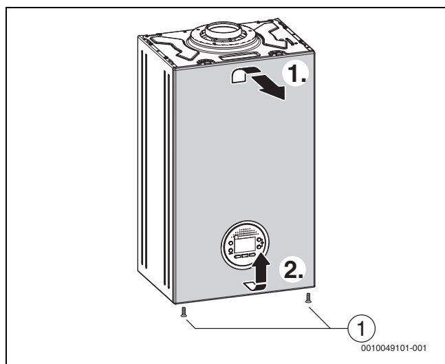
Fig. 18 Retirar la carcasa frontal
