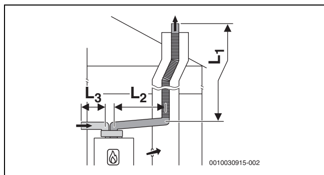
Fig. 10 Conducción flexible de gases de evacuación según C 53 y conducción rígida de la evacuación de gases con tubos separados para el acceso de aire de admisión y evacuación de gases
