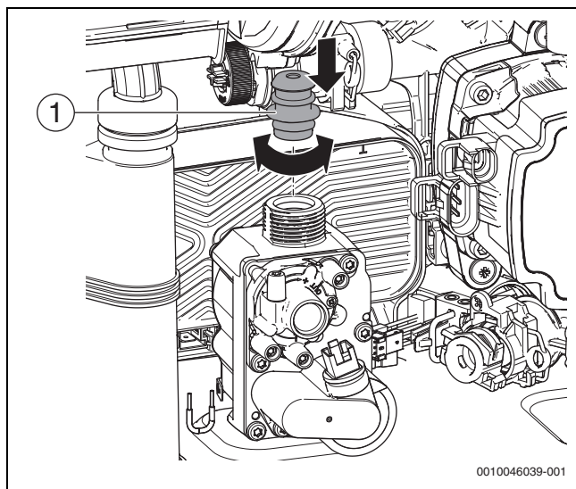
Fig. 119 Colocar la nueva válvula de mariposa primaria y la tuerca de gas
