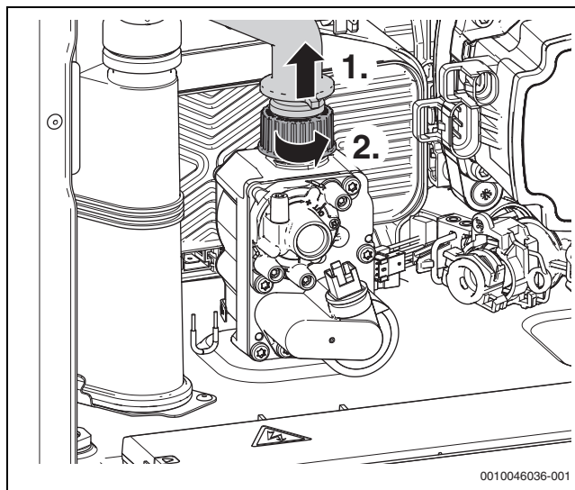
Fig. 116 Desmontar la manguera de conexión de gas y la tuerca de gas
