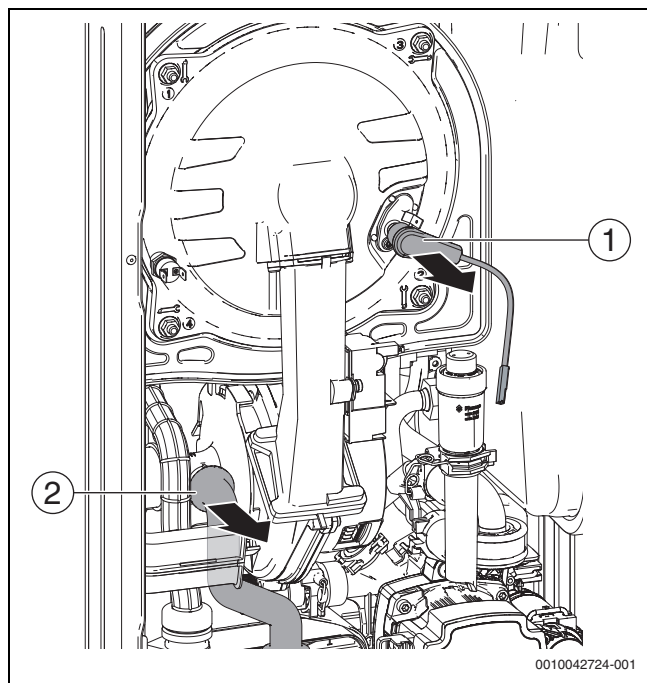
Fig. 38 Soltar el cable de encendido del set de electrodos y retirar la manguera de gas
