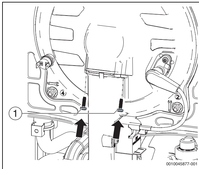
Fig. 82 Montaje del tubo de aire-gas en la puerta de la cámara de combustión
