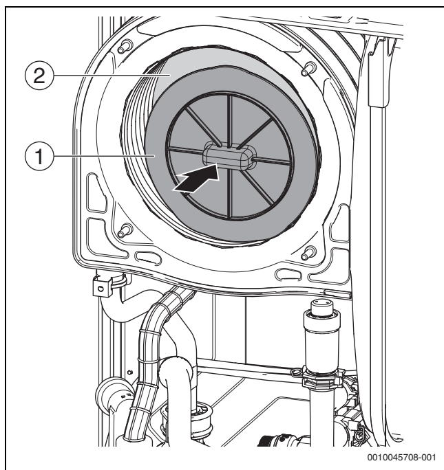
Fig. 42 Protección de aislamiento
