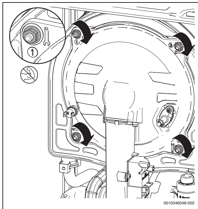
Fig. 63 Instalar el módulo de puerta de cámara de combustión en el intercambiador de calor
