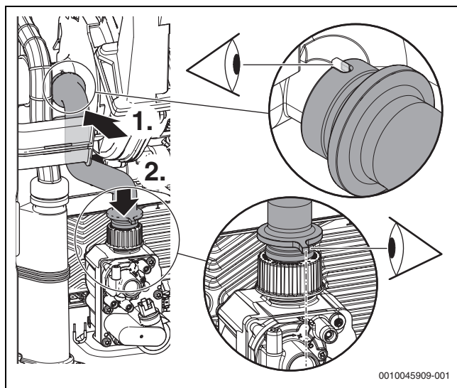
Fig. 84 Montaje de la manguera de conexión de gas
