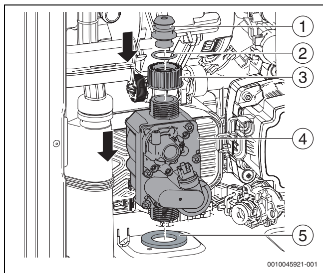
Fig. 89 Montaje de la válvula del gas
