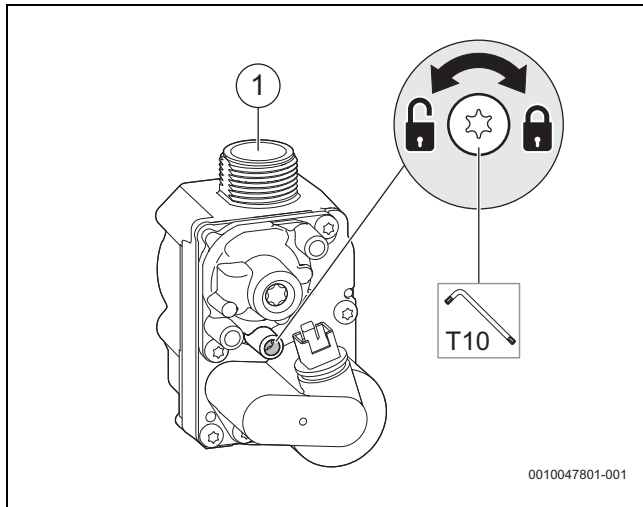
Fig. 29 Comprobar la presión de entrada del gas
