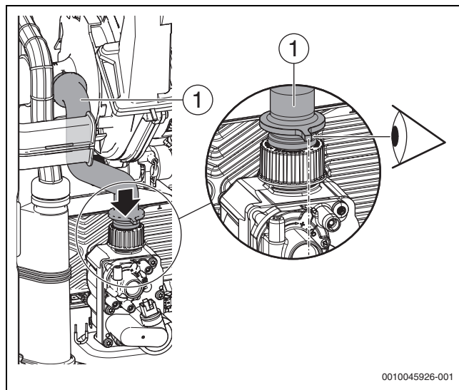
Fig. 120 Colocar y alinear la manguera de conexión de gas
