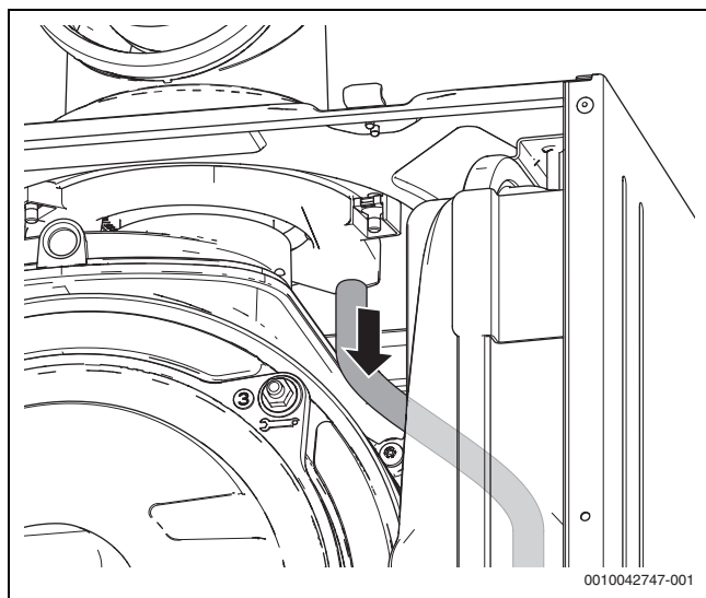
Fig. 142 Desmontar la protección contra la lluvia
