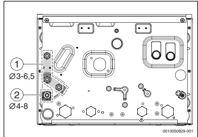
Fig. 22 Diámetros de cables
