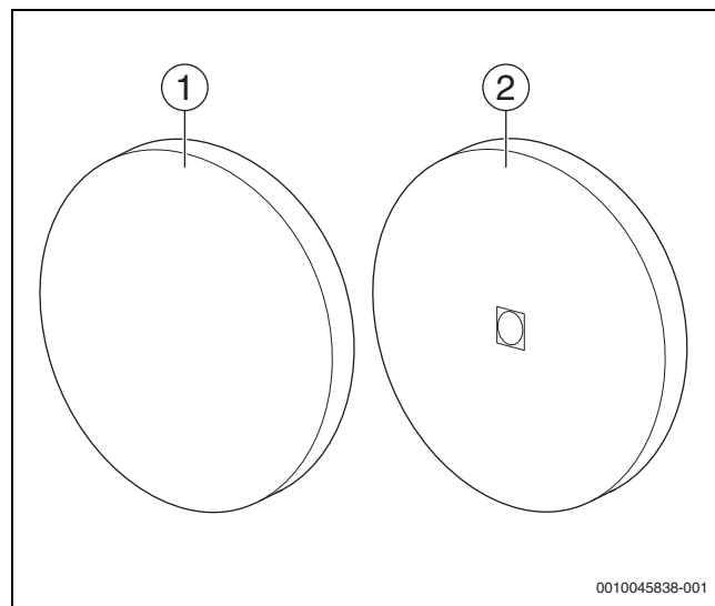
Fig. 70 Lado delantero y posterior del disco de aislamiento
