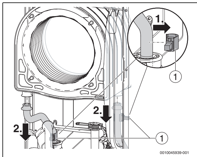
Fig. 98 Desmontar los NTC y los tubos
