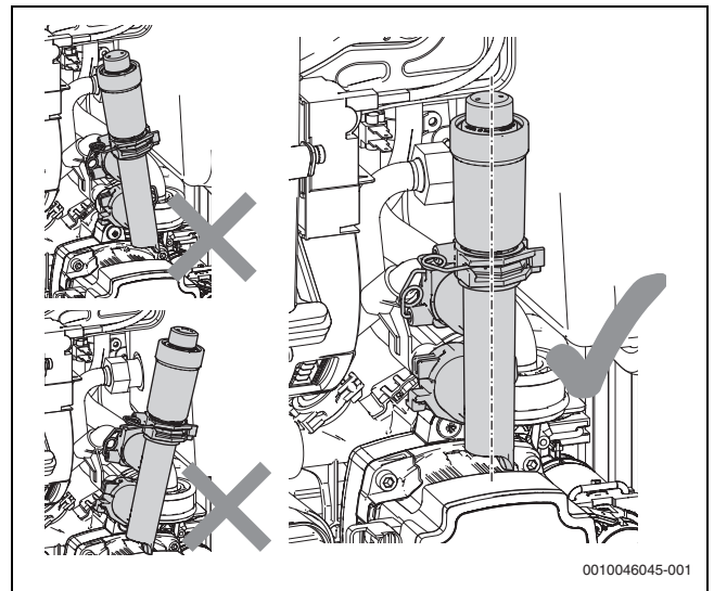
Fig. 128 Posición del purgador de aire
