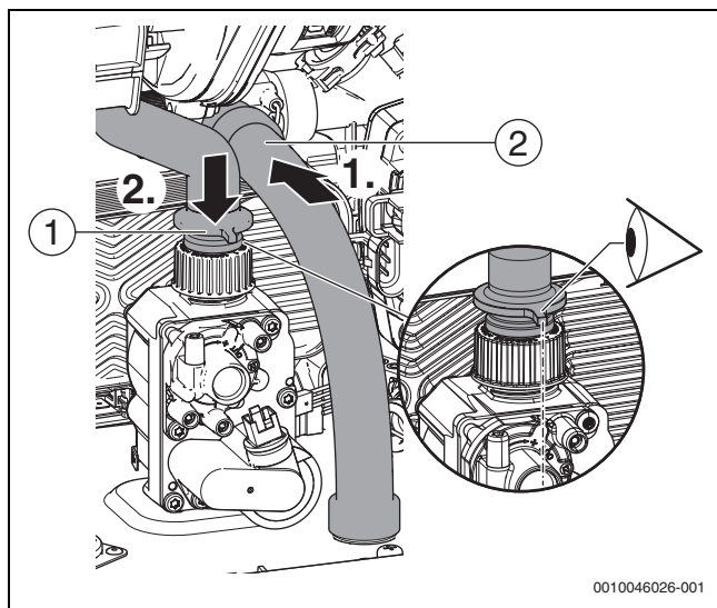
Fig. 141 Instalar la manguera de desagüe y de gas
