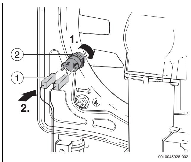
Fig. 93 Montaje del limitador de temperatura
