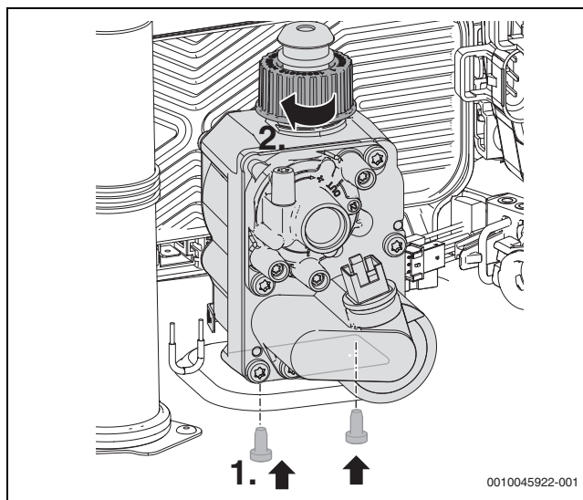
Fig. 90 Montaje del tornillo y de la tuerca
