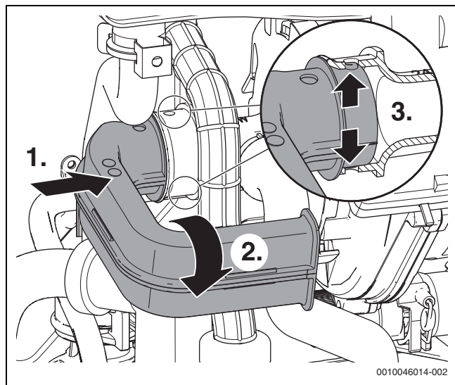
Fig. 106 Instalar un nuevo tubo de aire de entrada
