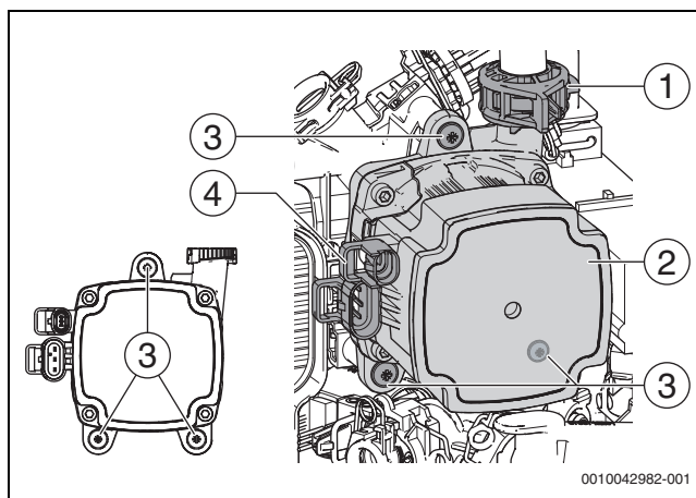
Fig. 149 Desmontar la bomba de calefacción
