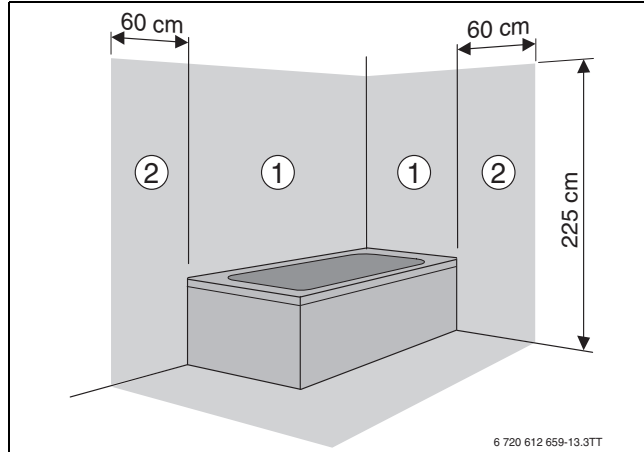
Fig. 21 Áreas de protección
