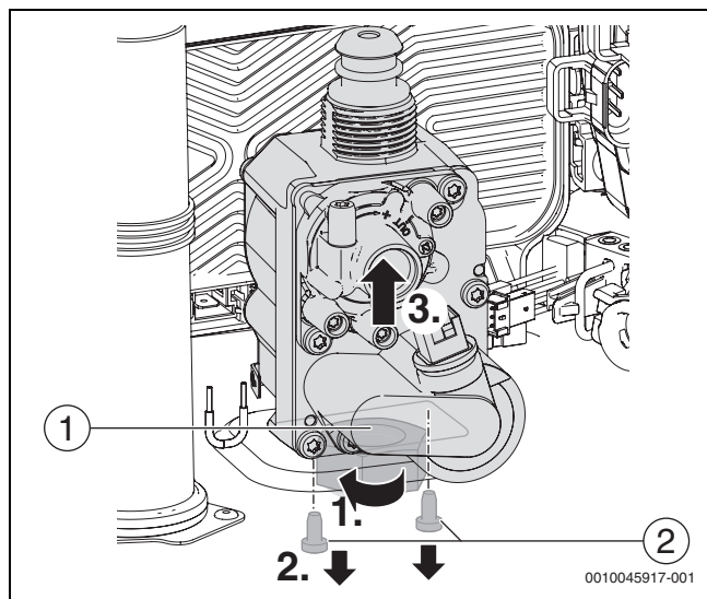
Fig. 88 Desmontaje de la válvula del gas
