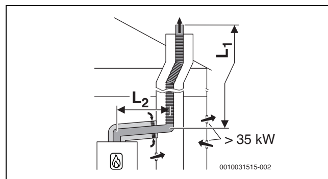
Fig. 12 Conducción canalizada flexible de la evacuación de gases según B 33 con suministro de aire de admisión mediante la instalación concéntrica de la evacuación de gases en el lugar de instalación
