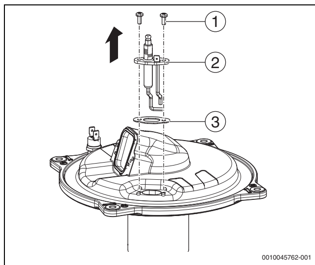
Fig. 64 Desmontaje del electrodo de encendido
