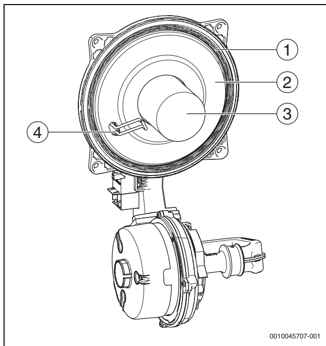
Fig. 41 Módulo de puerta de cámara de combustión
