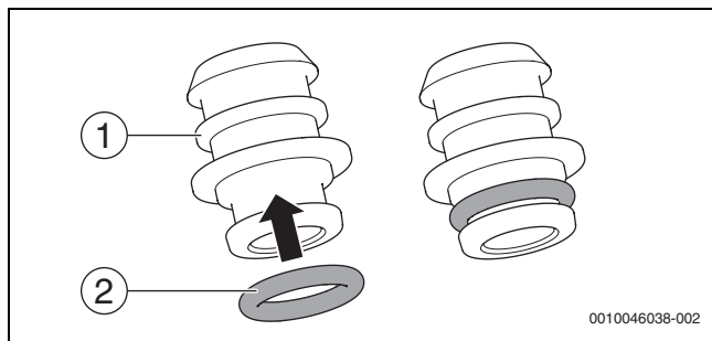
Fig. 118 Colocar la junta tórica en la válvula de mariposa primaria
