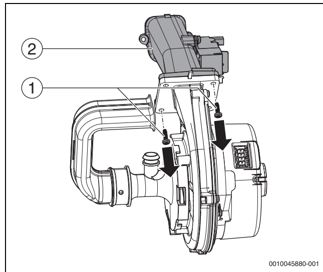
Fig. 78 Desmontaje del tubo de aire-gas
