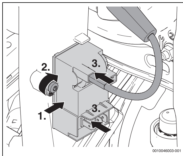
Fig. 104 Instalar el nuevo transformador de encendido
