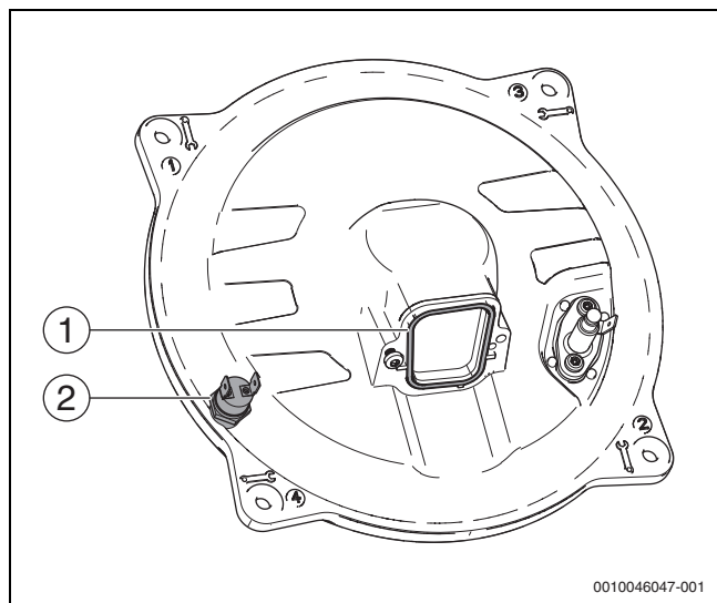
Fig. 122 Módulo de puerta de cámara de combustión
