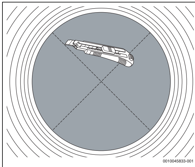
Fig. 66 Separar el material aislante
