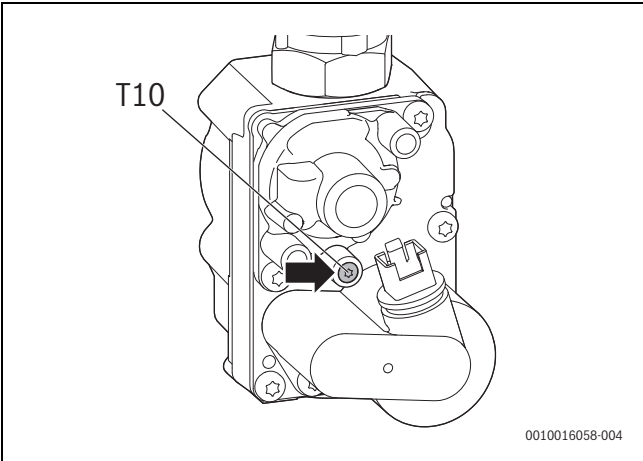
Fig. 34 Racor de medición para la presión de conexión de gas
