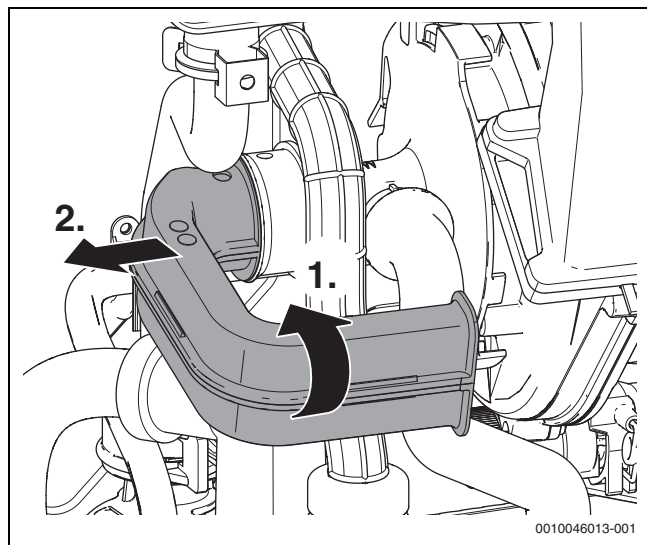
Fig. 105 Desmontar el tubo de aire de entrada
