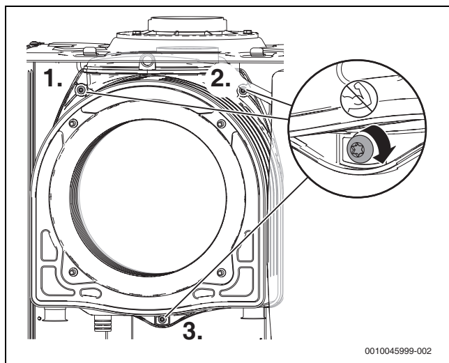
Fig. 101 Instalar el intercambiador de calor nuevo
