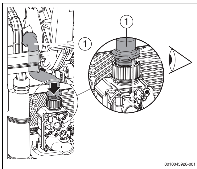
Fig. 91 Montaje de la manguera de conexión de gas
