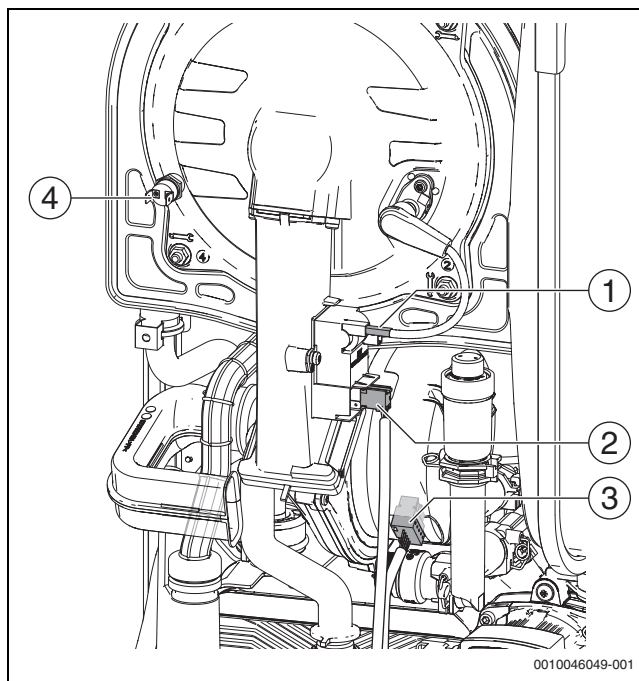
Fig. 124 Conectar el cable
