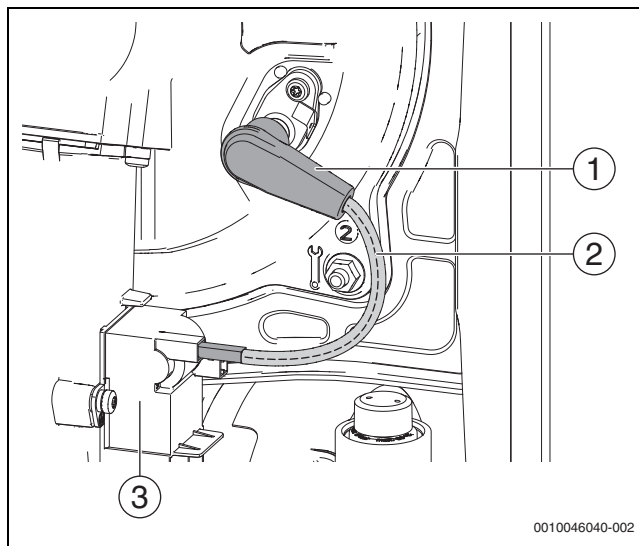
Fig. 125 Sustituir el cable de encendido
