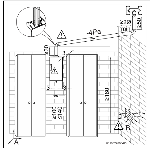
Fig. 8 Distancias mínimas
