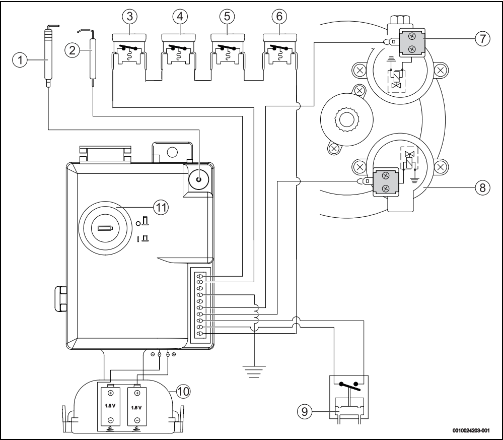
Fig. 30 Esquema eléctrico
