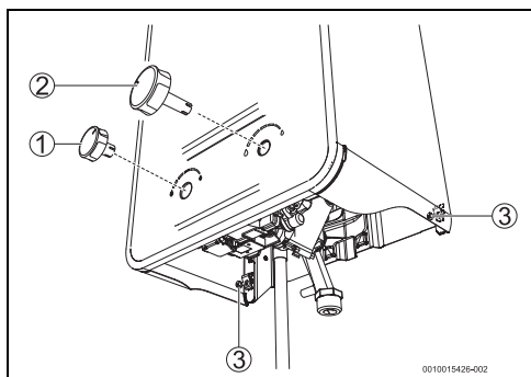
Fig. 16 Retirar la carcasa
