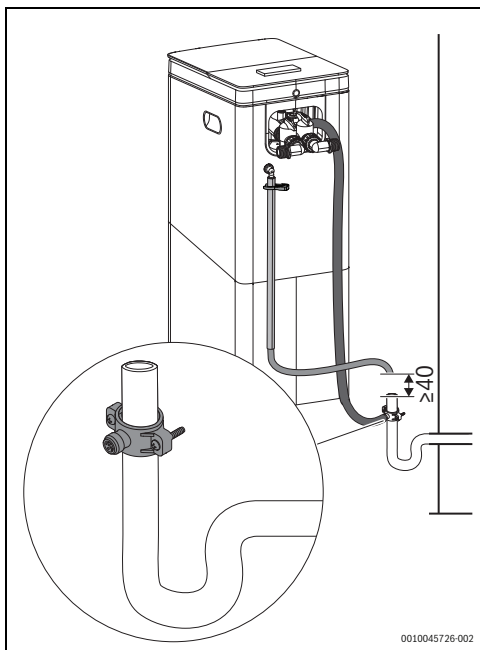
Fig. 12 Instalación del tubo de rebose y el tubo de drenaje al mismo tiempo
