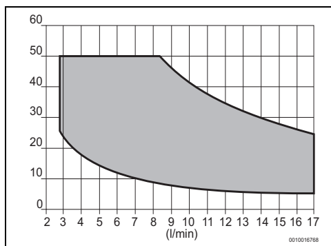
Fig. 29 Modelo 17 litros
