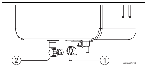
Fig. 15 Purga
