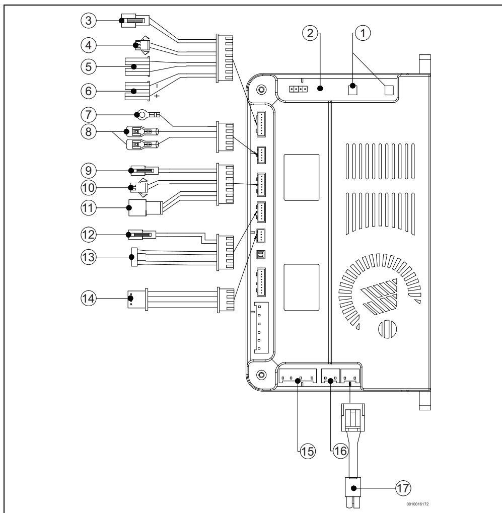
Fig. 26 Esquema de conexión
