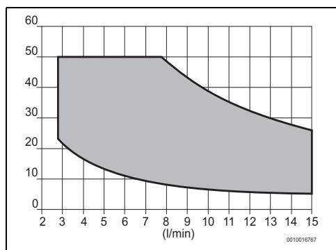
Fig. 28 Modelo 15 litros
