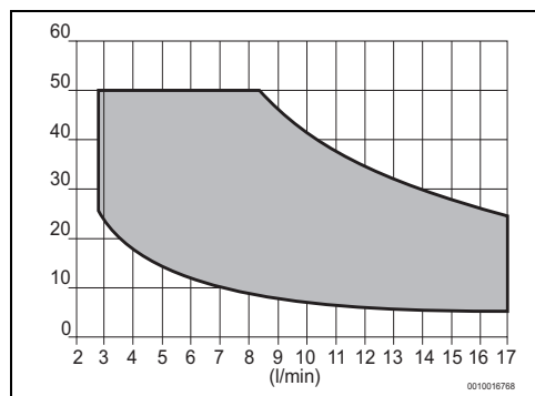
Fig. 29 Modelo 17 litros
