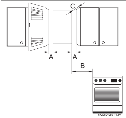
Fig. 19 Distancias mínimas
