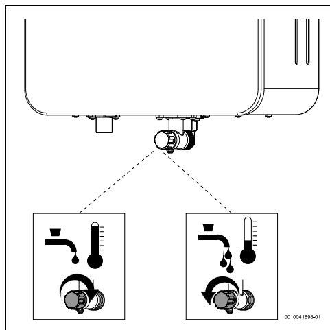
Fig. 7 Regulación del caudal
