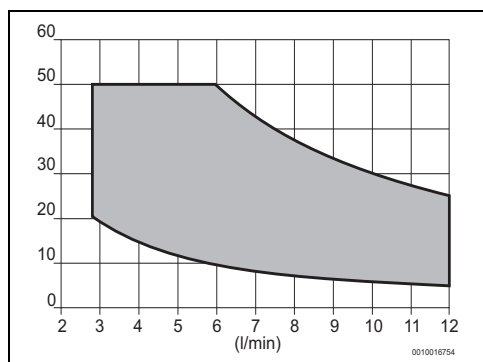
Fig. 27 Modelo 12 litros
