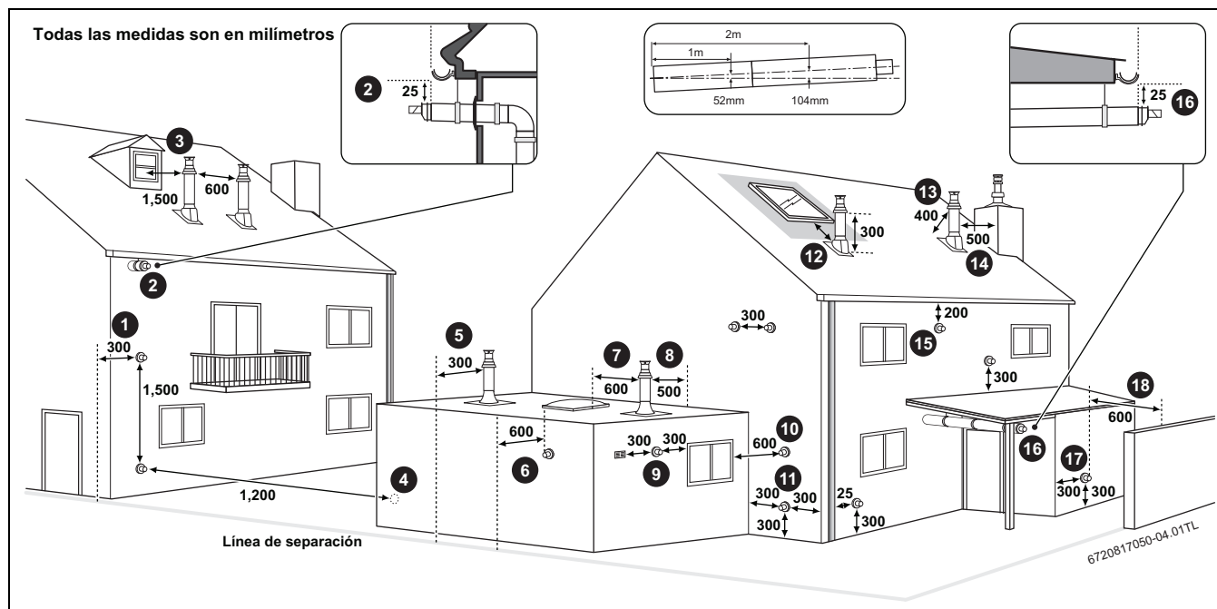
Fig. 29 Posiciones terminales del conducto de evacuación
