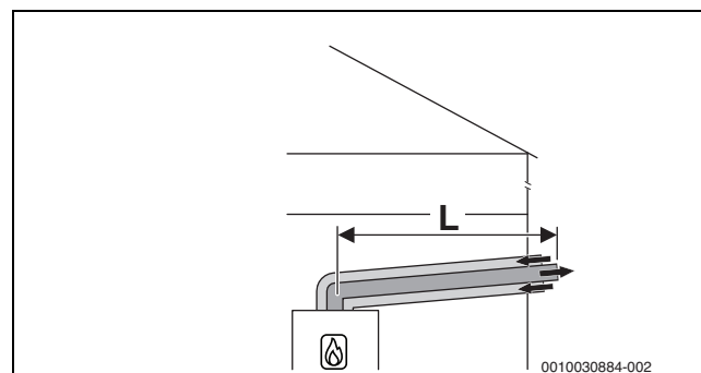
Fig. 6 Instalación de gas de escape concéntrica horizontal según C 13x mediante la pared externa
