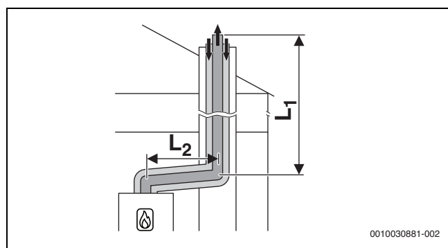
Fig. 7 Conducción concéntrica de la mezcla gas-aire hacia C 33x
