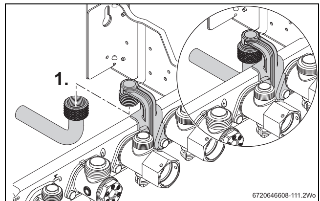
Fig. 40 Conexión de tubería de válvula de seguridad
