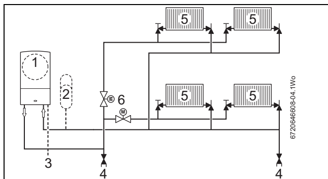
Fig. 16 Sistema cerrado con válvulas de zonas
