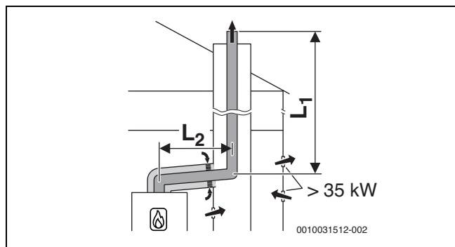
Fig. 11 Dirección rígida del conducto de gases de escape a través de un canal según B 33 con suministro de aire atmosférico mediante la instalación concéntrica de gas de escape en el lugar de instalación
