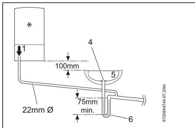
Fig. 18 Eliminación de condensado a un tubo de salida
