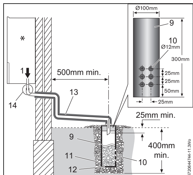
Fig. 23 Pozo absorbente
