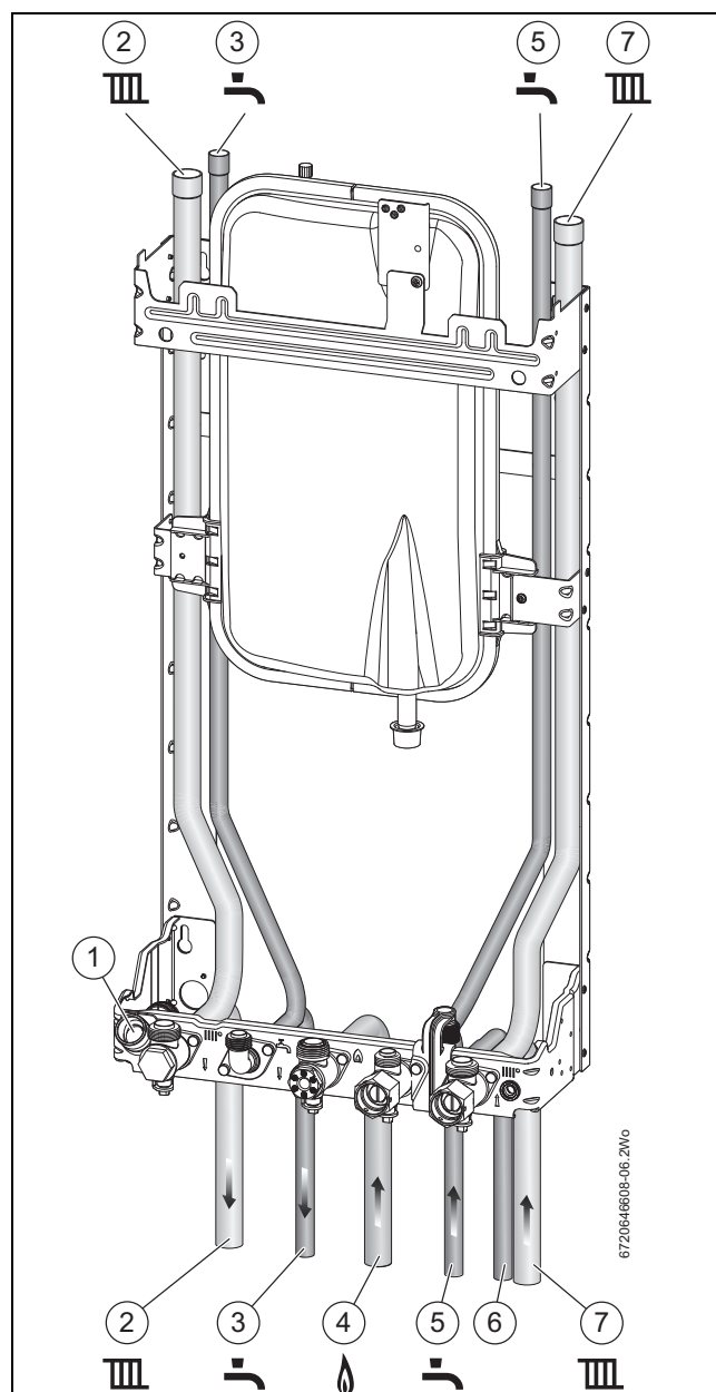
Fig. 28 Tuberías
