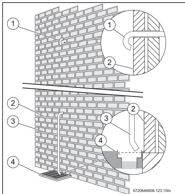
Fig. 24 Tubería de desagüe de la válvula de seguridad
