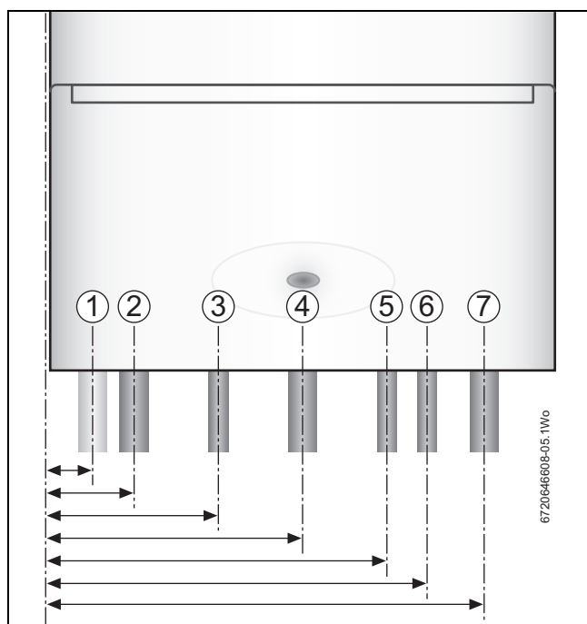
Fig. 27 Distancias y diámetros de los tubos
