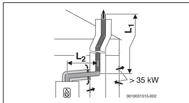
Fig. 12 Dirección flexible del conducto de gases de escape a través de un canal según B 33 con suministro de aire atmosférico mediante la instalación concéntrica de gas de escape en el lugar de instalación
