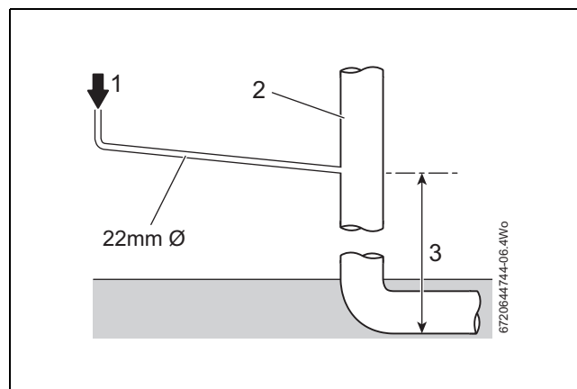
Fig. 17 Eliminación de condensado con orificio de ventilación
