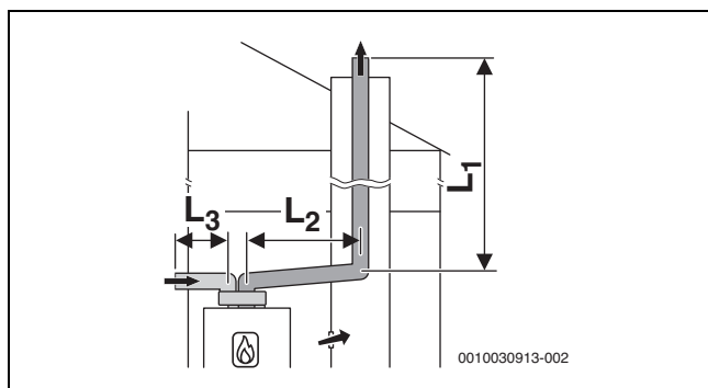
Fig. 9 Conducción rígida de evacuación según C 53 y conducción de la mezcla gas-aire con tubos separados para el acceso de aire y evacuación de gases
