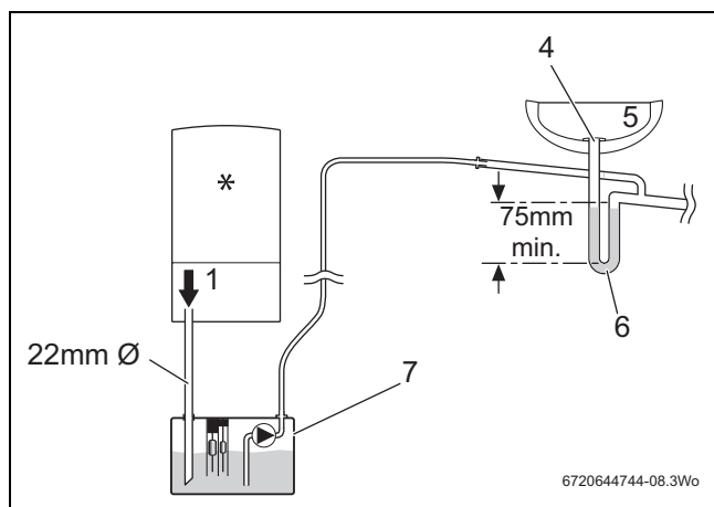
Fig. 19 Evacuación de condensados mediante bomba
