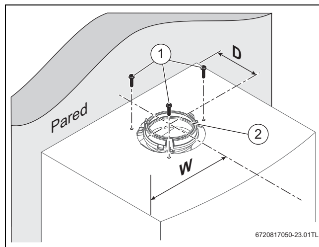
Fig. 48 Centro del adaptador de conducto de evacuación
