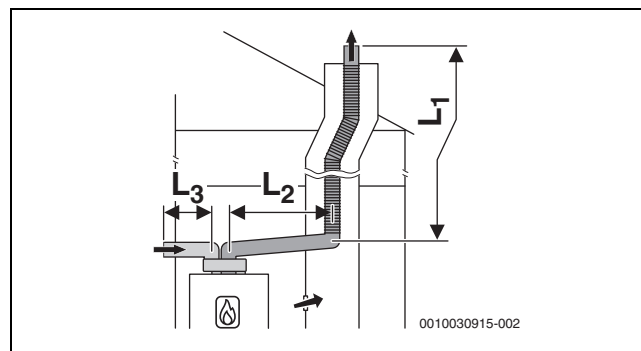
Fig. 10 Conducción flexible de gases de escape según C 53 y en la conducción de la mezcla gas-aire con tubos separados para el acceso de aire y evacuación de gases
