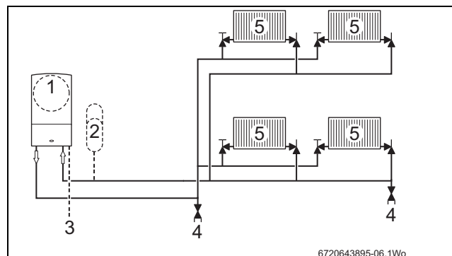
Fig. 15 Sistema cerrado
