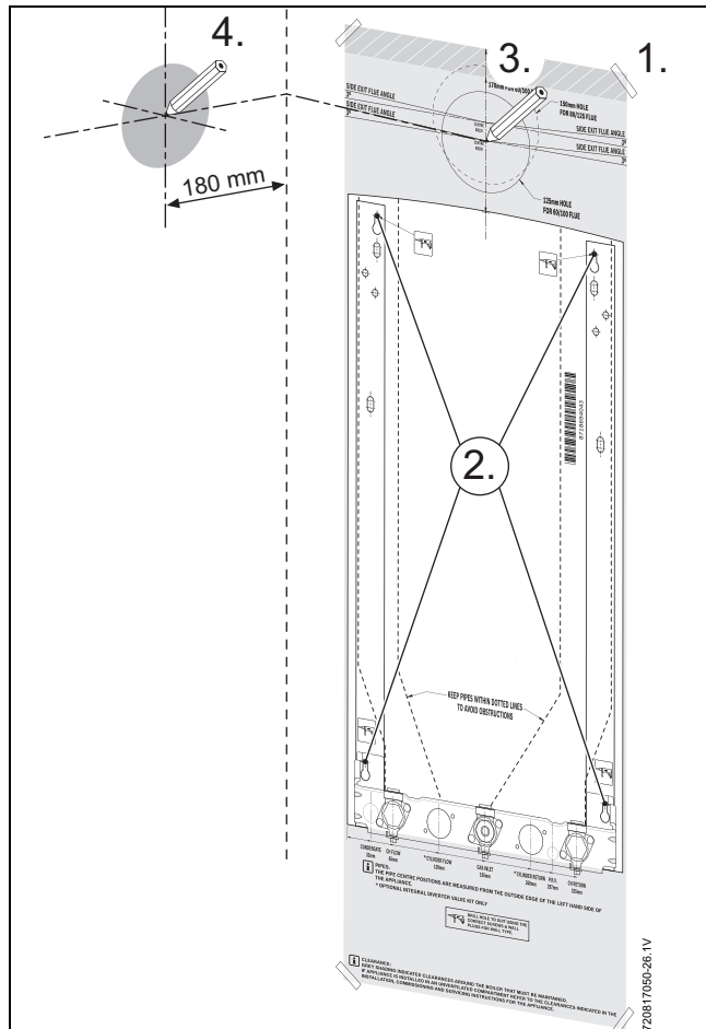
Fig. 34 Marcar la posición del conducto de evacuación
