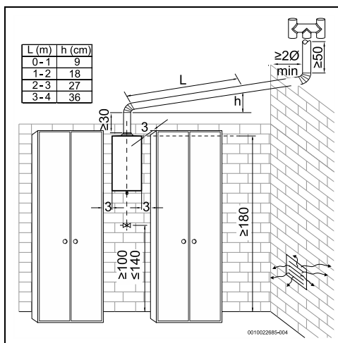
Fig. 10 Distancias mínimas
