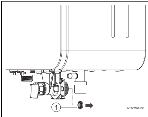
Fig. 30 Filtro de agua
