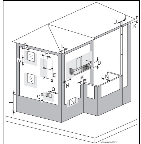
Fig. 20 Distancias mínimas para los conductos de gases de escape
