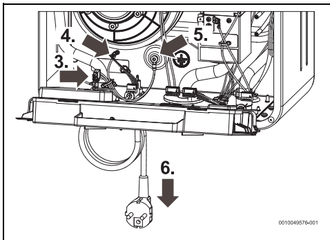
Fig. 27 Conexiones de la línea de conexión a la red
