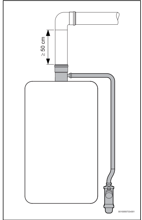
Fig. 17 Sifón de condensados (tubo horizontal)
