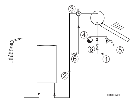
Fig. 18 Instalación solar
