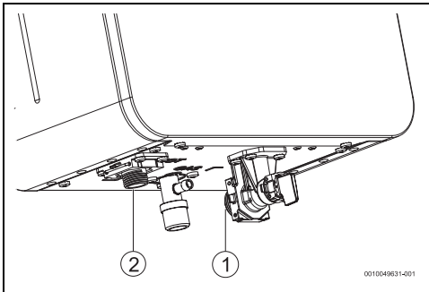
Fig. 22 Conexión de agua
