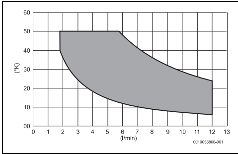
Fig. 32 Modelo de 12 litros
