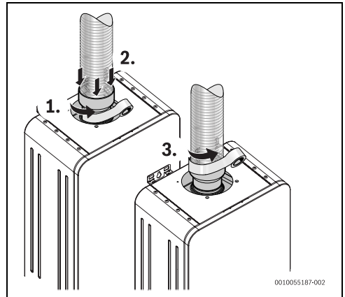
Fig. 24 Instalación tipo B23
