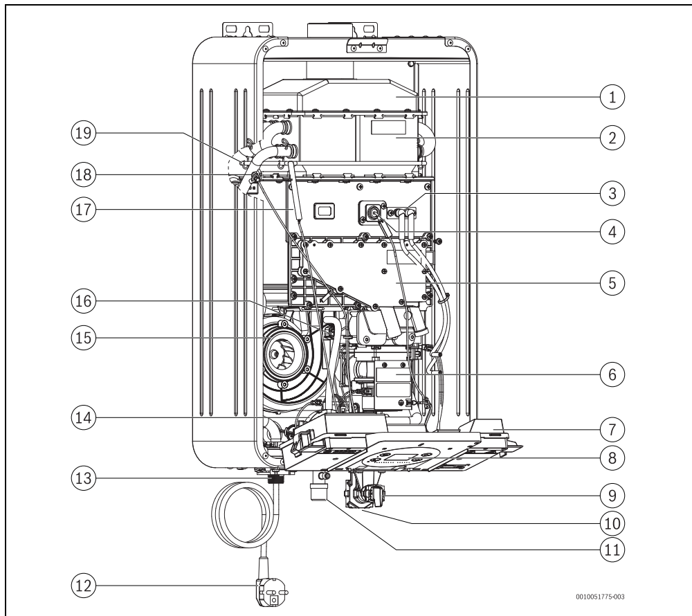
Fig. 3 Diseño del aparato
