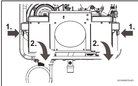
Fig. 26 Inclinación de la caja de control
