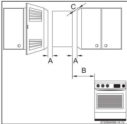
Fig. 19 Distancias mínimas
