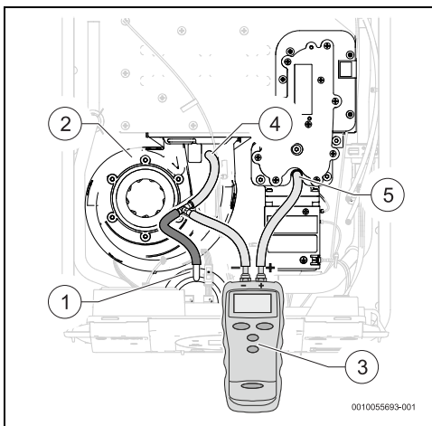
Fig. 28 Conexión del ventilador, sensor de presión y punto de comprobación de la presión de gas
