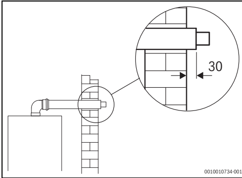
Fig. 25 Dimensiones (en mm)
