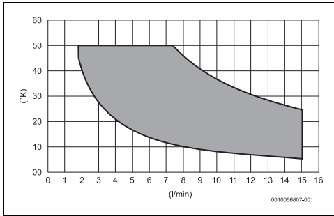
Fig. 33 Modelo de 15 litros
