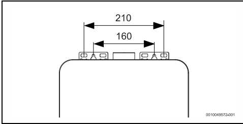
Fig. 21 Puntos de fijación
