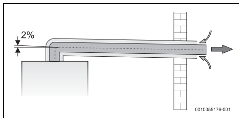
Fig. 23 Instalación tipo C13
