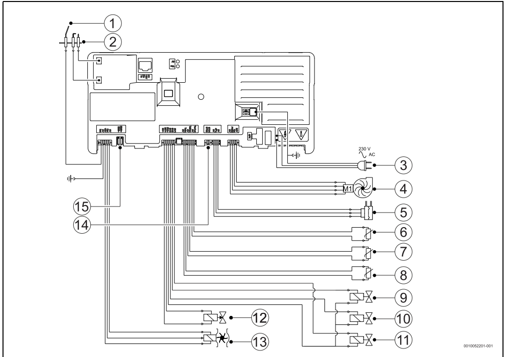
Fig. 31 Esquema de circuitos
