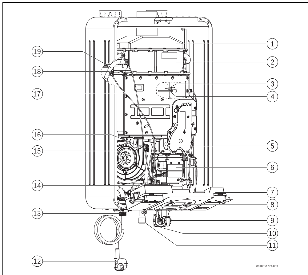
Fig. 2 Diseño del aparato
