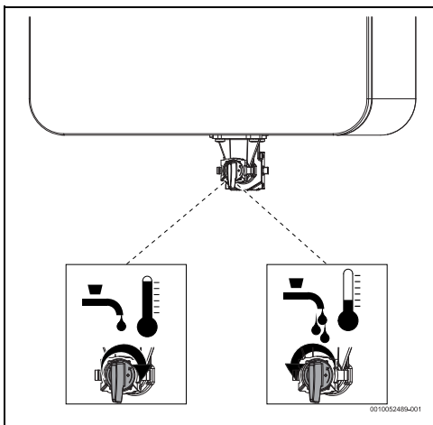
Fig. 9 Control de caudal
