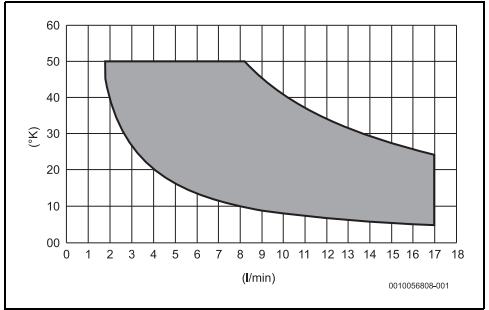
Fig. 34 Modelo de 17 litros
