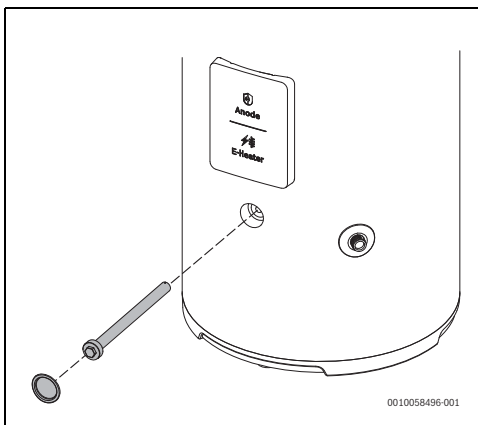
Fig. 25 Rimozione dell'anodo al magnesio
