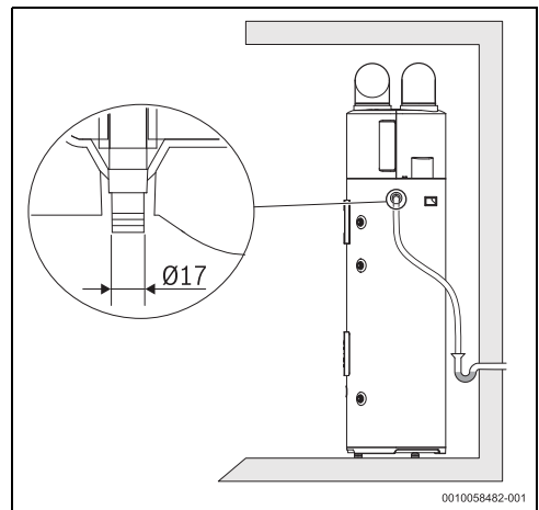
Fig. 15 Conexión de la salida de condensados
