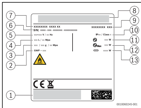
Fig. 2 Descrizione della targhetta identificativa
