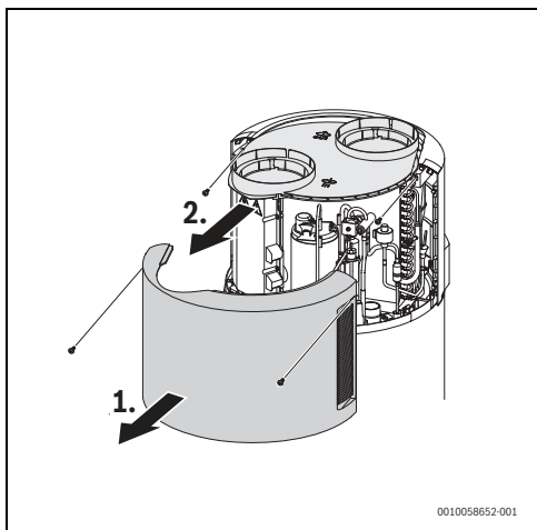
Fig. 24 Rimuovere il coperchio superiore
