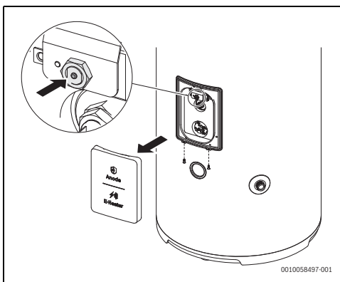
Fig. 26 Reset del termostato di sicurezza
