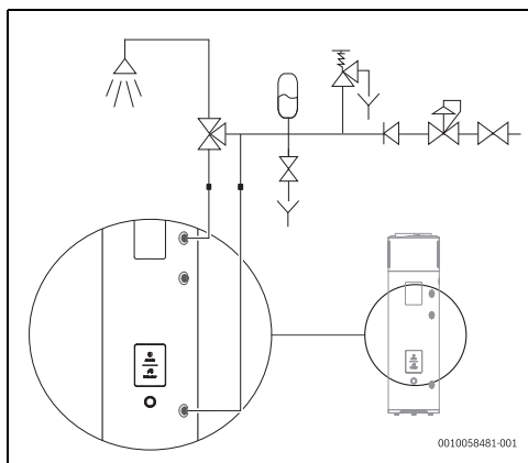
Fig. 14 Conexiones de suministro de agua
