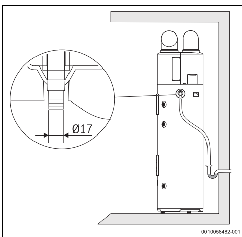
Fig. 15 Collegamento dello scarico condensa
