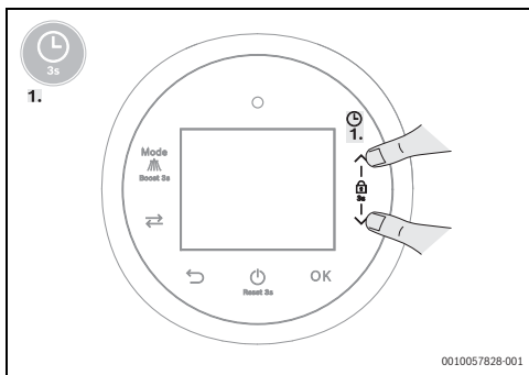
Fig. 20 Bloqueo de los botones
