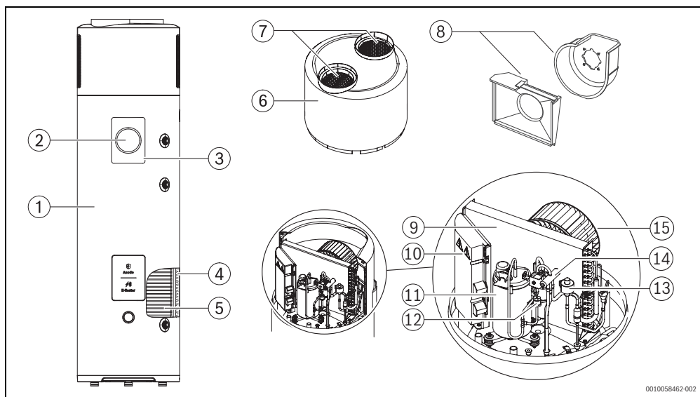
Fig. 4 Vista general del producto
