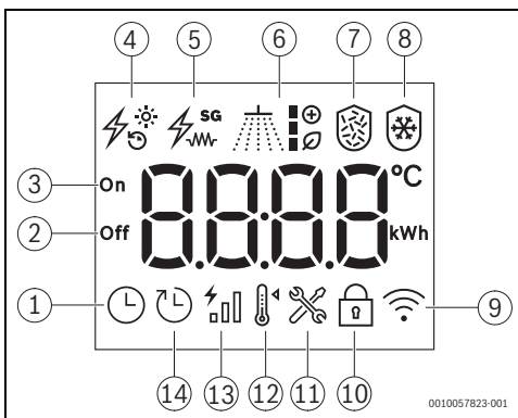
Fig. 19 Interfaccia utente - simboli sul display
