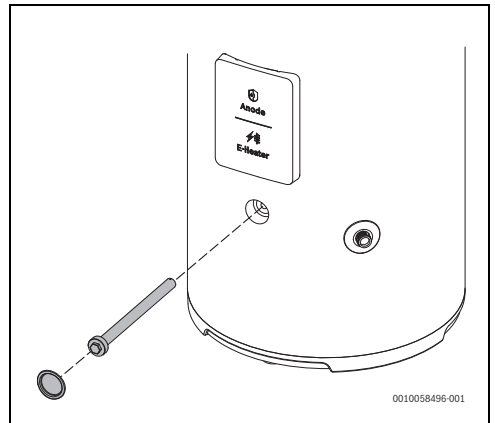
Fig. 25 Desmontaje del ánodo de magnesio
