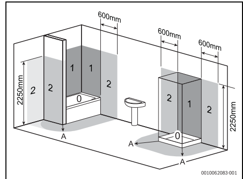
Fig. 8 Distancias mínimas recomendadas (mm)
