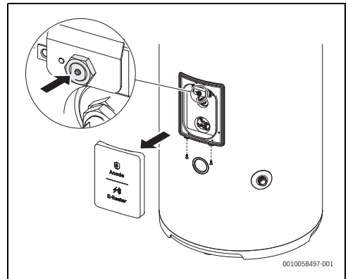
Fig. 26 Reseteo del termostato de seguridad
