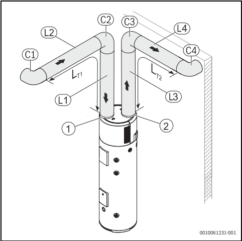
Fig. 12 Ejemplo de instalación
