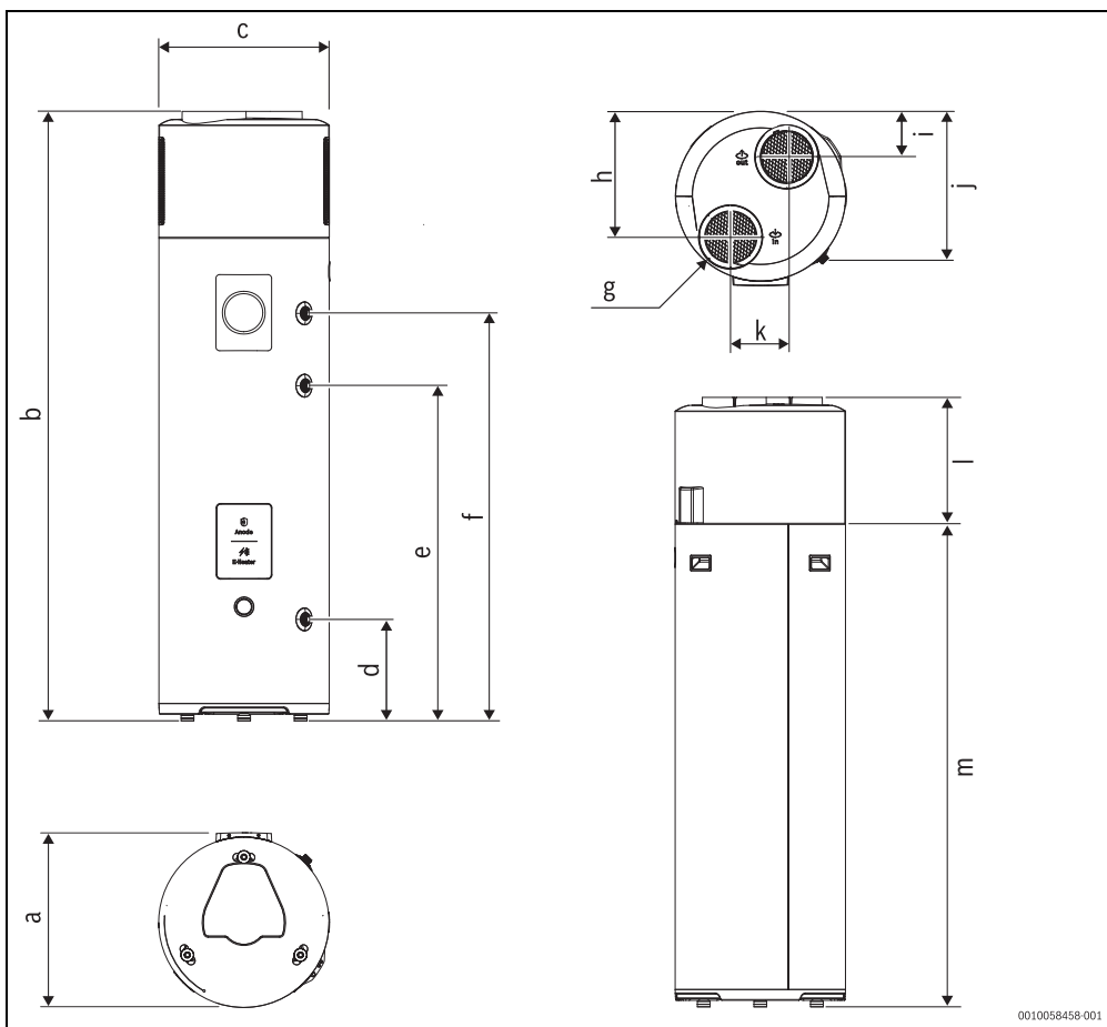
Fig. 3 Dimensiones del aparato
