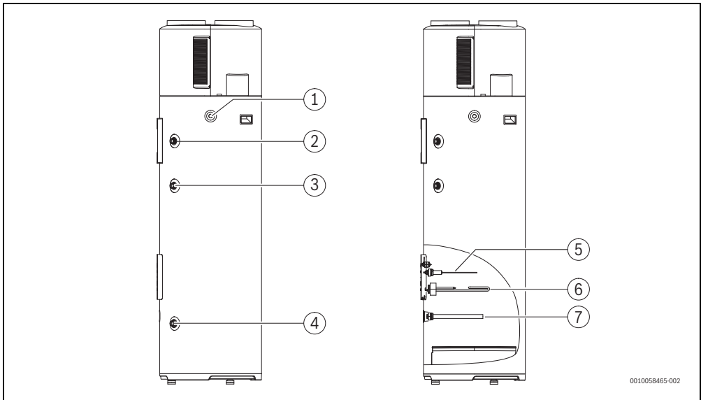
Fig. 5 Vista general del producto
