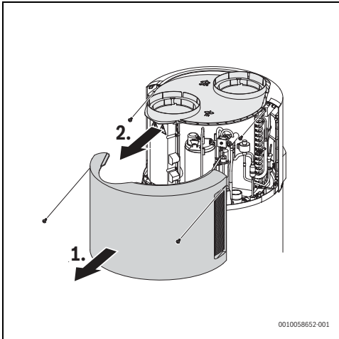
Fig. 24 Retirar la cubierta superior
