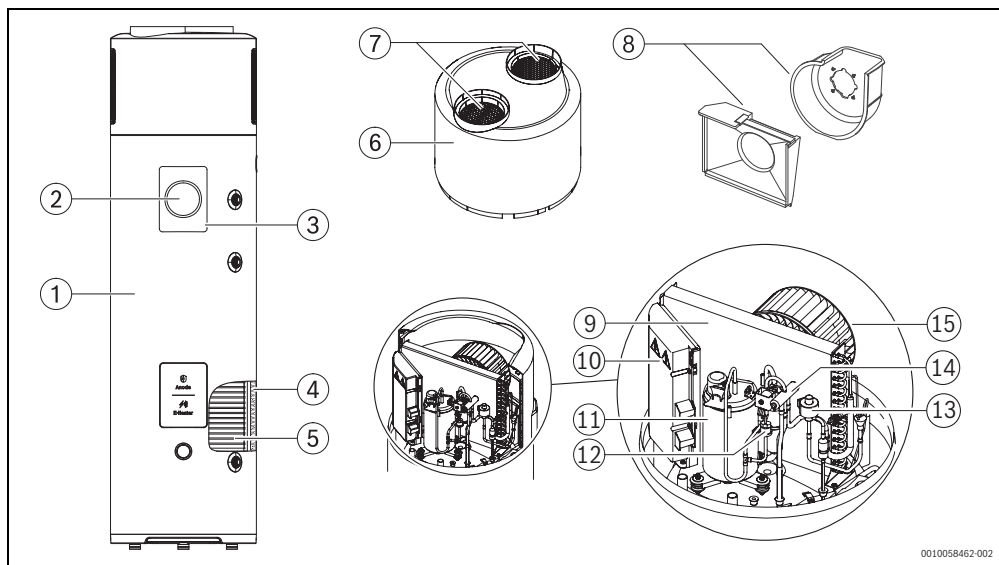
Fig. 4 Panoramica sul prodotto
