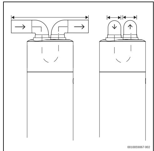
Fig. 11 Segundo canal de ventilación específico
