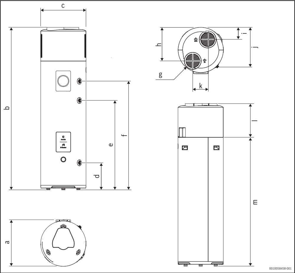
Fig. 3 Dimensões do aparelho
