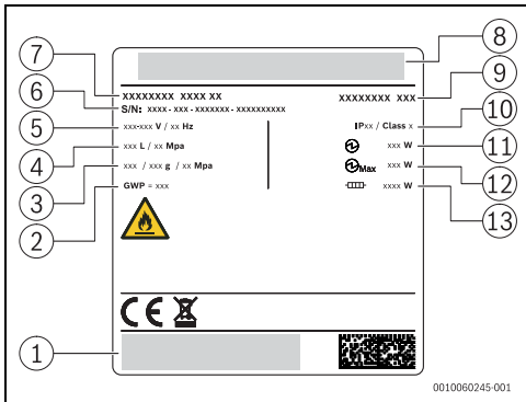
Fig. 2 Descripción de la placa de características
