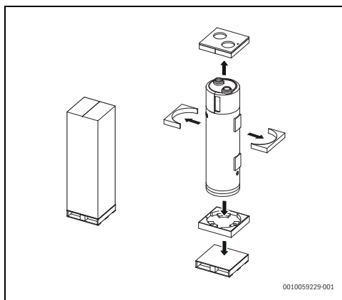
Fig. 7 Disimballaggio dell'apparecchio
