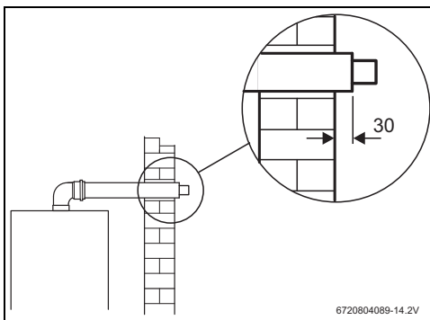
Fig. 16 Dimensiones (en mm)
