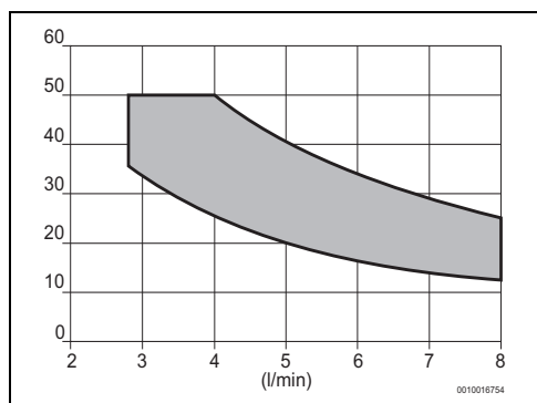
Fig. 23 Modelo 8 litros
