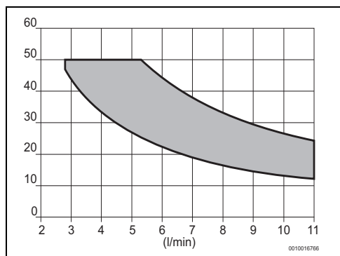
Fig. 24 Modelo 11 litros
