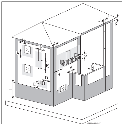
Fig. 13 Distancias mínimas a puntos de salida
