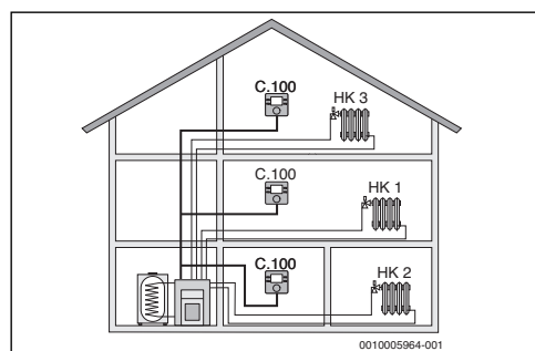
Fig. 3 Ejemplo de una instalación de calefacción con tres circuitos de calefacción con un C 100 como regulador (vivienda multifamiliar)
