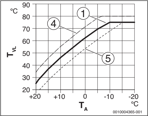
Fig. 15 Ajuste de la curva de calefacción para radiadores Desplazamiento paralelo mediante temperatura ambiente deseada
