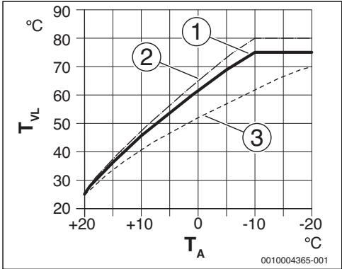
Fig. 14 Ajuste de la curva de calefacción para radiadores Incremento mediante temperatura de referencia T_{AL} y temperatura exterior mínima T_{A,min}
