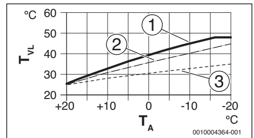
Fig. 11 Ajuste de la curva de calefacción para la calefacción por suelo radiante
