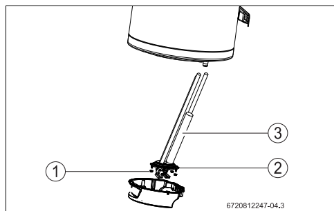
Fig. 13 Acceso a la zona interior e identificación de las partes
