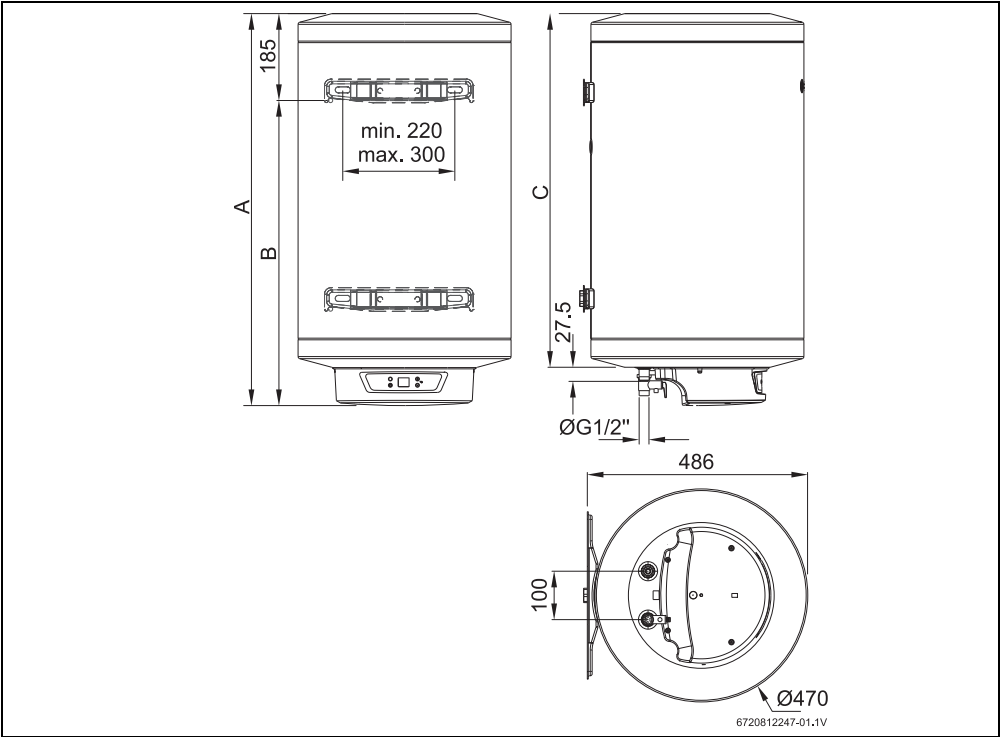
Fig. 2 Dimensiones en mm (Montaje mural, instalación vertical)
