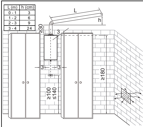
Fig. 10 Separaciones mínimas (en cm)
