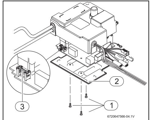
Fig. 14 Caja de comando
