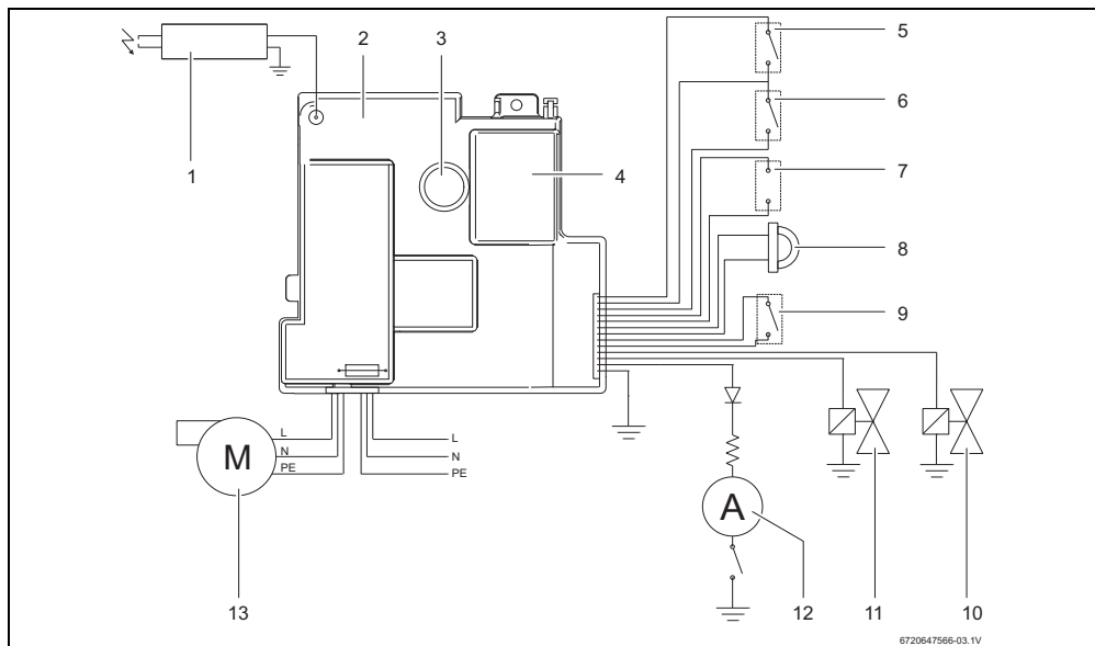
Fig. 2 Esquema eléctrico
