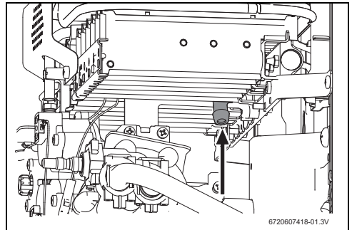
Fig. 12 Punto de medición de presión
