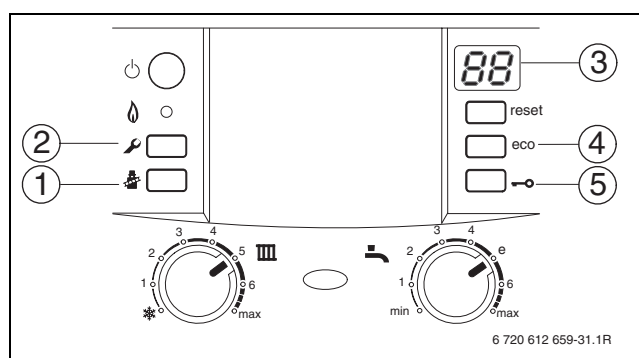
Fig. 29 Relación de los elementos de manejo
