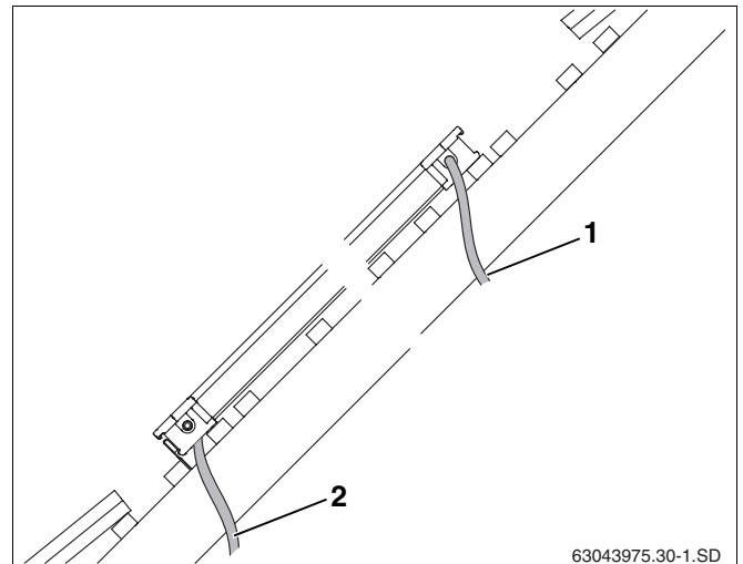
Fig. 34 Introducir las tuberías de conexión por debajo del tejado
