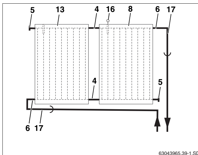
Fig. 63 Conexión hidráulica
