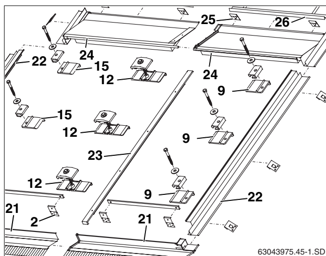
Fig. 64 Fijación y recubrimiento de dos colectores
