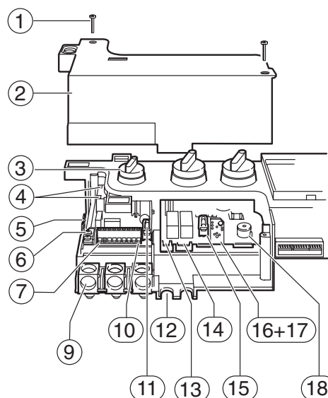
Fig. 10 Conexiones en la Eurotronic
