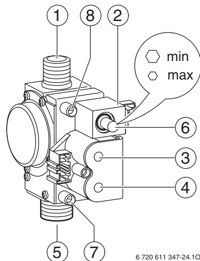
Fig. 23 Cuerpo de gas
