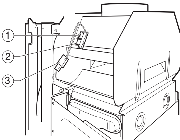
Fig. 39 Sonda de control de los gases de evacuación
