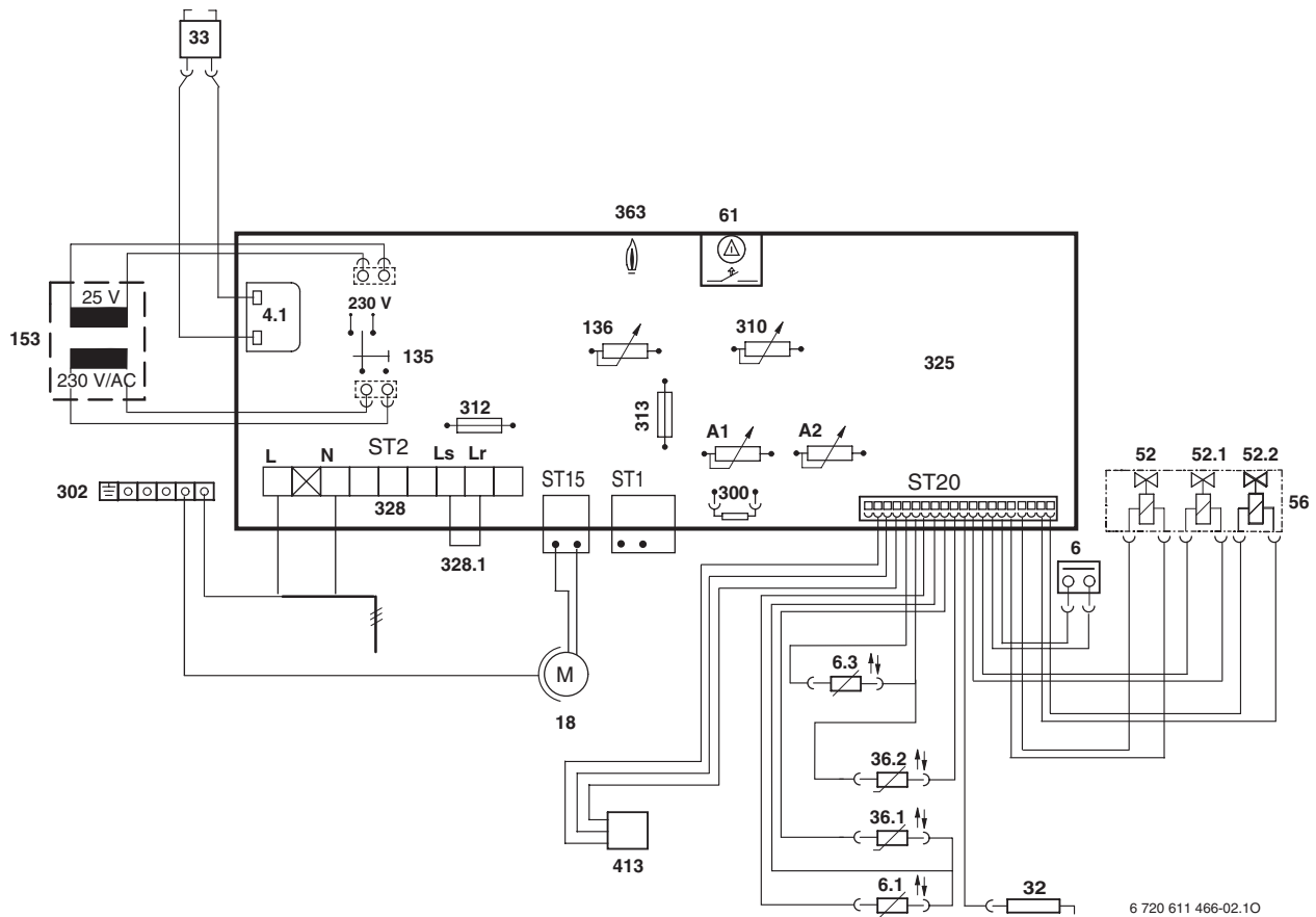
Fig. 2 Cableado eléctrico
