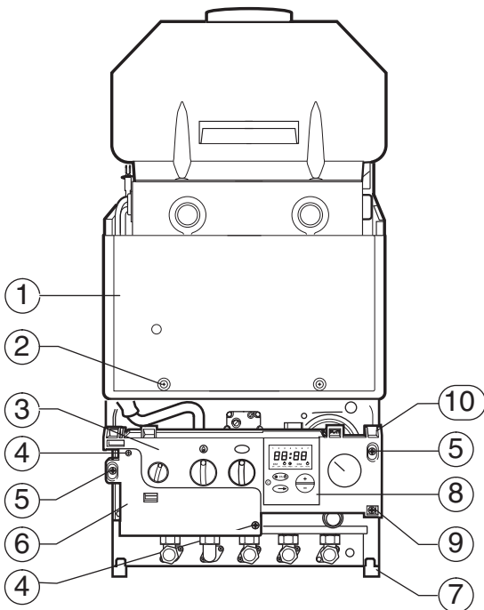
Fig. 36 Sujeción de la cubierta termoaislante y de la Eurotronic
