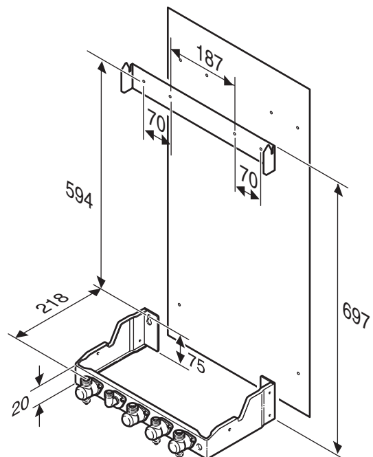
Fig. 5 Sujeción a la pared
