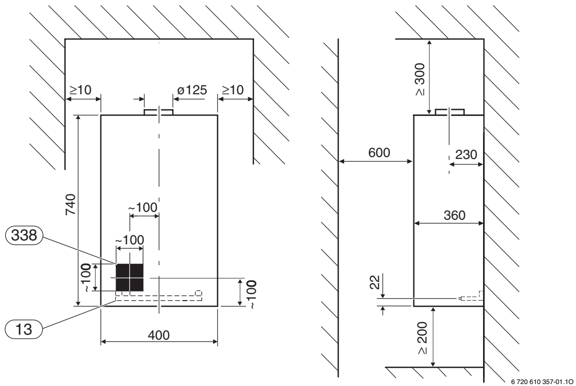
Fig. 1 Vista frontal y lateral
