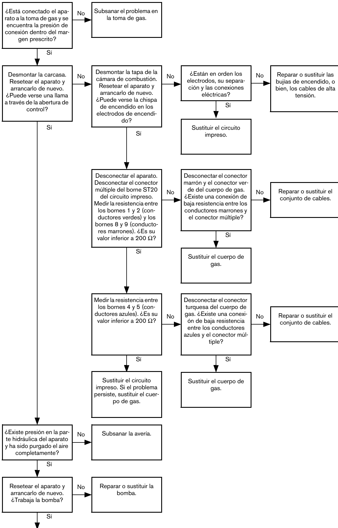
Fig. 47 Prueba D (Capítulo 1 de 2)
