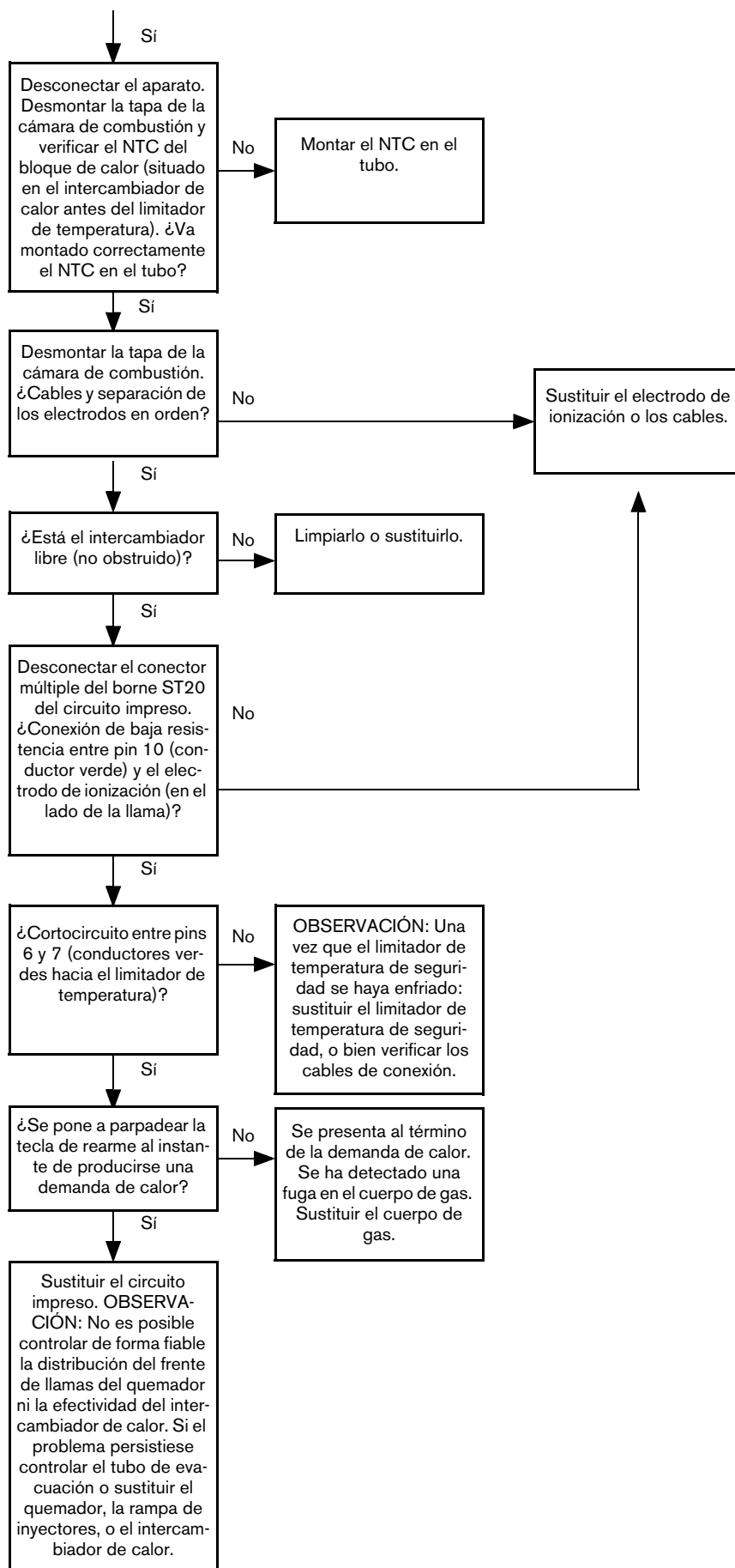
Fig. 48 Prueba D (Capítulo 2 de 2)
