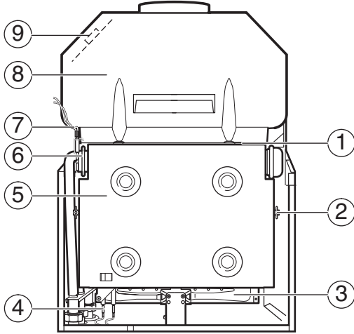
Fig. 38 Componentes situados detrás de la cubierta termoaislante
