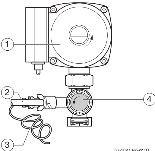
Fig. 21 Válvula de seguridad
