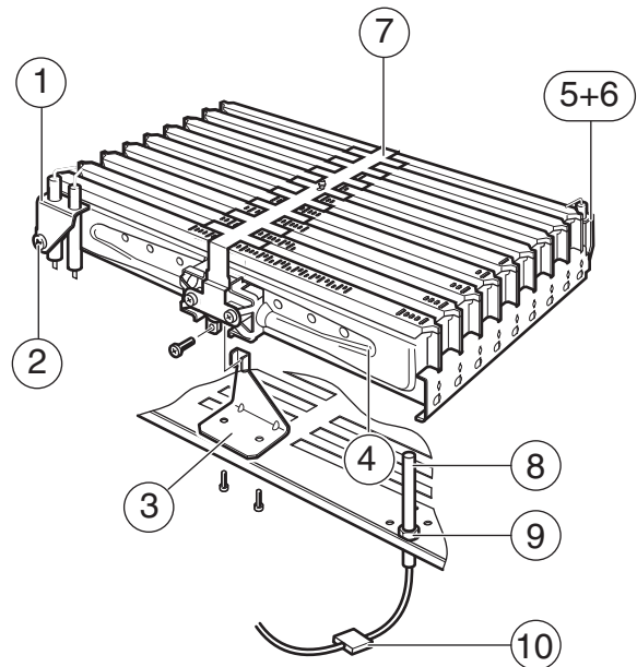
Fig. 40 Unidad de quemador
