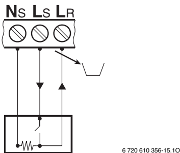
Fig. 14 Conexión del termostato ambiente 230 V (retirar el puente entre L_S y L_R )
