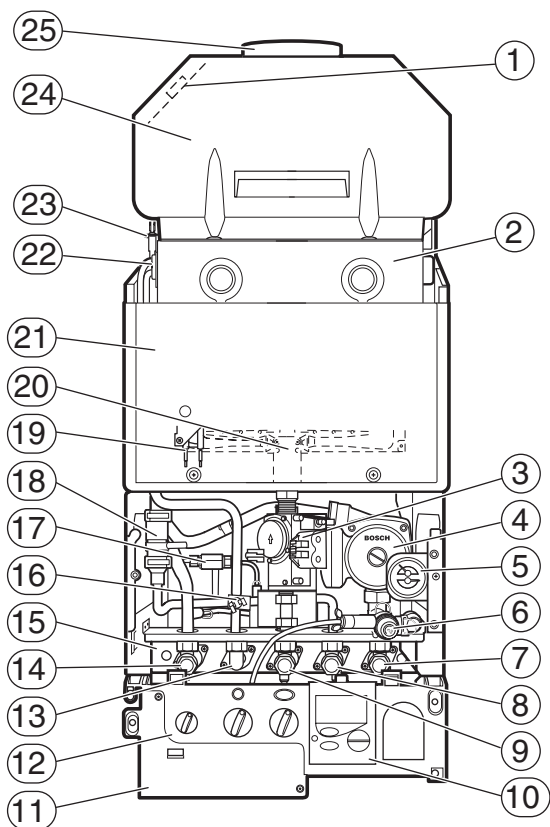
Fig. 18 Componentes del aparato; Eurotronic en posición de servicio
