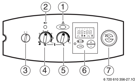
Fig. 26 Panel de mandos
