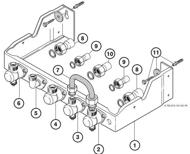
Fig. 7 Plantilla de montaje
