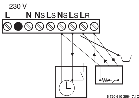
Fig. 16 Conexión del termostato ambiente 230 V y del reloj programador 230 V (retirar el puente entre L_S y L_R )
