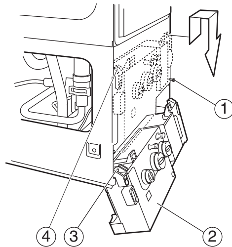
Fig. 37 Colocación de la Eurotronic en posición de servicio
