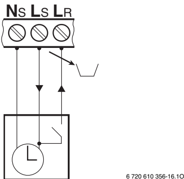
Fig. 15 Conexión del reloj programador 230 V (retirar el puente entre L_S y L_R )
