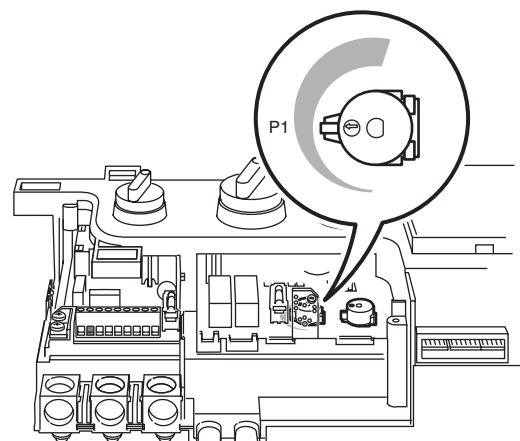
Fig. 25 Ajuste de la potencia máxima de calefacción
