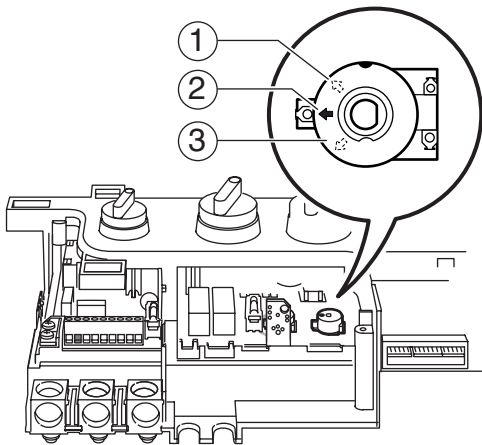
Fig. 24 Selección del modo de operación
