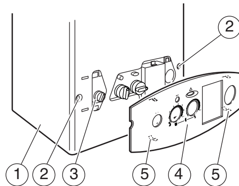
Fig. 35 Carcasa – panel de mandos
