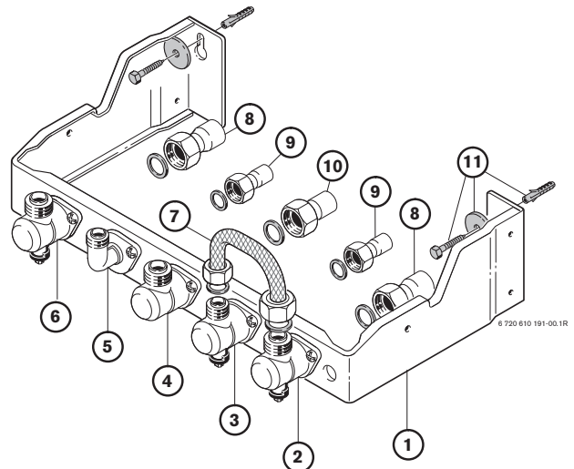
Fig. 11 Plantilla de montaje
