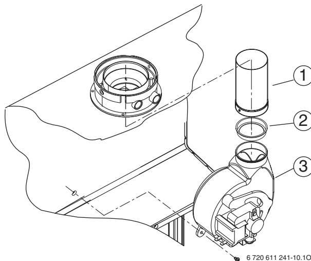
Fig. 25 Desmontaje del ventilador
