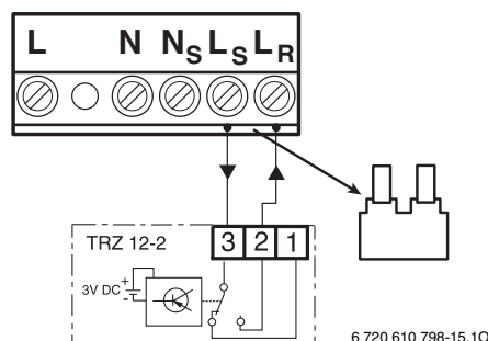
Fig. 31 Conexión con un termostato ON/OFF TRZ .. (230 V AC, quitar el puente L_S e L_R )
