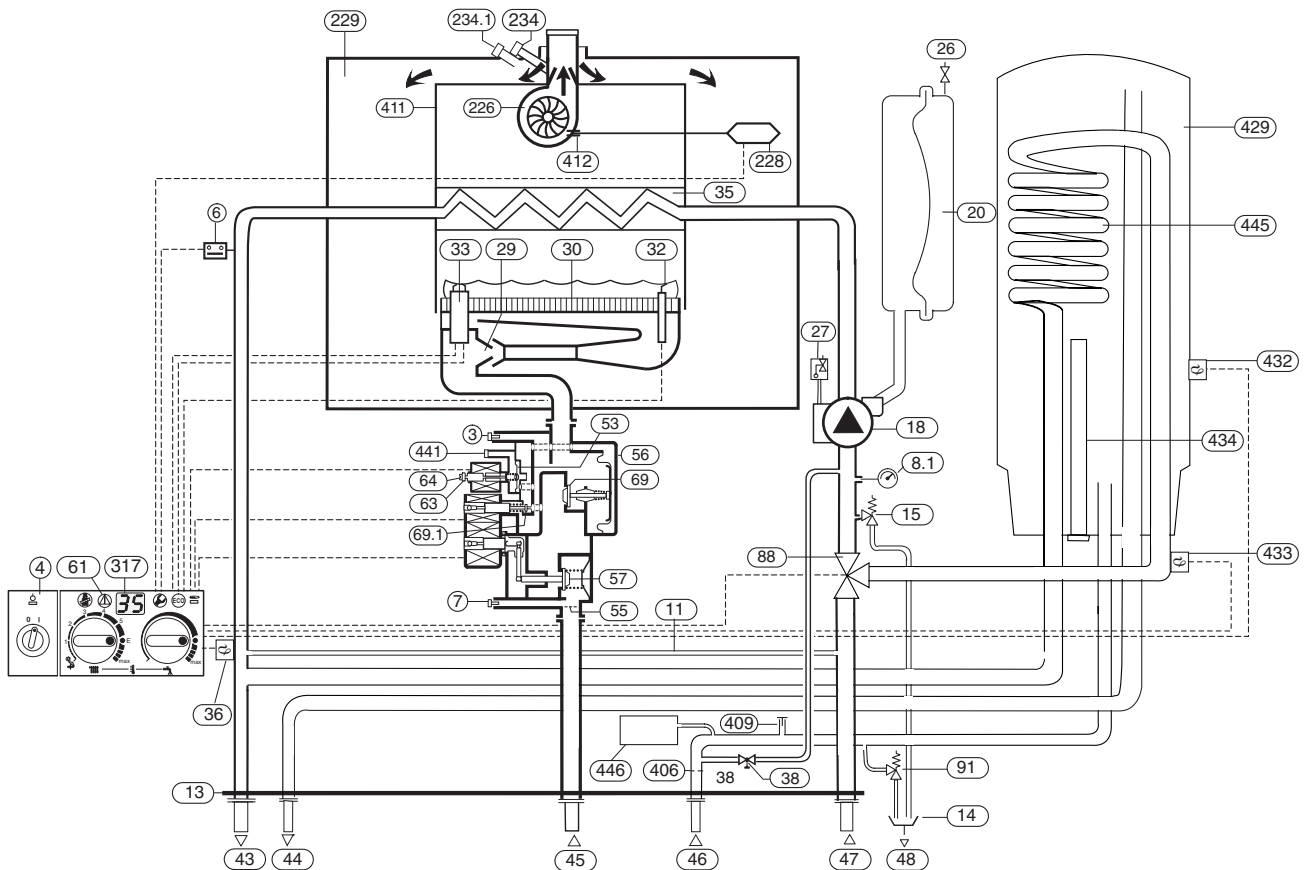
Fig. 3 Esquema de funcionamiento del ZWSE 28-4 MFA
