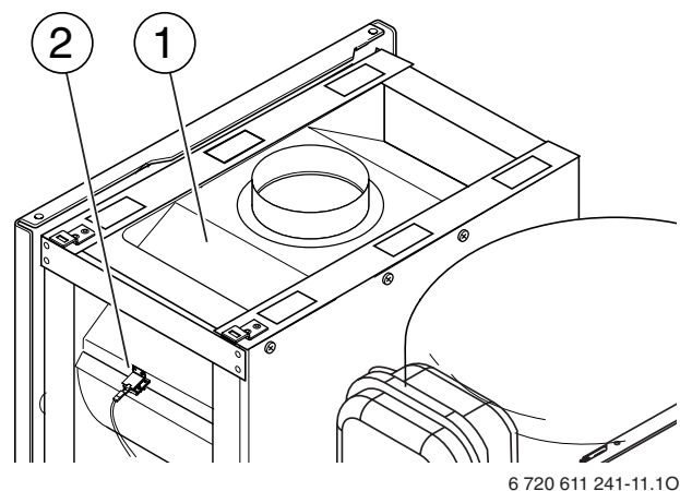
Fig. 72 Sonda de los productos de la combustión en el cortatiro
