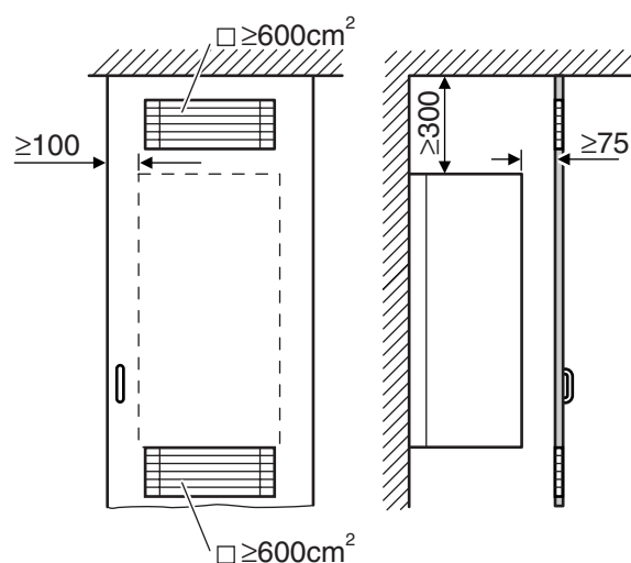
Fig. 7 Aberturas de refrigeración para el caso de instalación en un armario
