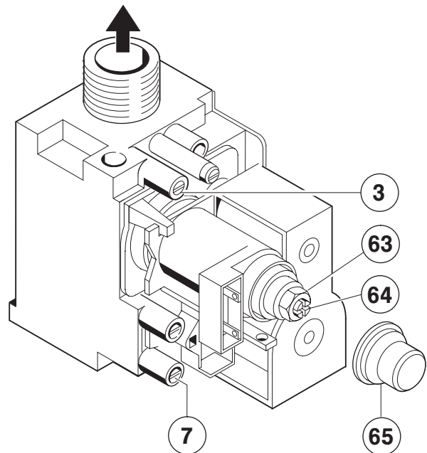
Fig. 58 Cuerpo de gas
