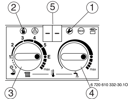
Fig. 40 Relación de los elementos de mando
