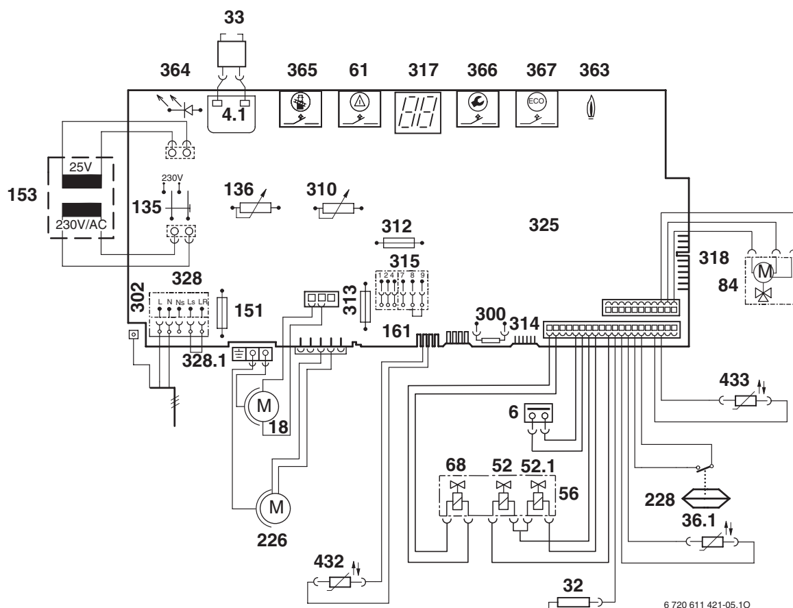
Fig. 5 Cableado eléctrico del ZWSE 28-4 MFA
