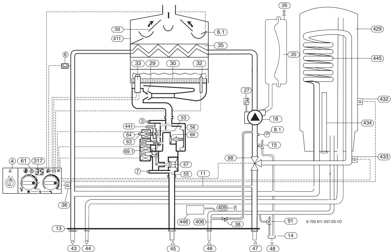
Fig. 4 Esquema de funcionamiento del ZWSE 23-4 MFK
