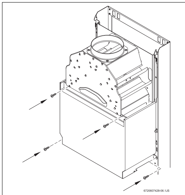
Fig. 23 Tampa protectora
