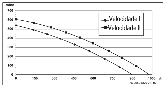
Fig. 4 Curva característica da bomba
