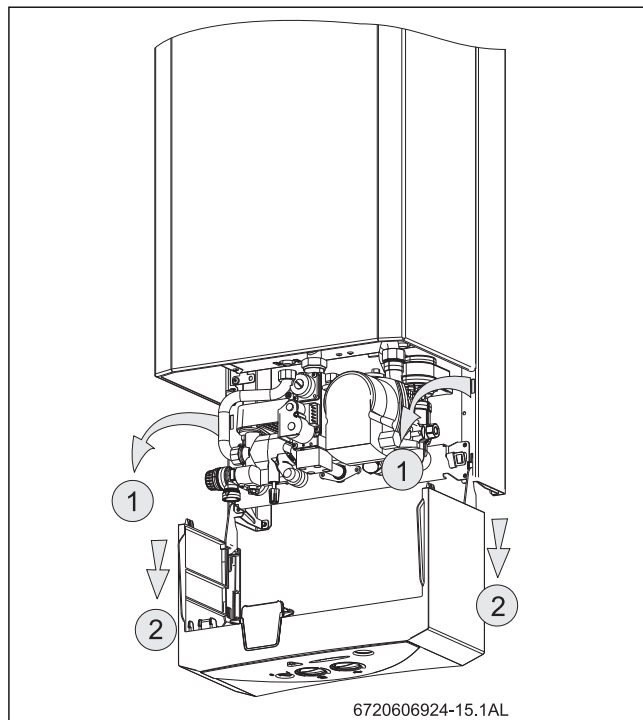
Fig. 25 Posição de serviço para acessibilidade à hidráulica e à electrónica
