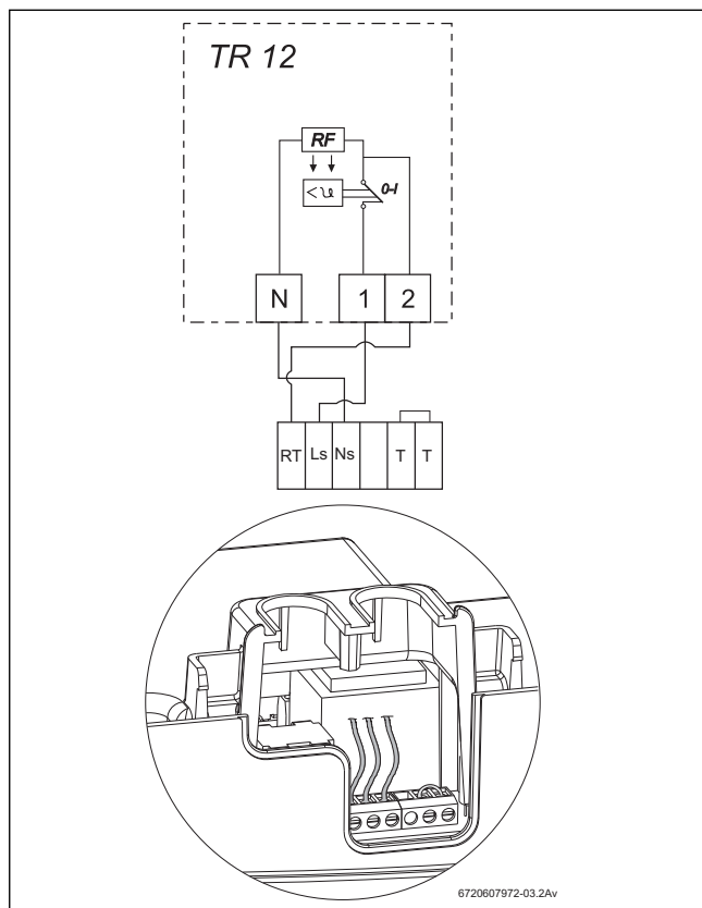
Fig. 41 TR 12
