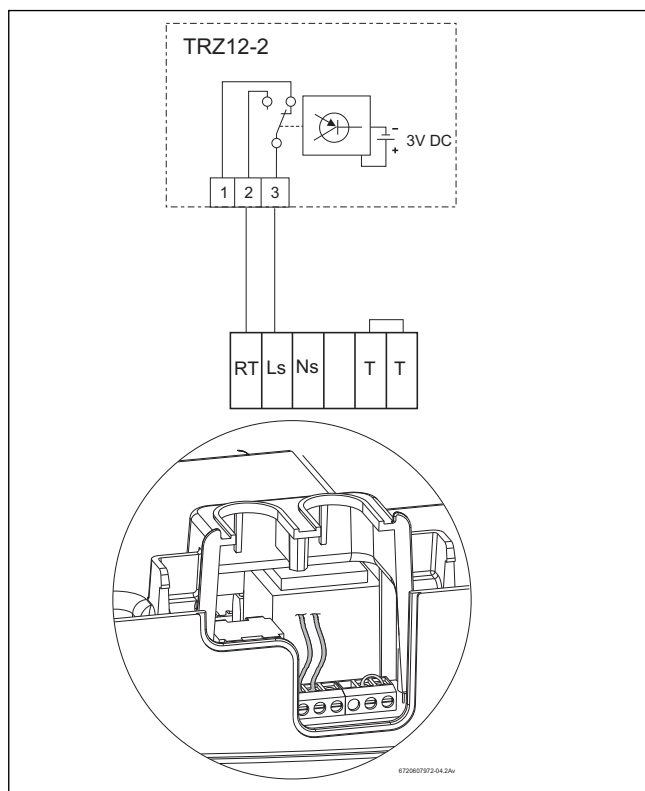
Fig. 14 TRZ 12-2
