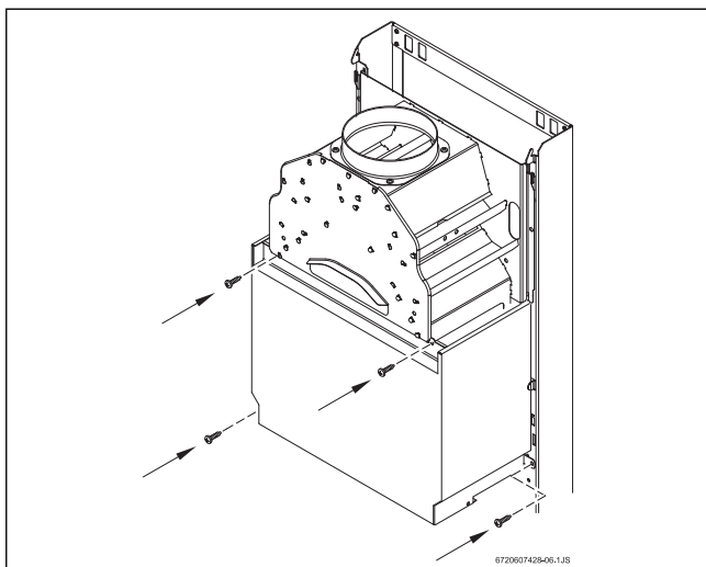
Fig. 51 Tapa protectora
