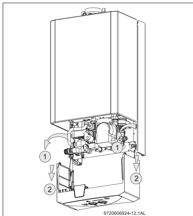
Fig. 36 Posición de servicio para tener acceso al sistema hidráulico y electrónico
