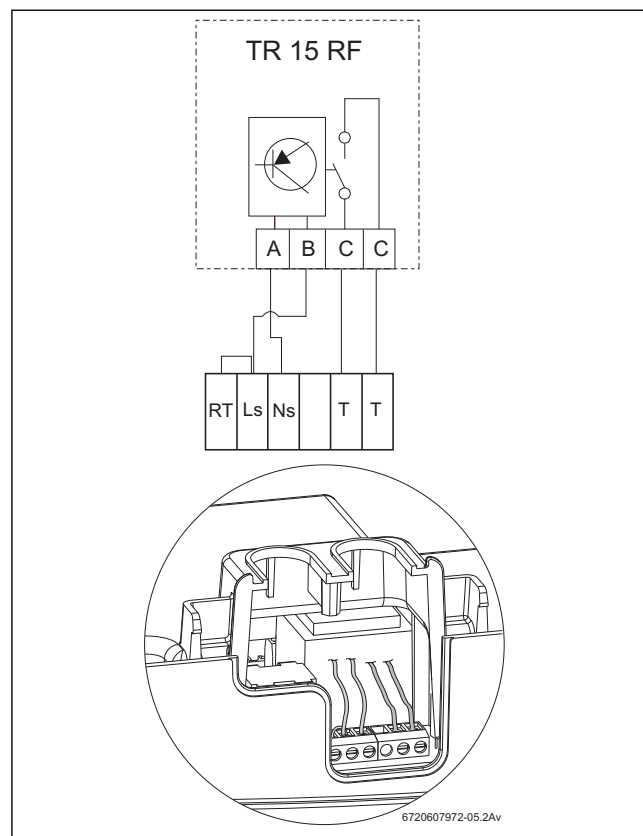
Fig. 43 TR 15RF
