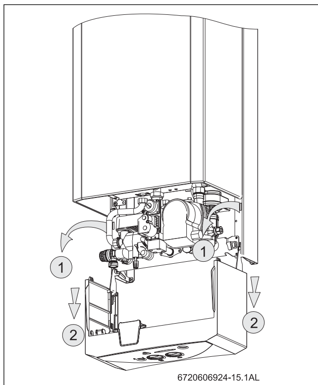
Fig. 53 Posición de servicio para acceso a la parte hidráulica y electrónica
