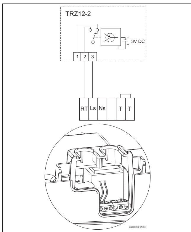
Fig. 42 TRZ 12 - 2
