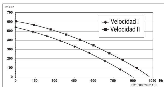
Fig. 33 Curva característica de la bomba
