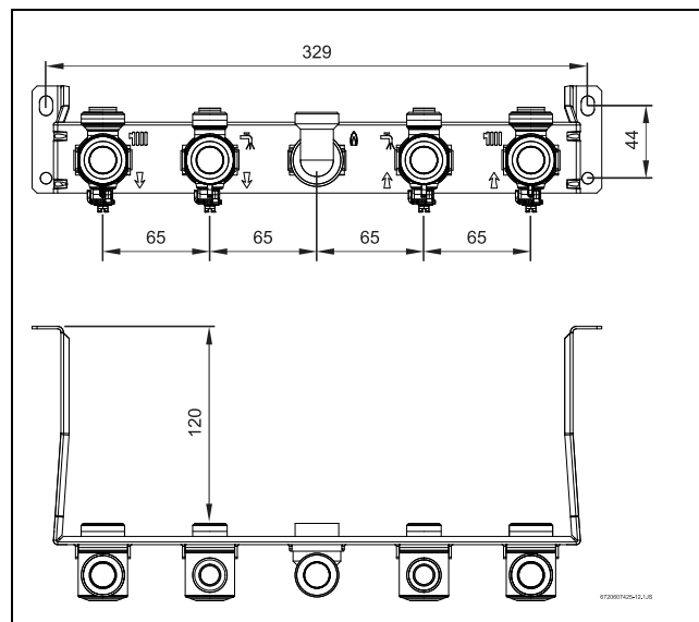
Fig. 8 Conexiones hidráulicas
