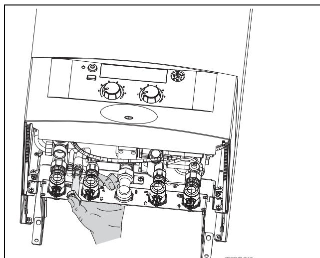
Fig. 15 Llave de llenado
