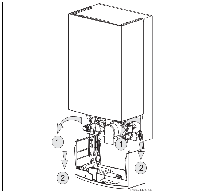
Fig. 31 Posición de servicio para acceso a la parte hidráulica y electrónica
