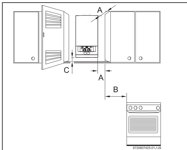
Fig. 6 Separaciones mínimas
